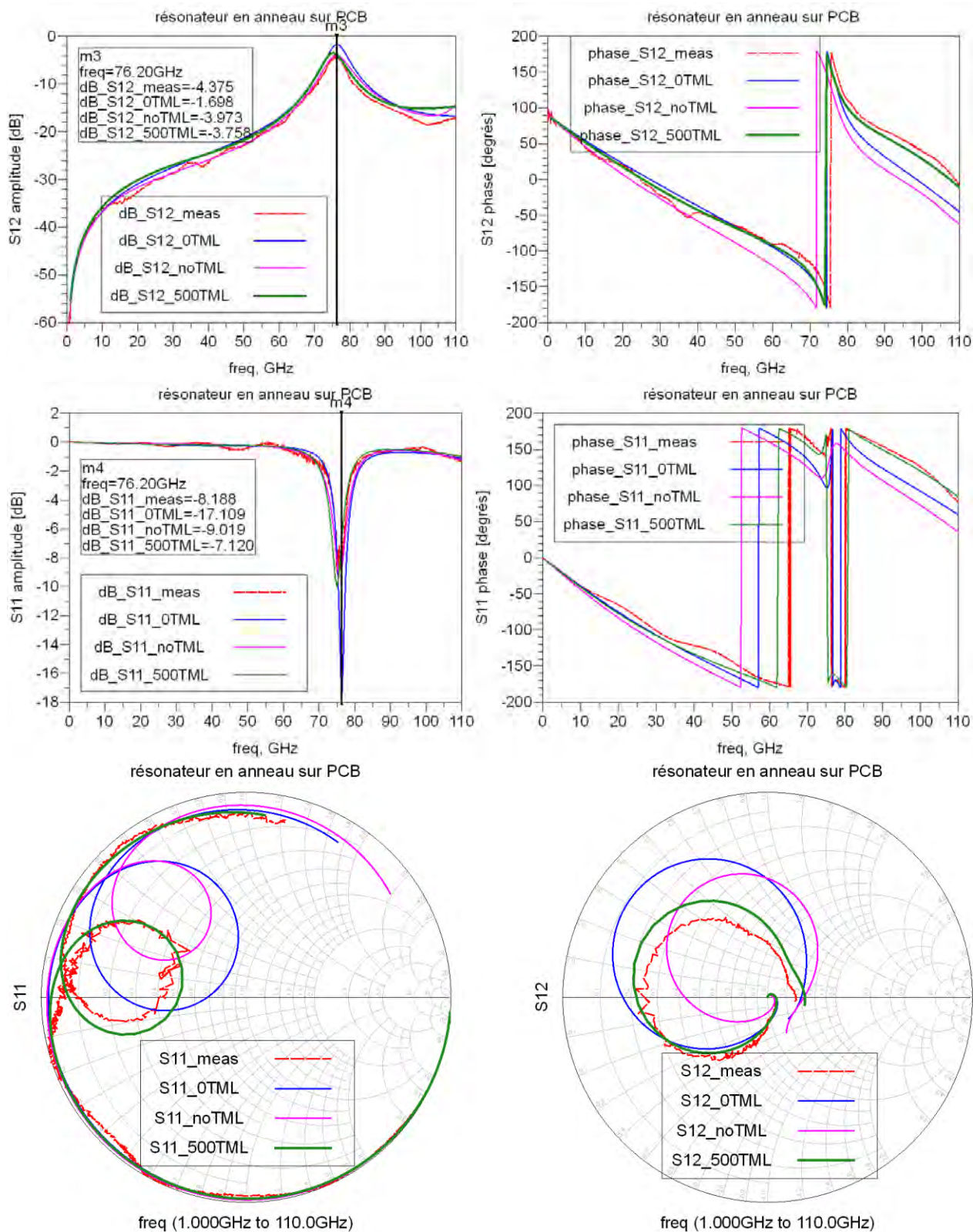
Figure 45 : comparaison des résultats de simulations et de mesures du résonateur en anneau pour différentes définitions de ports
