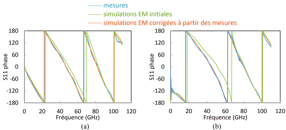
Figure 55 : comparaison des simulations et des mesures des structures « circuit ouvert (O) » (a) et « charge 50 Ω (L) » (b) en boîtier avant et après correction
