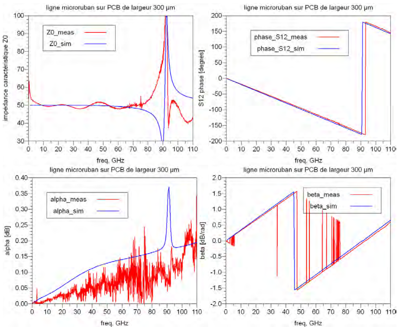
Figure 46 : comparaison des simulations et mesures d'une ligne microruban 50 Ω sur PCB
