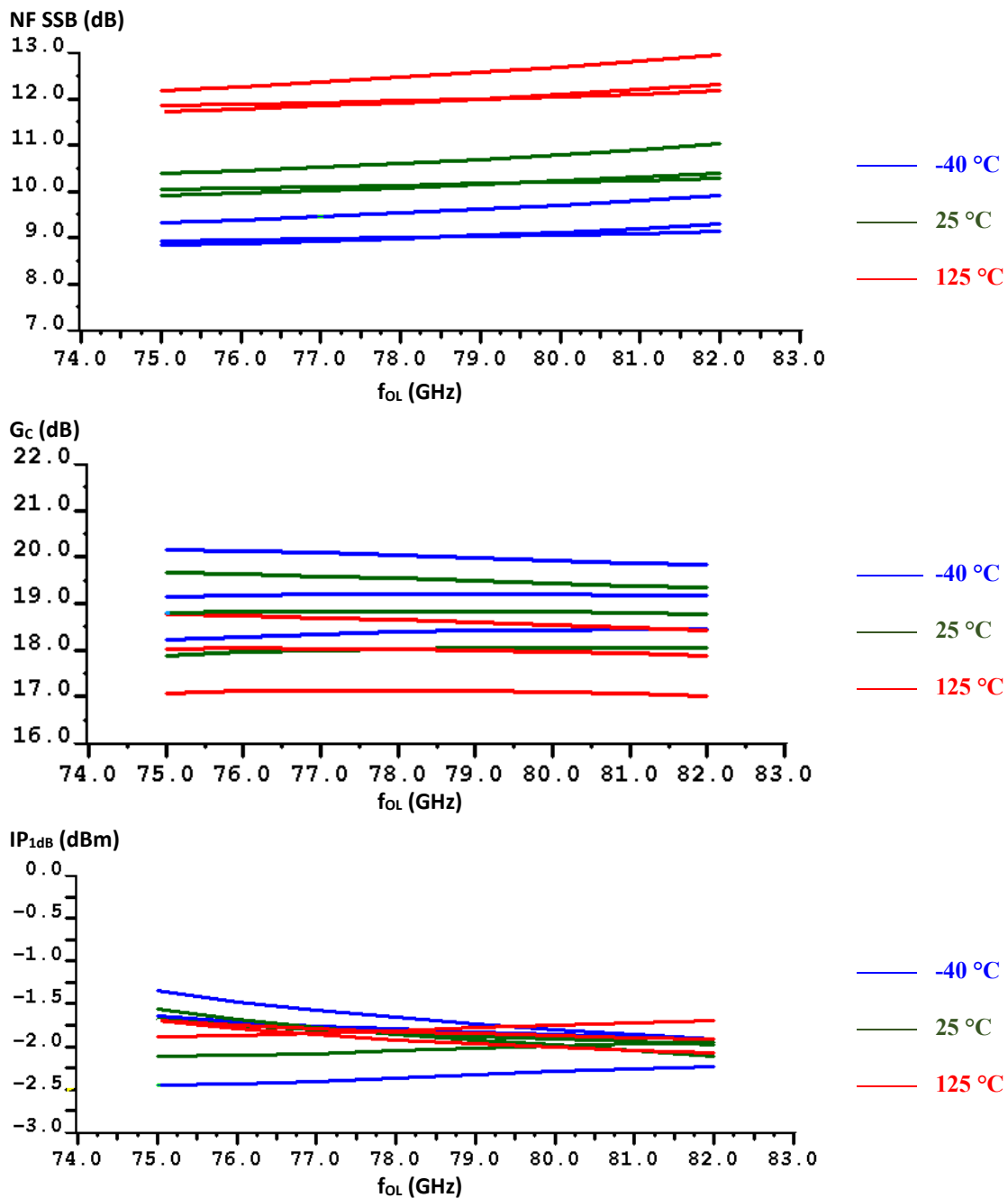
Figure 100 : résultats de simulations du facteur de bruit (NF SSB), du gain de conversion ( G_c ) et de la compression en entrée ( IP_{1dB} ) du mélangeur en boîtier en fonction de la fréquence OL ( f_{OL} ) pour f_{F1} = 1 MHz et pour différentes températures
