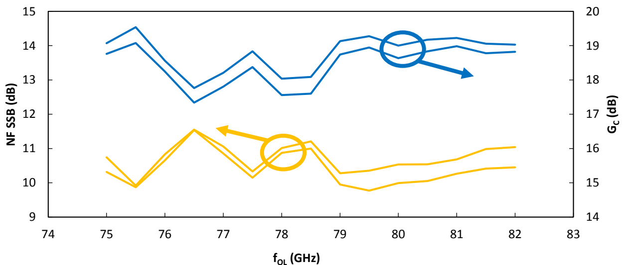
Figure 102 : facteur de bruit SSB (NF SSB) et gain de conversion ( G_c ) du mélangeur en boîtier en fonction de la fréquence OL ( f_{OL} ) pour f_{FI} = 1 MHz et pour 2 pièces
