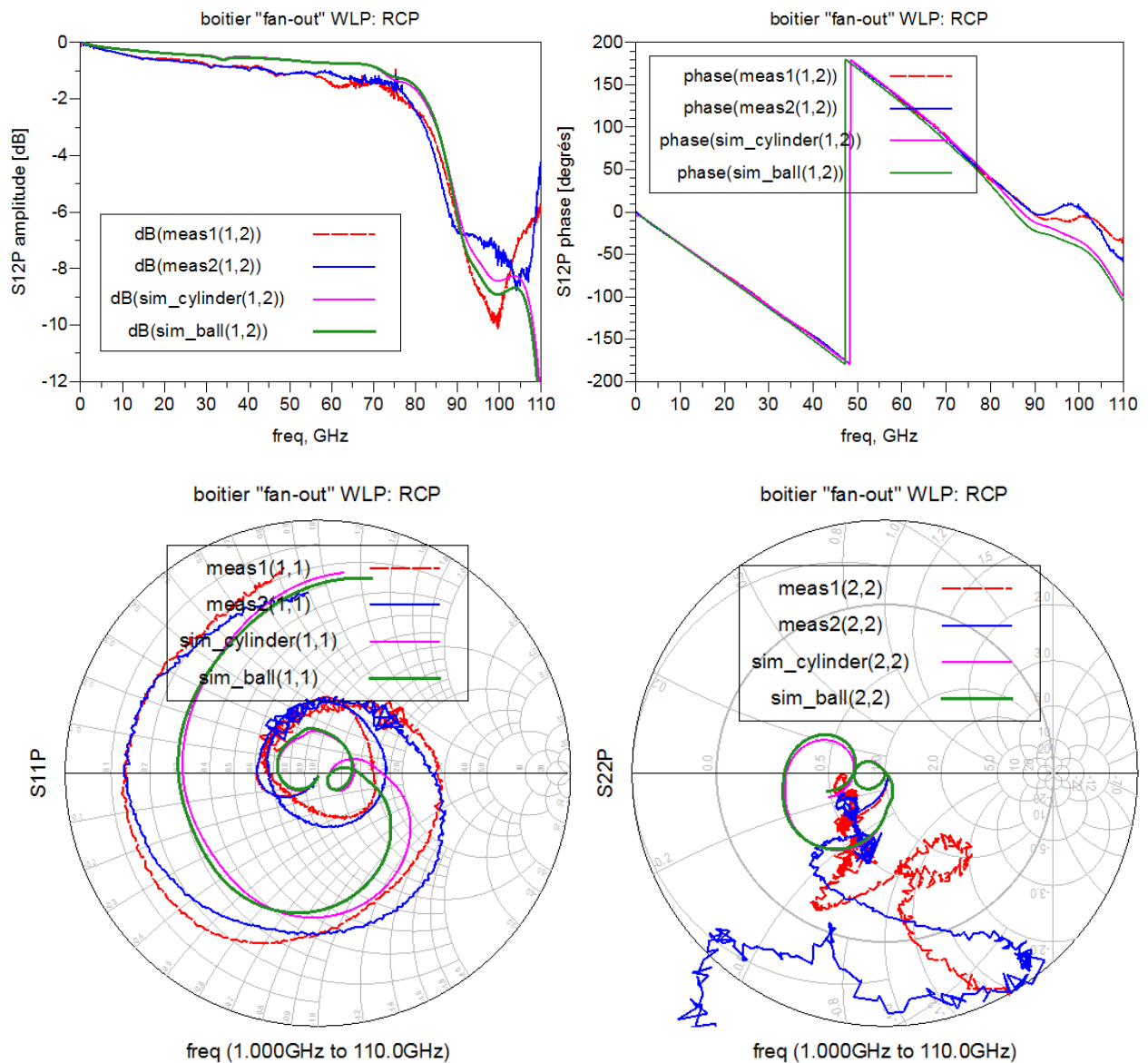
Figure 54 : comparaison des simulations et des extractions par la mesure des paramètres S du boîtier RCP
