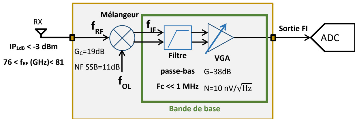
Figure 75 : diagramme de blocs d'une chaîne e réception à base d'un mélangeur actif
