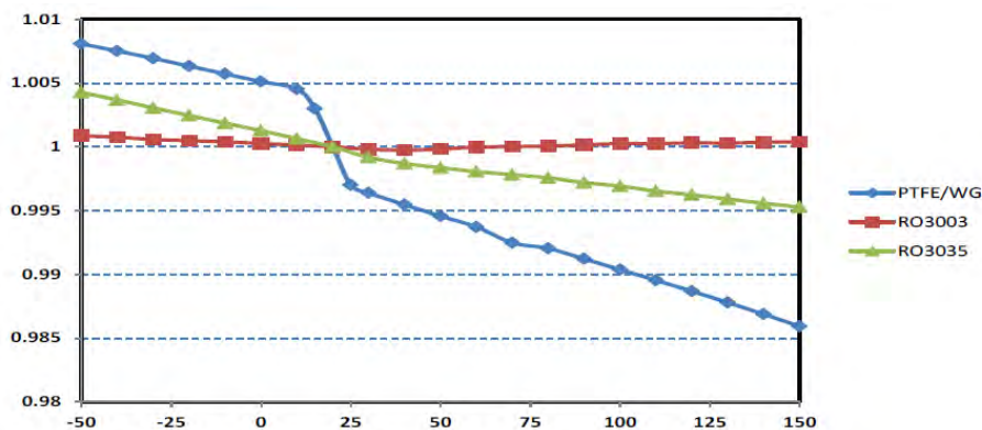
Figure 14 : variation de la constante diélectrique de quelques substrats Rogers en fonction de la température [1.20]
