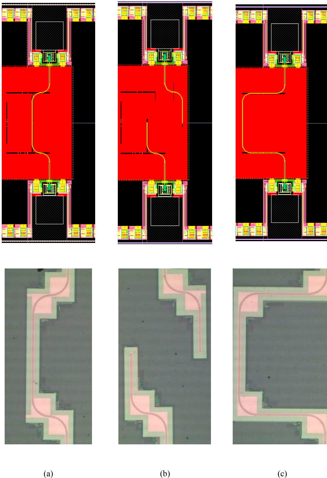
Figure 70 : les dessins de masque et photos des 3 standards TRL sur puce nue : Thru (a), Reflect (b) et Line (c)
