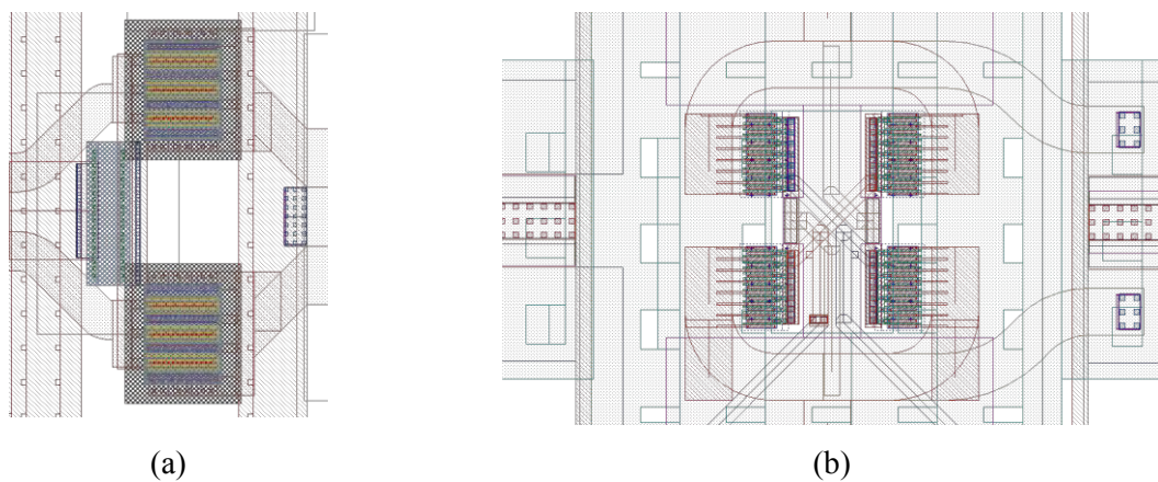
Figure 87 : dessins de masque des transistors MOS du mélangeur passif (a) et des transistors bipolaires de l'amplificateur RF (b)
