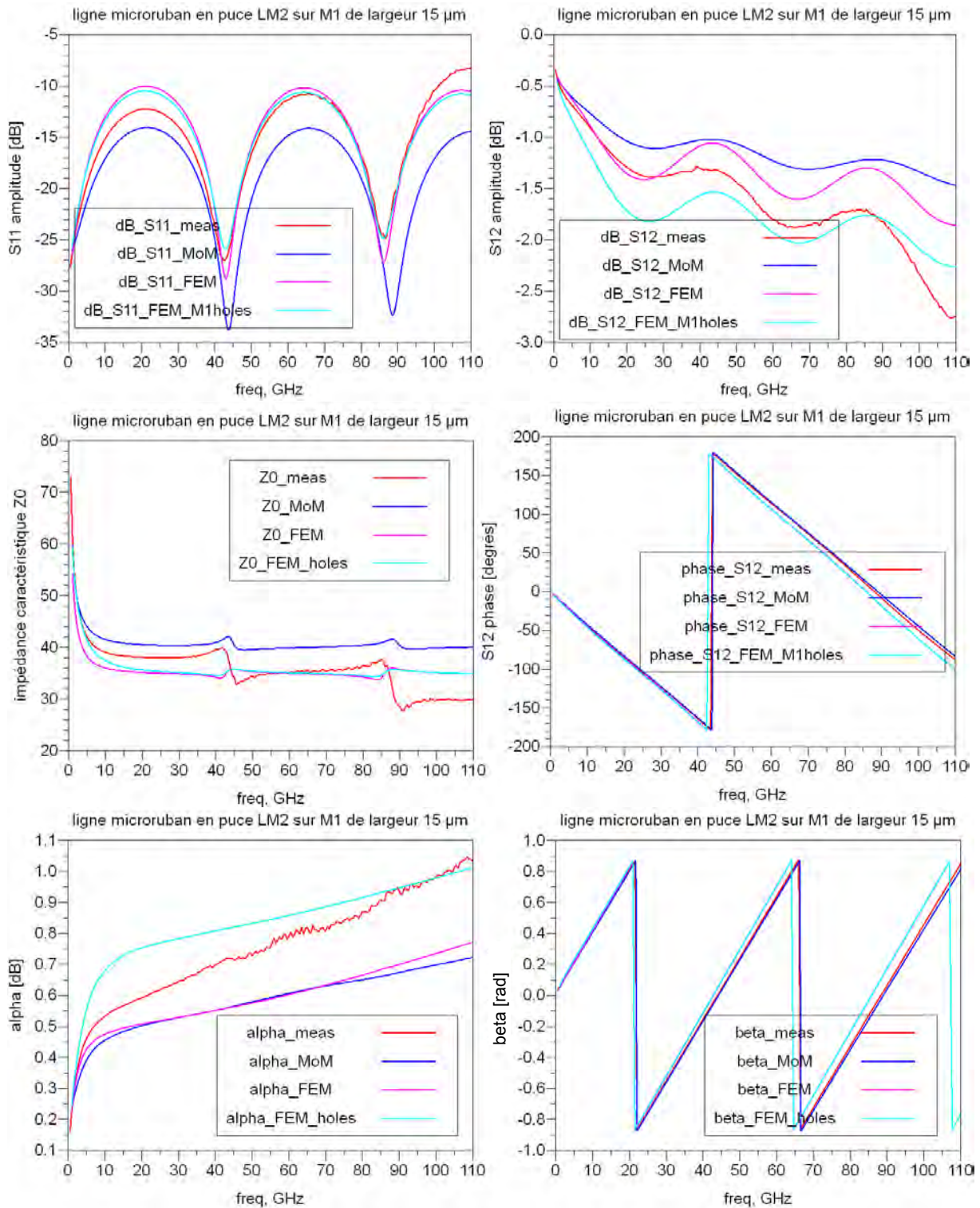
Figure 34 : résultats de simulation et de mesures d'une ligne d'une largeur de 15 μm
