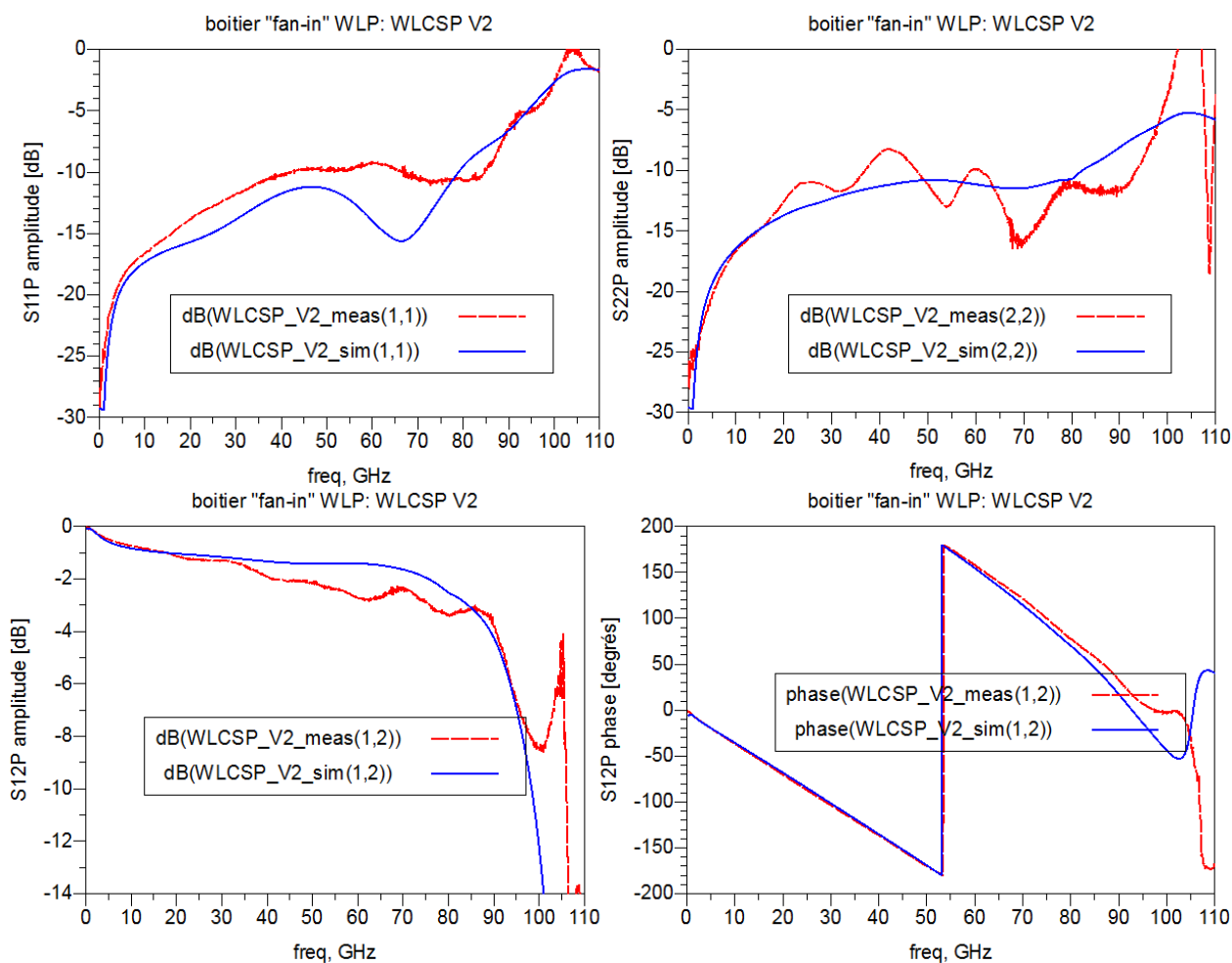
Figure 66 : simulations et mesures de la nouvelle interface boitier conçue WLCSP V2
