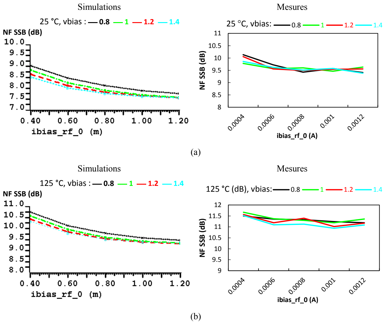
Figure 96 : comparaison des simulations et des mesures du facteur de bruit SSB (NF SSB) du mélangeur actif en puce nue en fonction du courant de polarisation de référence ( i_{bias\_rf} ) et de la tension de polarisation ( v_{bias} ) pour f_{OL} = 76.5 GHz et f_{RF} = 1 MHz aux températures de 25 °C (a) et 125 °C (b)
