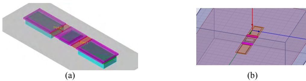
Figure 24 : comparaison entre les vues 3D ADS (a) ET 3D HFSS (b) utilisant les mêmes types de port
