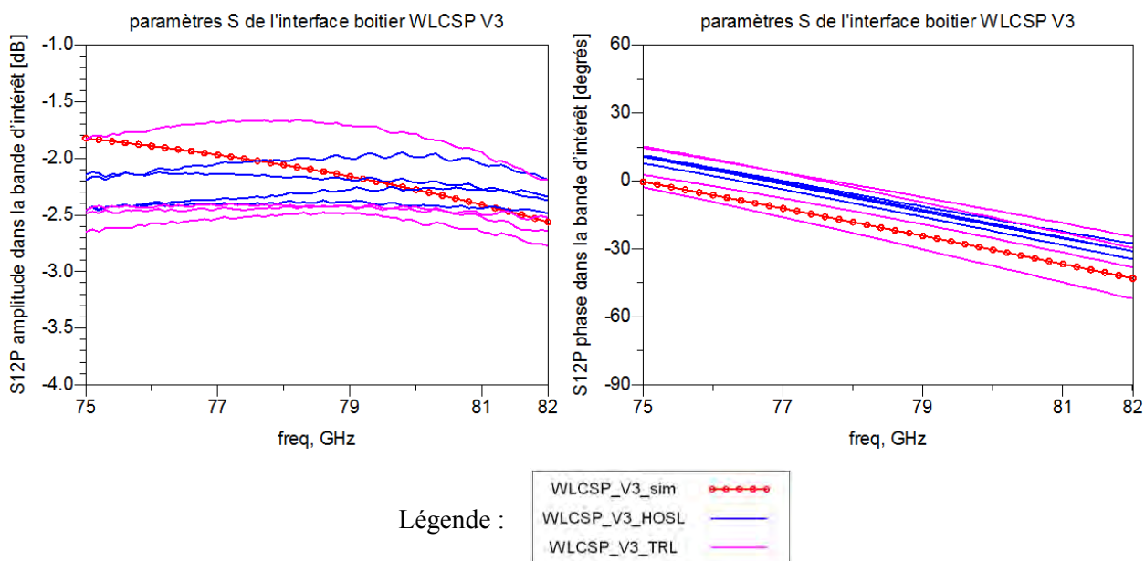
Figure 71 : comparaison des simulations et des mesures de l'interface boitier WLCSP V3 par les méthodes Half-OSL et TRL
