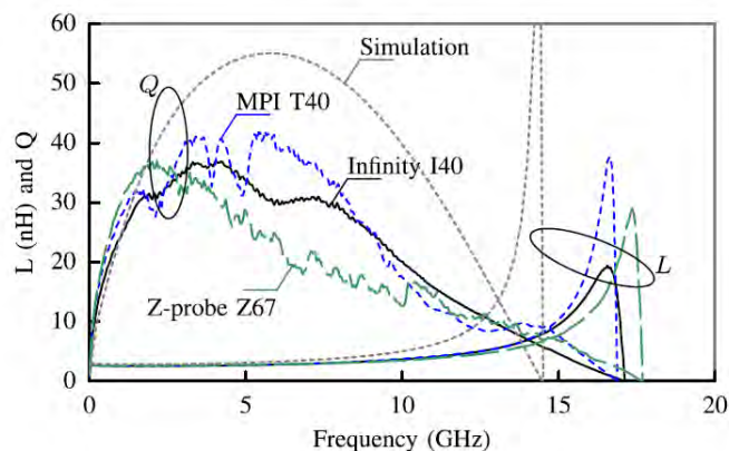
Figure 40 : coefficient de qualité simulé et mesuré en fonction du type de pointes [2.11]
