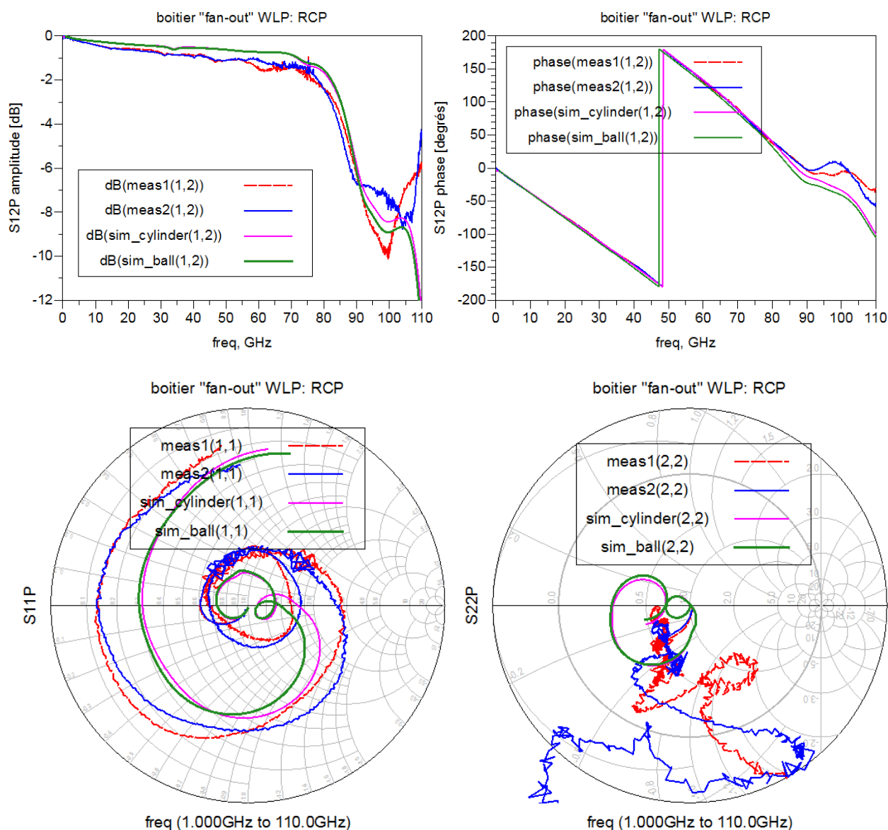
Figure 54 : comparaison des simulations et des extractions par la mesure des paramètres S du boîtier RCP
