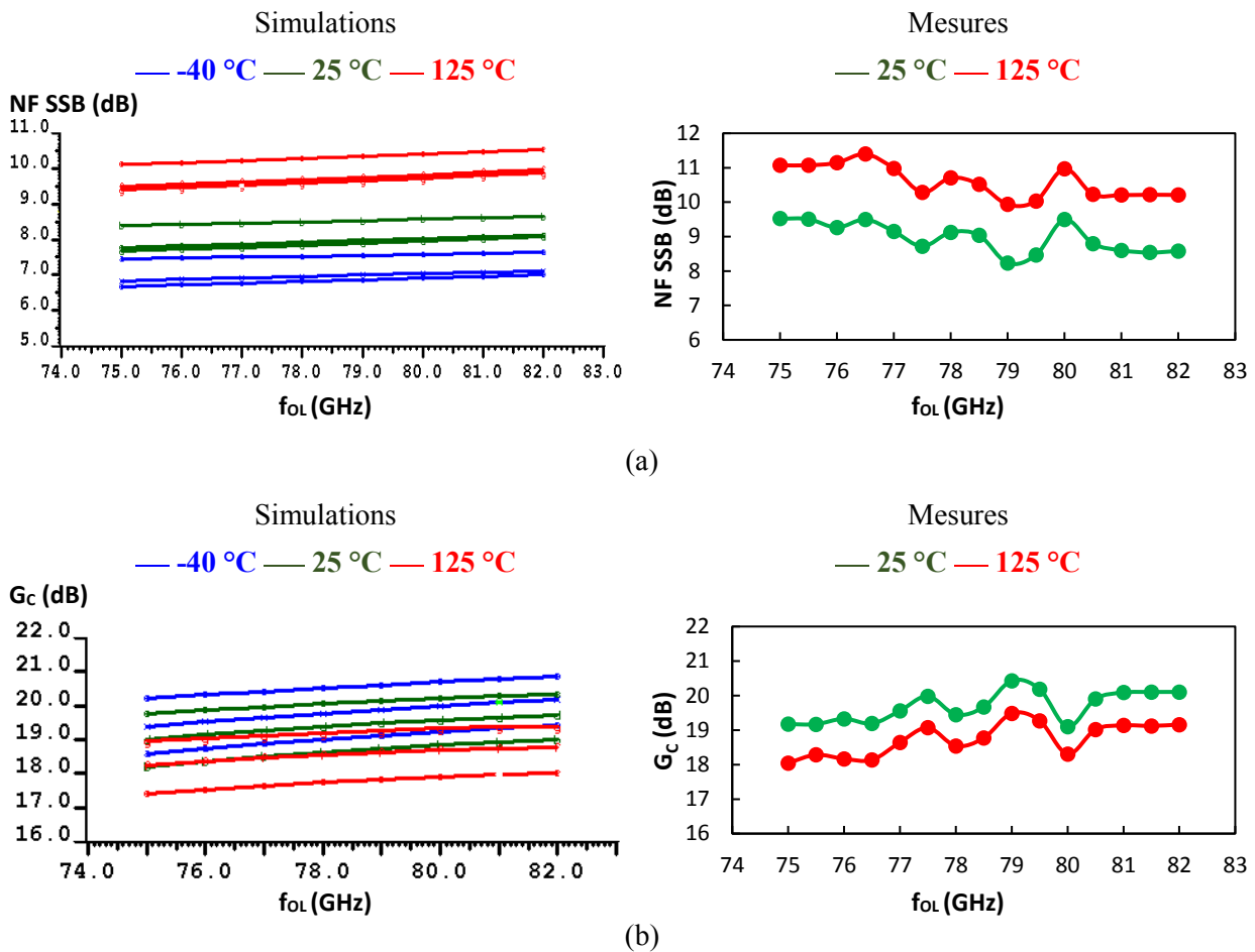
Figure 95 : comparaison des simulations et des mesures du facteur de bruit SSB (NF SSB) (a) et du gain de conversion (G c ) (b) du mélangeur actif en puce nue en fonction de la fréquence OL (f OL ) pour f FI = 1 MHz pour différentes températures
