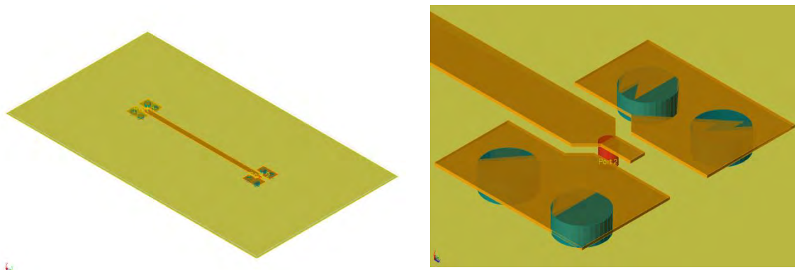
Figure 47 : modèle de la ligne PCB incluant les plots
