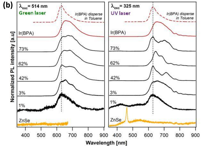
Figure 16: (a) PL régime d'expérience où les échantillons sont excités en utilisant UV et lasers verts. (b) PL spectre normalisé RT de ZnSe+Ir(BPA) des films épais composites, déposés sur des substrats en quartz sous 514 nm (laser vert) et 325 nm (laser UV) d'excitation ainsi que les spectres de ZnSe vierge (de plus basse) et colorant (deuxième à partir du haut) des films et des molécules de colorant dans une solution de toluène (le plus élevé). Tous les spectres sont normalisés à l'intensité maximale PL. Les pourcentages de colorant contenu comme indiqué sont obtenus à partir des intensités intégrées de la PL composites par rapport à celle de la couche de colorant vierge.
