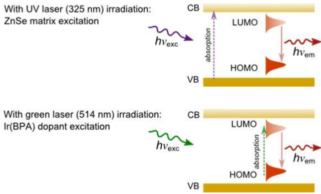
Figure 16: (a) PL régime d'expérience où les échantillons sont excités en utilisant UV et lasers verts. (b) PL spectre normalisé RT de ZnSe+Ir(BPA) des films épais composites, déposés sur des substrats en quartz sous 514 nm (laser vert) et 325 nm (laser UV) d'excitation ainsi que les spectres de ZnSe vierge (de plus basse) et colorant (deuxième à partir du haut) des films et des molécules de colorant dans une solution de toluène (le plus élevé). Tous les spectres sont normalisés à l'intensité maximale PL. Les pourcentages de colorant contenu comme indiqué sont obtenus à partir des intensités intégrées de la PL composites par rapport à celle de la couche de colorant vierge.
