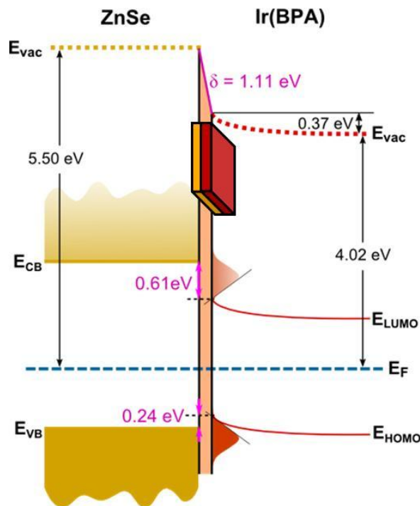
Figure 8: Interface diagramme de bande de la bicouche ZnSe/Ir(BPA), y compris un grand dipôle de l'interface de 1,11 eV et de la bande de flexion dans l'émetteur de 0,37 eV.
