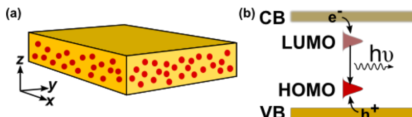
Figure 4: (a) Représentation schématique du composite en vrac proposé comme une couche active électroluminescente pour HLEDs comprenant d'une matrice de semi-conducteur inorganique dopé avec de petites molécules organiques et (b) le diagramme de niveau d'énergie désignée correspondant pour le transfert direct d'électrons/trous de la inorganique large semi-conducteur à bande interdite les dopants de matrice à émission radiative ultérieure de dopants.
