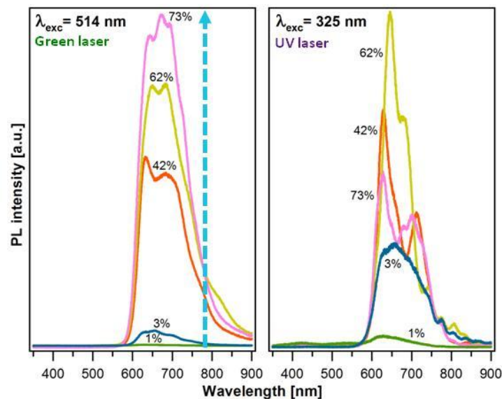
Figure 17: Spectres PL superposée des composites dans le cadre du 514 nm et 325 nm excitation laser. Avec une excitation laser UV, la luminescence du colorant dans les 1% et 3% des composites est améliorée par rapport à la luminescence des composites avec la grande teneur en colorant.
