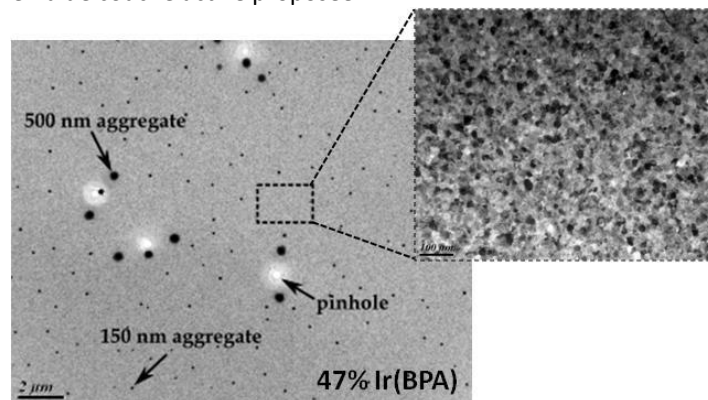
Figure 9: Images TEM d'une ZnSe+Ir(BPA) de composite avec un film de pourcentage en volume de 47 Ir(BPA). L'agrégation du colorant augmente avec la quantité accrue de concentration de colorant dans le film composite.
