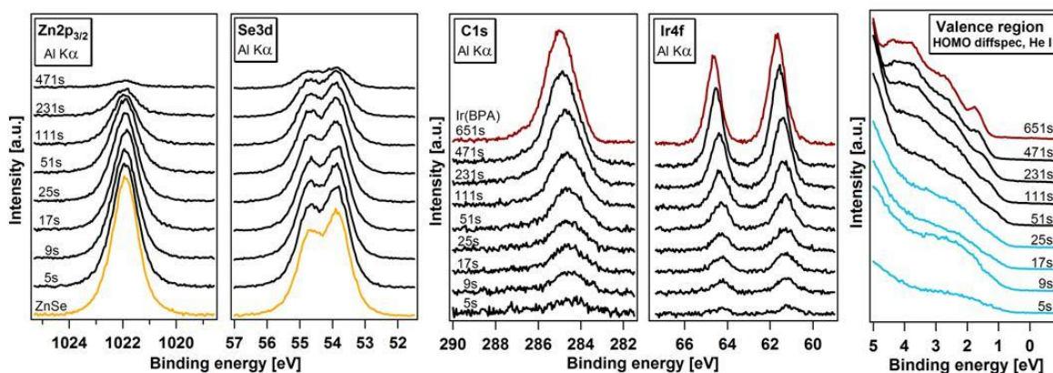
Figure 11: Zn2p 3/2 et Se3d spectres d'émission du substrat de ZnSe, ainsi que les C1s, Ir4f et des spectres d'émission de zone de valence de l'Ir(BPA) surcouche pendant le dépôt par étapes de Ir(BPA) sur ZnSe. Les Ir(BPA) des temps de dépôt sont indiqués.
