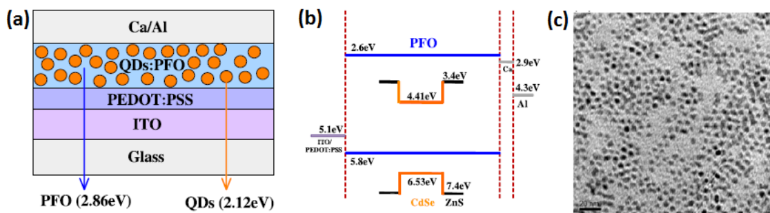
Figure 3: (a) Un schéma d'une structure de dispositif à couche unique qui montre les points quantiques de CdSe/ZnS noyées dans une couche de PFO sandwich entre ITO et Ca/Al électrodes. Les flèches indiquent les pics d'énergie EL des boîtes quantiques et PFO. (b) Energy niveau schéma du dispositif, où toutes les énergies sont indiquées par rapport au niveau de vide. (c) HR-TEM de 80% en poids QD intégré dans PFO. 7
