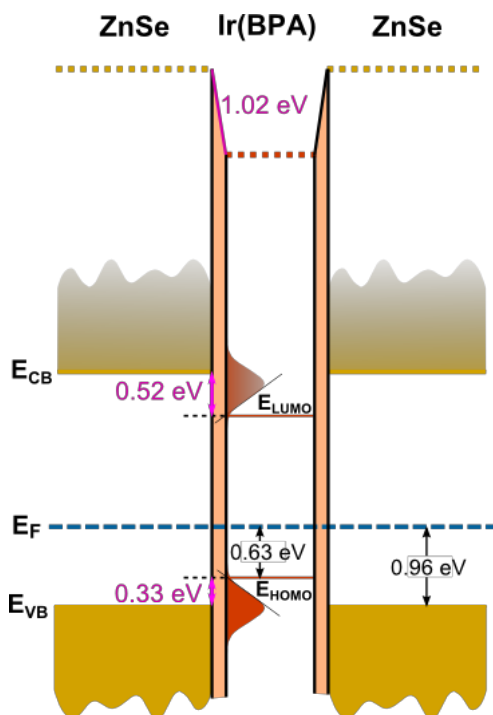
Figure 10: L'alignement de la bande de l'énergie au niveau des interfaces internes de la 19% ZnSe+Ir(BPA) composite. Ce diagramme de bande affiche les orbitales colorant frontalières étant pris en sandwich par les niveaux d'énergie de ZnSe. La différence mesurée \phi du ZnSe et de la vierge calculé \phi du colorant dans le matériau composite est affecté à une interface de dipôle 1,02 eV qui mène à la gamme de mesure.
