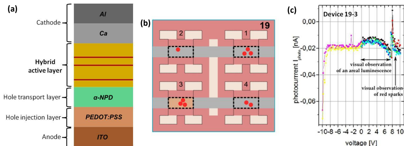
Figure 18: (a) Schéma de la structure Périphérique 19 section. La couche active est composée d'une alternance de 4 ZnSe et 3 Ir(BPA) couches. (b) Haut-vue image schématique montrant 4 appareils sur un substrat. Les régions actives des dispositifs sont définies par les rectangles en pointillés. Tous les dispositifs émis plusieurs étincelles rouges faibles qui ont duré aussi longtemps que le courant n'a pas finalement brûler les dispositifs appliqués. Dispositif 19-3 présentait une faible émission surfacique de pâle teinte orangée. (c) Plot du photocourant généré sur une photodiode au silicium contre la tension appliquée sur l'appareil 19-3.
