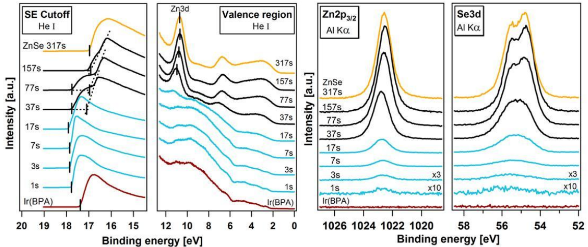
Figure 13: SE spectres coupure et la région d'émission de valence, ainsi que les spectres Zn 2p_{3/2} et Se3d émission de la sur-couche de ZnSe pendant le dépôt par étapes de Zn sur Ir(BPA). Les temps de dépôt de ZnSe sont indiqués.
