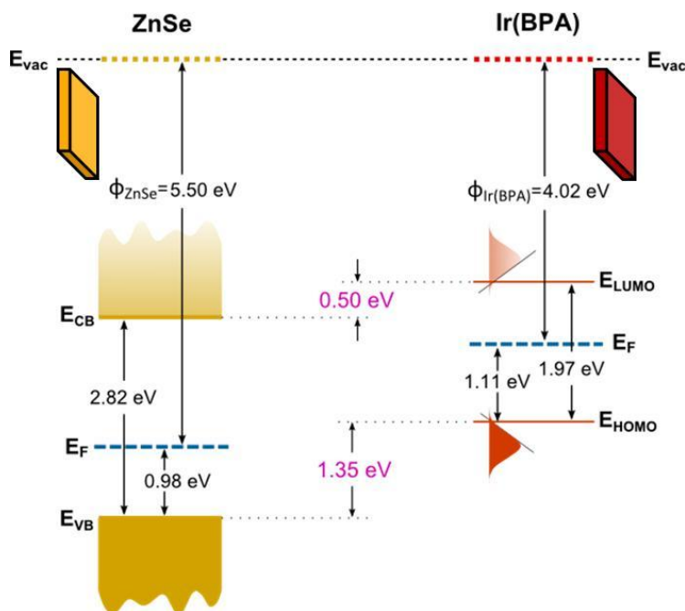
Figure 7: Les niveaux d'énergie de la ZnSe vierge et Ir(BPA) couches dans une gamme Anderson qui suppose un niveau de vide commune pour les deux matériaux. Avant le contact, en alignant les niveaux de vide révèle un alignement du niveau d'énergie défavorables pour notre conception hybride proposée.
