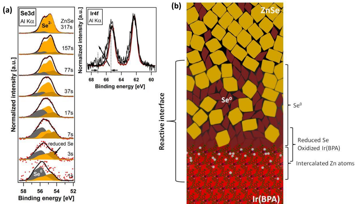
Figure 14: (a) Pic équipée Se3d photoémission spectres (bon ajustement est obtenu avec trois contributions qui sont affectés à élémentaire Se 0 , Se 2- en ZnSe et un volet Se plus réduite). Spectres d'émission Ir4f révèlent clairement espèces énergie de liaison élevés qui sont prononcés près de l'interface. (b) Une représentation de l'Ir(BPA)/ZnSe bicouche, qui présente une interface de matériel très impur.
