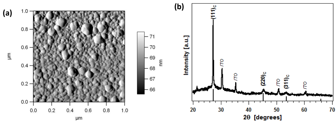
Figure 5: (a) Image AFM de la surface et (b) diagramme de XRD (avec des marques le long de la barre sur l'axe des x) pour l'essentiel d'un film de ZnSe déposée par évaporation thermique sur un substrat en verre d'ITO.
