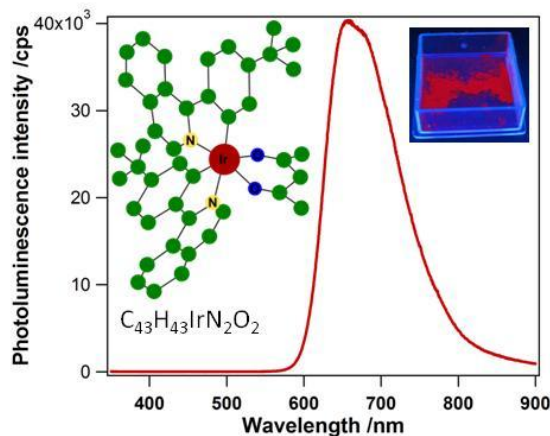
Figure 6: PL spectres du colorant Ir(BPA) sous une excitation laser vert avec sa structure moléculaire et d'une image numérique de la poudre de colorant est exposé à un éclairage UV.
