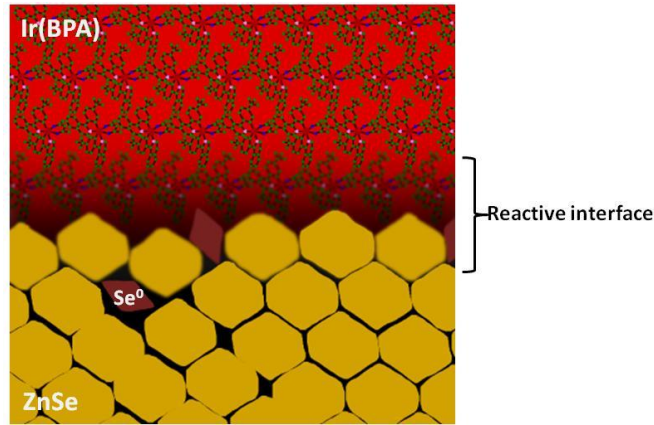
Figure 12: Une représentation de la bicouche ZnSe/Ir(BPA), qui dispose d'une interface réactive.
