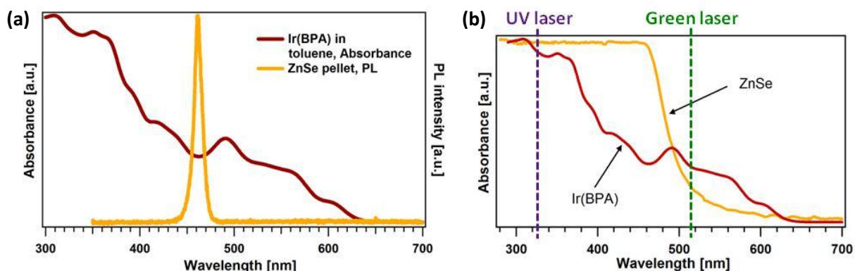
Figure 15: (a) Spectre de photoluminescence d'une pastille de ZnSe montré avec le spectre d'Ir(BPA) de molécules dispersées dans du toluène pour démontrer le chevauchement spectral total, ce qui indique la probabilité de résonance transfert d'énergie de l'exciton de ZnSe à Ir(BPA) molécules absorption. (b) Les spectres d'absorption de Ir(BPA) et ZnSe montrant que les deux matériaux peuvent être excités par un laser à haute énergie.
