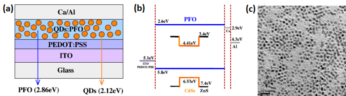
Figure 3: (a) Un schéma d'une structure de dispositif à couche unique qui montre les points quantiques de CdSe/ZnS noyés dans une couche de PFO sandwich entre ITO et Ca/Al électrodes. Les flèches indiquent les pics d'énergie EL des boîtes quantiques et PFO. (b) Energy niveau schéma du dispositif, où toutes les énergies sont indiquées par rapport au niveau de vide. (c) HR-TEM de 80% en poids QD intégré dans PFO. 7
