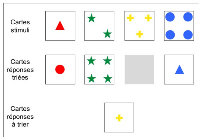
Figure 4. Configuration du Wisconsin Card Sorting Test pour un tri en fonction du critère de couleur.
