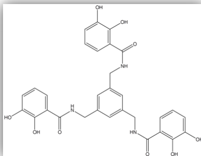
Figure 9 : Structure du sidérophore MECAM.
