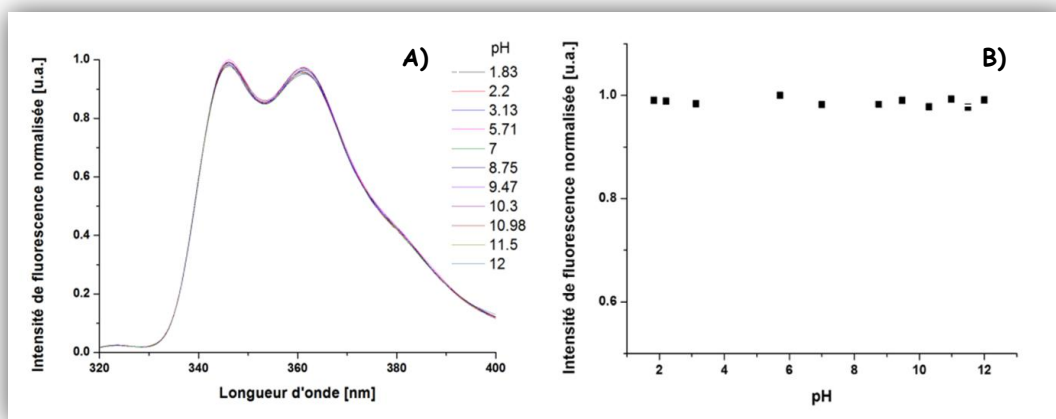
Figure 24 : A) Spectre d'émission de fluorescence de la sonde ( 5 \cdot 10^{-7} \text{ M} ) dans l'eau en fonction du pH. B) Intensité de fluorescence de la sonde à 346 nm en fonction du pH.
