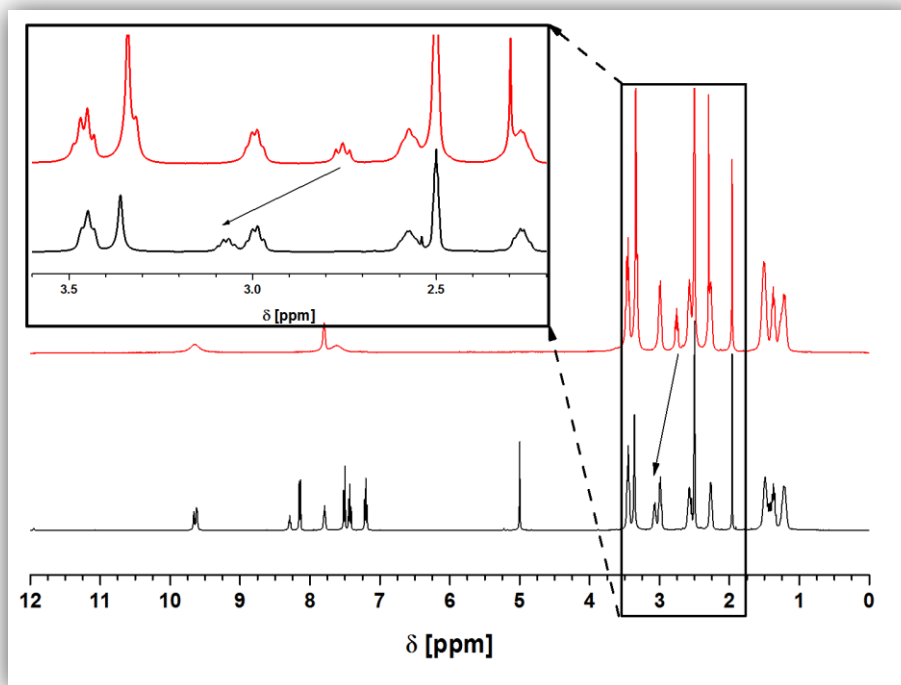
Figure 38 : Spectres RMN ^1\text{H} dans le DMSO de la déféroxamine B (haut) et de la sonde CBZ-DFO (bas).
