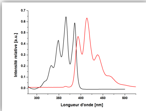
Figure 11 : Spectre UV de la sonde ANT-CE à 5.10^{-5} M dans le méthanol (noir) et spectre d'émission fluorescence dans le méthanol ( \lambda_{ex} = 366 nm) (rouge).
