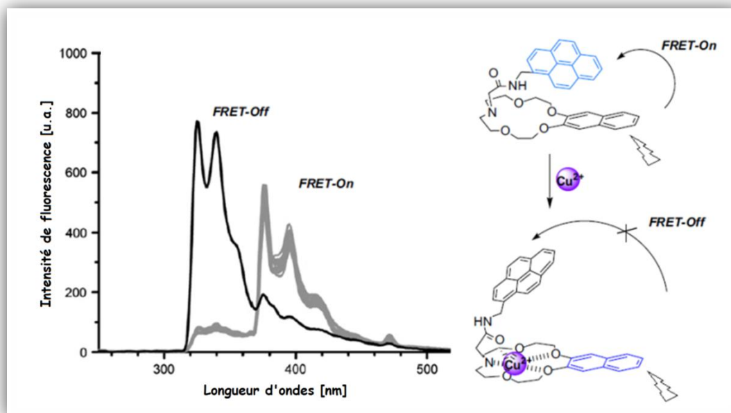
Figure 26 : Illustration du principe de FRET. 67
