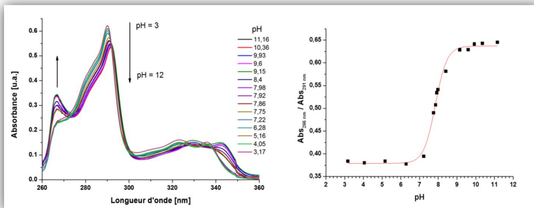
Figure 35: Influence du pH sur le spectre ultraviolet de la sonde CBZ-RED.
