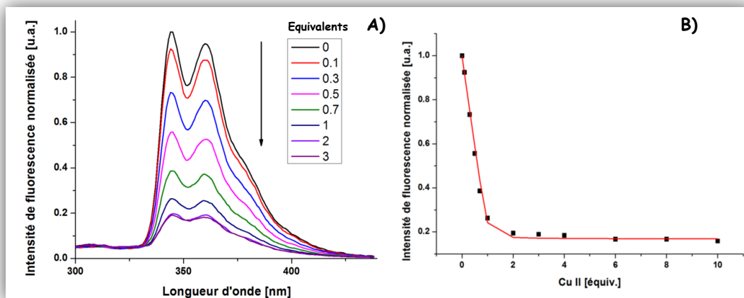
Figure 41 : A) Emission de fluorescence de la sonde 16 ( 2 \cdot 10^{-7} M ; \lambda_{ex} = 232 nm) en présence de cuivre II dans le méthanol. B) Suivi de la décroissance de fluorescence expérimentale à 345 nm (points) et théorique (ligne rouge).
