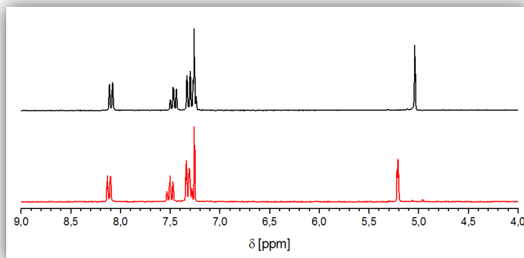
Figure 18: Spectre RMN dans \text{CDCl}_3 de l'acide carboxylique 11 (noir) et du fluorure d'acyle 13 (rouge).
