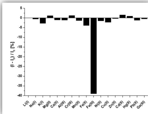
Figure 25: Modification du signal de fluorescence de la sonde 14 ( 0,5 \mu\text{M} , \lambda_{\text{ex}}=292 \text{ nm} ) enregistré en milieu aqueux suite à l'ajout de 200 équivalents de divers métaux sous forme de perchlorates.
