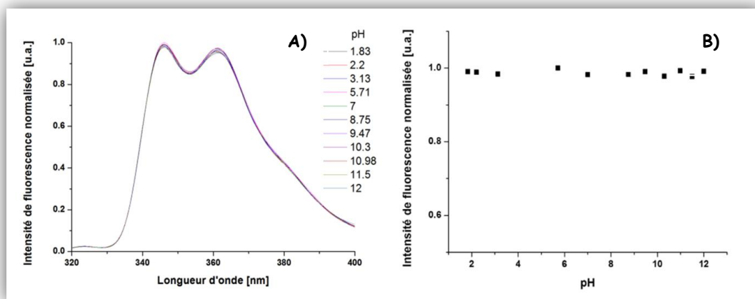
Figure 24 : A) Spectre d'émission de fluorescence de la sonde ( 5 \cdot 10^{-7} \text{ M} ) dans l'eau en fonction du pH. B) Intensité de fluorescence de la sonde à 346 \text{ nm} en fonction du pH.
