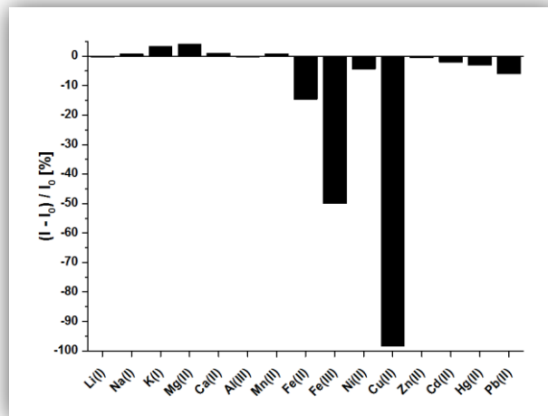
Figure 21: Modification du signal de fluorescence de la sonde 14 ( 0,5 \mu\text{M} , \lambda_{\text{ex}}=292 \text{ nm} ) enregistrée dans l'acétonitrile aqueux suite à l'ajout de 200 équivalents de divers métaux sous forme de perchlorate.
