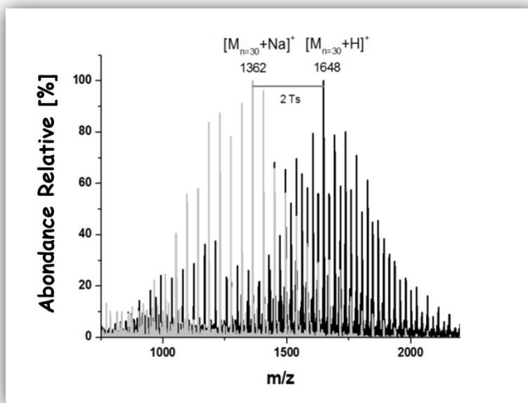
Figure 2 : Spectres de masses du PEG 1500 avant (gris) et après tosylation (noir).
