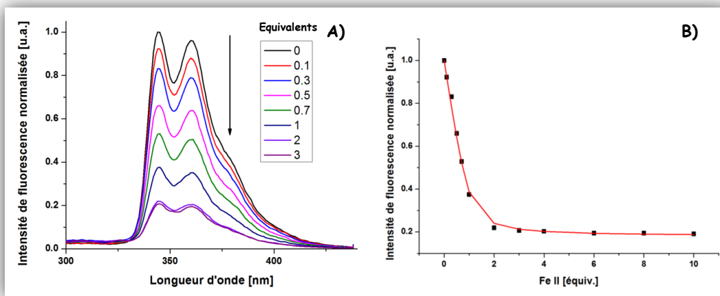
Figure 40 : A) Emission de fluorescence de la sonde 16 ( 2 \cdot 10^{-7} M ; \lambda_{ex} = 232 nm) en présence de fer II dans le méthanol. B) Suivi de la décroissance de fluorescence expérimentale à 345 nm (points) et théorique (ligne rouge).
