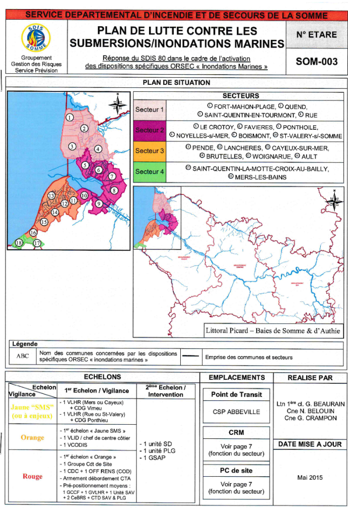
Figure 2.3 : Plan de lutte contre les submersions marines de la Somme à destination du SDIS 80
