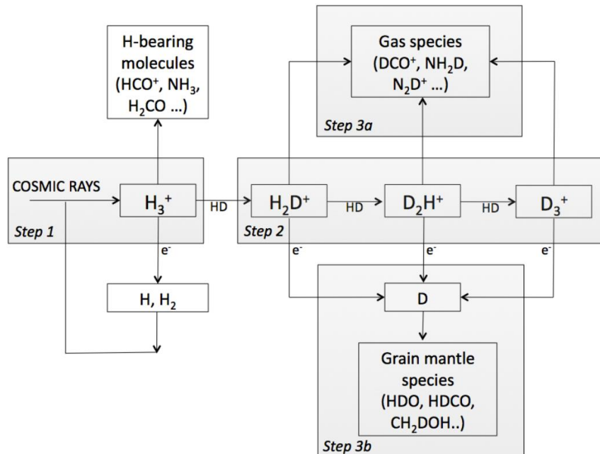
Figure 2.2.5 : Schéma des trois étapes expliquant la formation de matière enrichie en deutérium dans un environnement froid ( T < 30 K). Figure extraite de [77].
