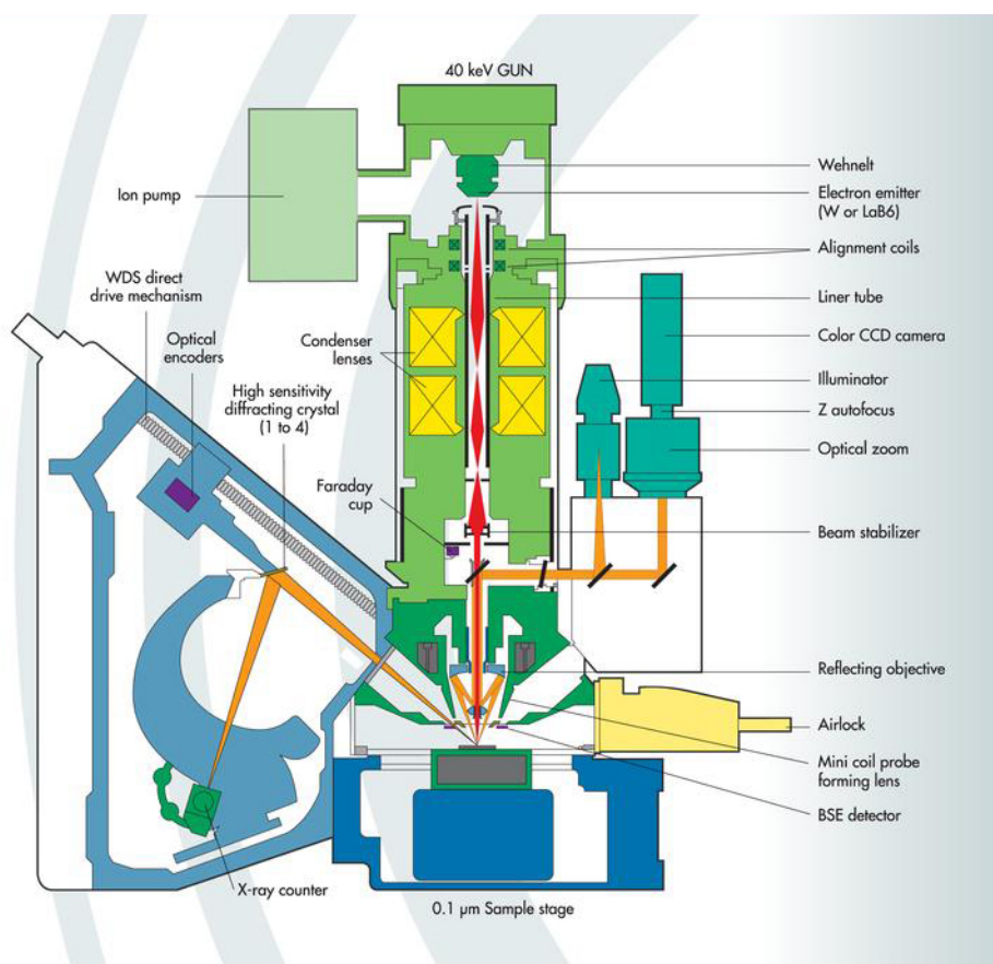
Figure 3.2.2 : Schéma fonctionnel de la microsonde électronique CAMECA SX-100. Crédits : CAMPARIS.
