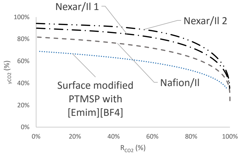
Figure 41. Performance de séparation des 4 membranes liquide ionique synthétisées dans le cadre du projet HiPerCap pour un rapport de pression ( \psi ) de 0,1.
