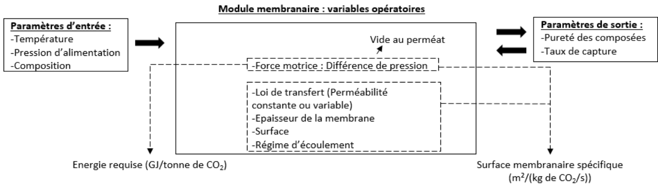
Figure 30. Détails des entrées et sortie d'un programme de module membranaire
