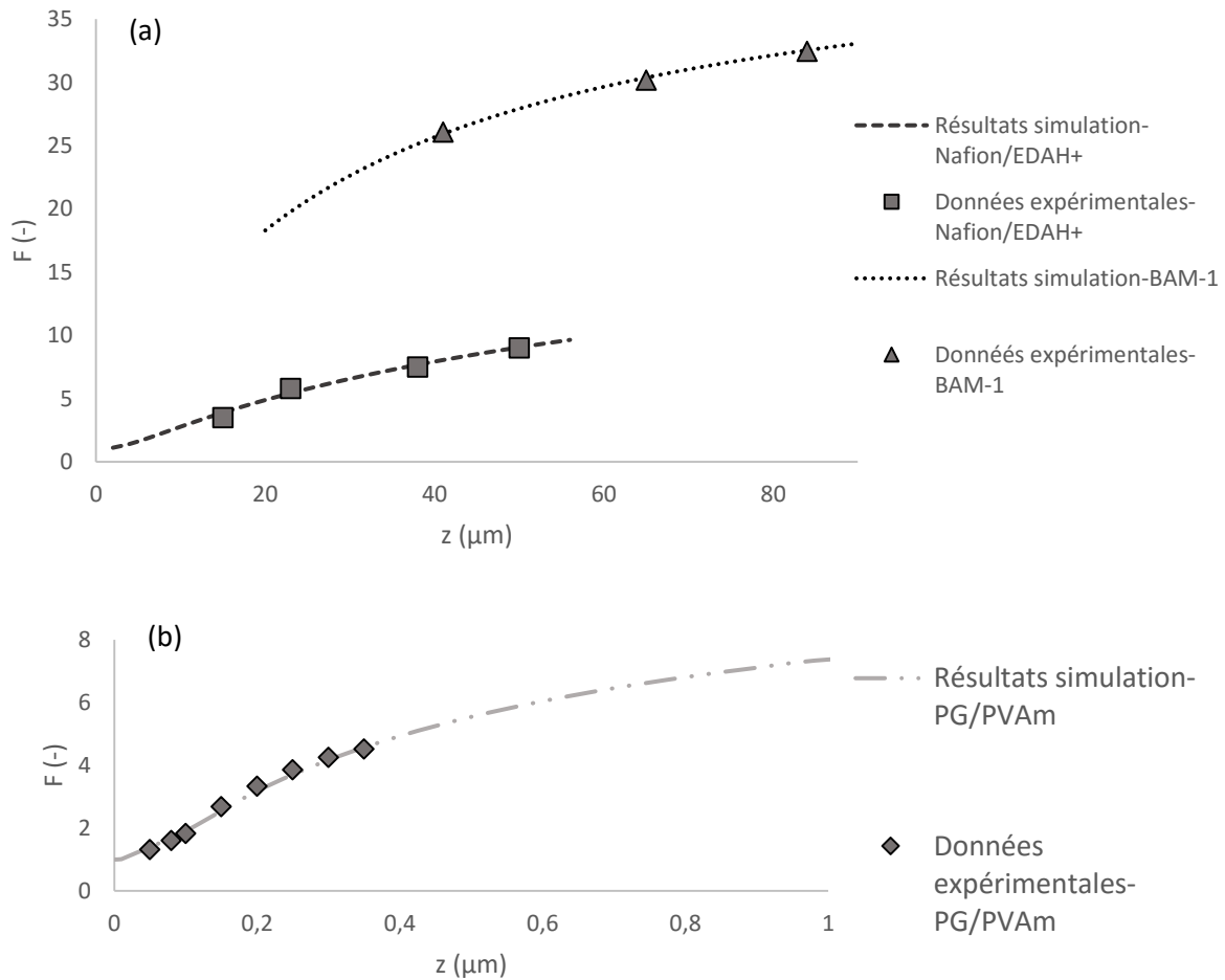
Figure 67a et 67b. Evolution du facteur de facilité dans une membrane réactive en fonction de l'épaisseur de la membrane.
