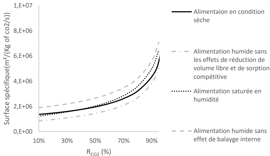
Figure 47. Comparaison de la surface spécifique du module membranaire en condition sèche et humide et évaluation de l'influence des deux phénomènes ( \psi = 0,1 ; p' = 1 \text{ bar} et p'' = 0,1 \text{ bar} ).
