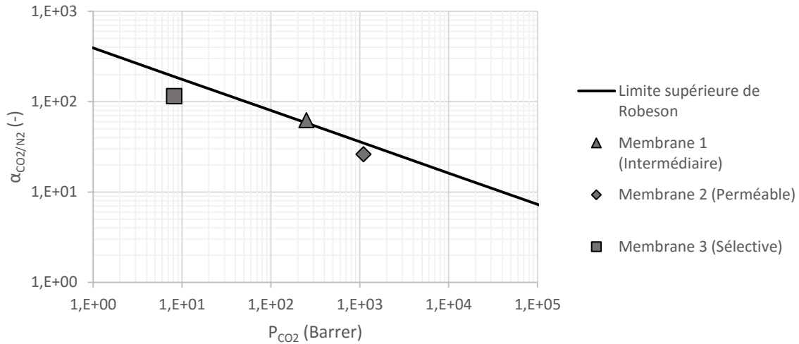
Figure 33. Performances de séparation des trois membranes (Tableau 13)
