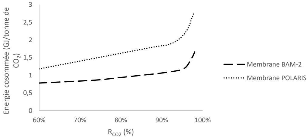
Figure 64. Comparaison sur l'énergie consommée entre la membrane BAM-2 et la membrane POLARIS avec une alimentation CO 2 /N 2 (15%/85% en base sèche et y CO2 =70%)
