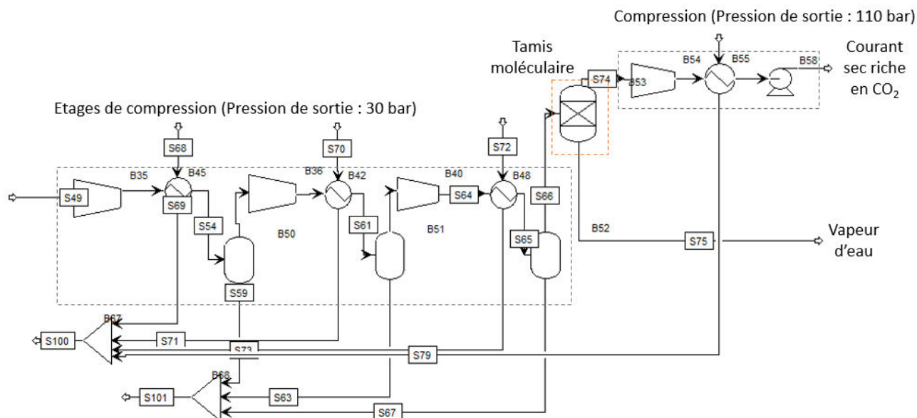
Figure 75. Description du procédé de séchage par adsorption avec un tamis moléculaire
