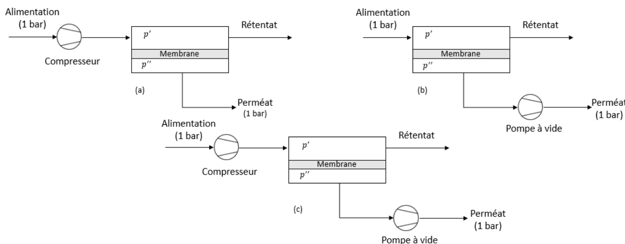
Figure 4. Schéma des différentes possibilités de force motrice dans un étage de perméation gazeuse : (a) compression, (b) vide, (c) compression et vide
