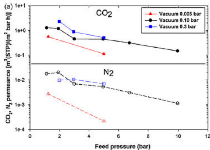
Figure 94. Evolution de la perméance du CO 2 en fonction de la pression amont pour différents vides [105]
