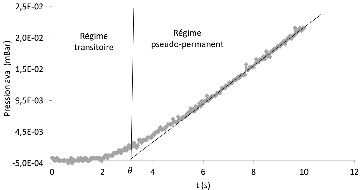
Figure 55. Evolution de la pression dans la chambre aval du système expérimental. Détermination de la perméabilité de CH 4 à travers une membrane PDMS de 100 μm à une température de -5°C.
