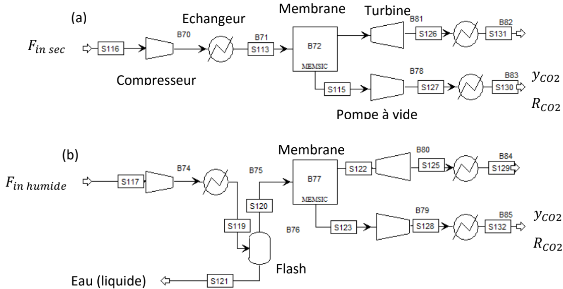
Figure 45. Schéma d'un procédé de perméation gazeuse développé dans l'environnement de simulation ASPEN PLUS. Comparaison des performances de séparation (voir Tableau 17) d'une membrane Matrimid de 1 \mu\text{m} avec un flux sec (a) et un flux humide (b)
