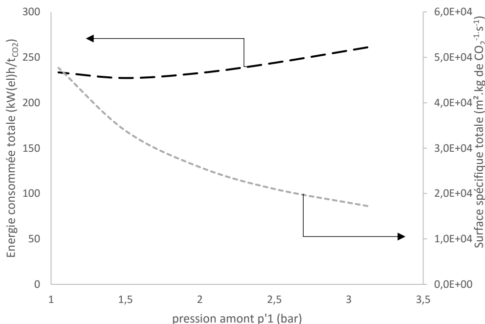
Figure 87. Etude du compromis entre la compression et le vide sur la première membrane du procédé. Le taux de capture en CO 2 ( R_{\text{CO}_2} ) du procédé est de 85% pour une pureté en CO 2 ( y_{\text{CO}_2} ) de 95%. Le rapport de pression de la première membrane ( \psi_1 ) est de 0,08 et le rapport de pression de la seconde membrane ( \psi_2 ) est de 0,1.
