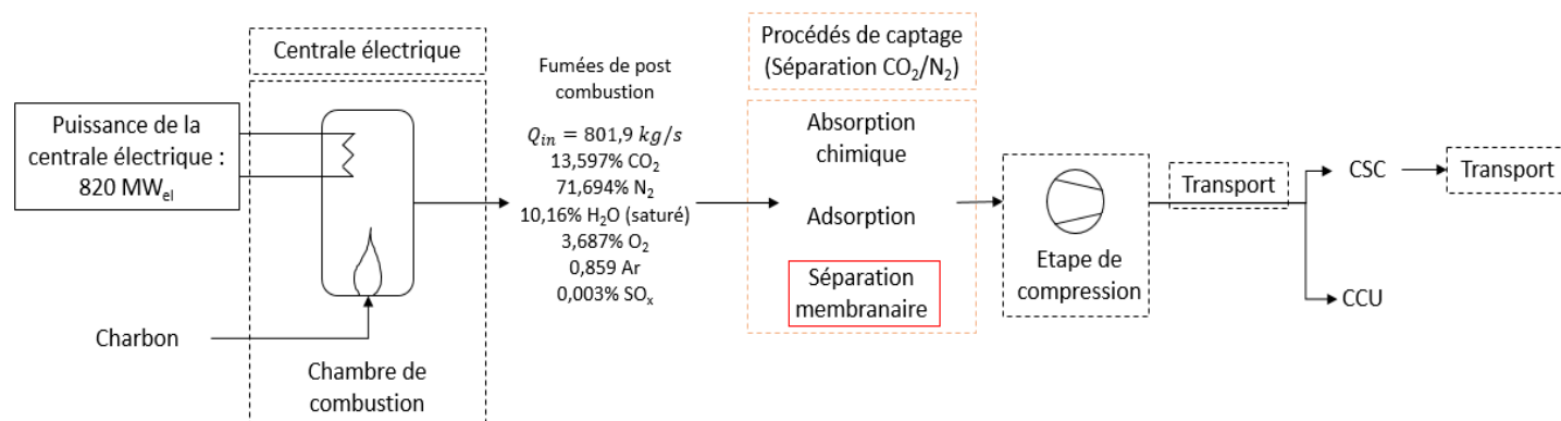
Figure 1. Schéma du captage du CO 2 en post combustion à partir de la centrale à charbon étudiée dans le projet HiPerCap [4]
