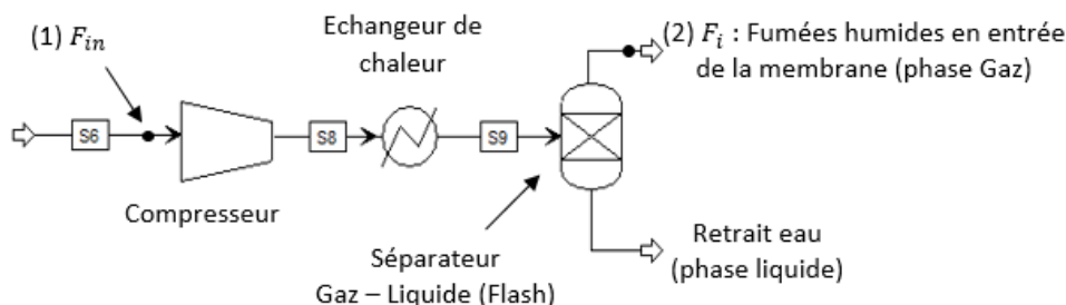
Figure 42. Représentation d'un compresseur isotherme dans l'environnement de simulation Aspen Plus. F_{in} : Flux d'alimentation initial / F_i : Flux en entrée du module membranaire (sortie de séparateur)
