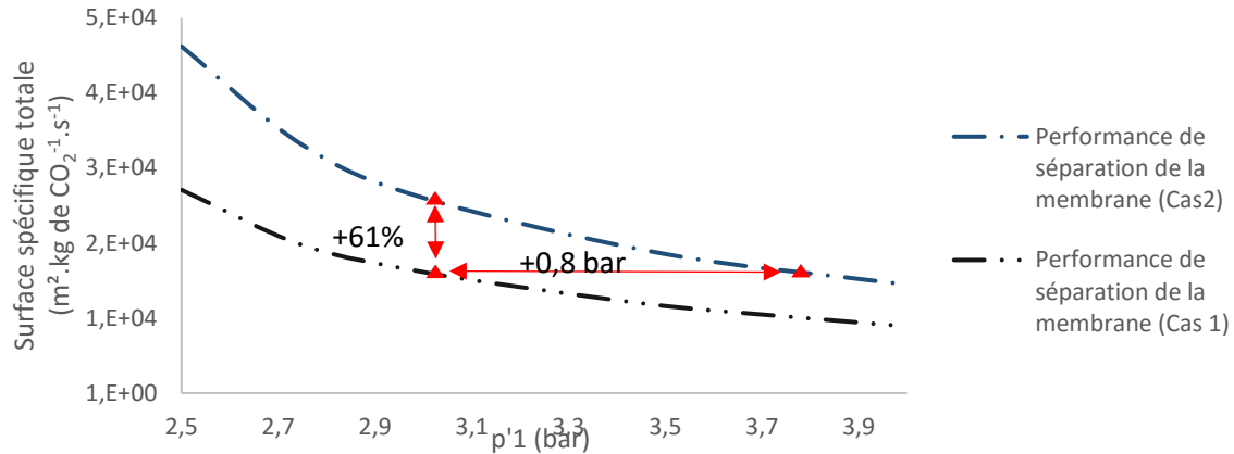
Figure 88. Résultats de la simulation sur la comparaison entre le cas 1 et le cas 2 en fonction de la variation de la pression amont du premier étage ( p'_1 ). Le taux de capture global ( R_{CO_2} ) est de 85% pour une pureté en CO 2 ( y_{CO_2} ) de 95% en sortie de procédé. ( p'_1 = 0,25 bar ; \psi_2 = 0,1 ; p'_2 = 2,5 bar et p''_2 = 0,25 bar)
