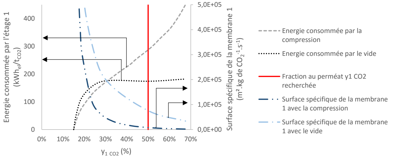
Figure 85. Estimation de l'énergie consommée et de la surface spécifique du premier module membranaire du procédé de perméation gazeuse. Le taux de capture en CO 2 ( R_{CO_2 M_1} ) est fixé à 92,2%.
