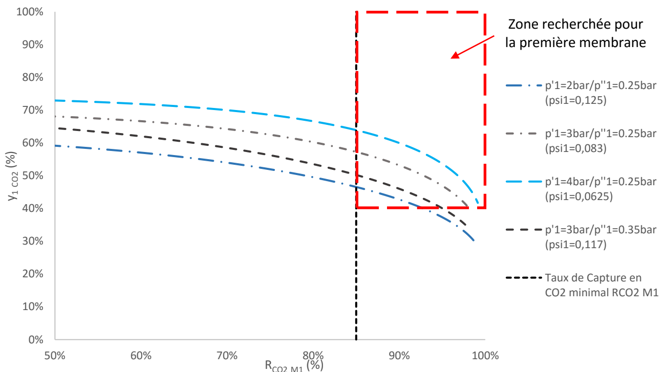
Figure 81. Courbes de pureté de la membrane réactive du cas 1 pour différents rapports de pression ( \psi_1 ).
