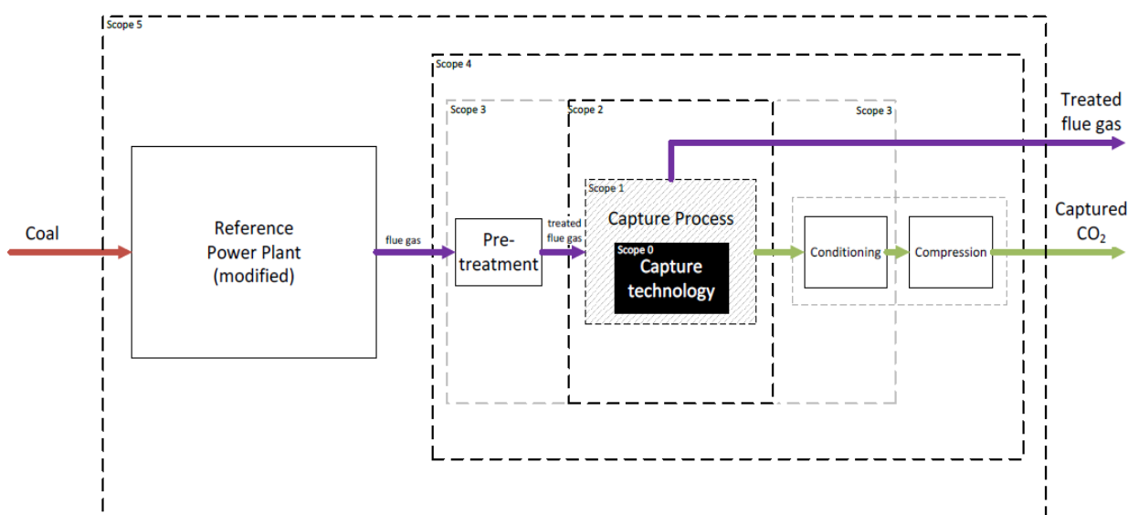
Figure 72. Schéma général d'une centrale électrique avec un module de captage de CO 2
