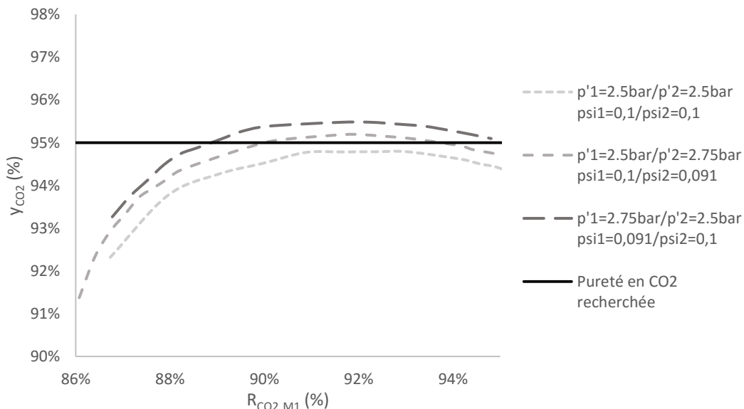
Figure 83. Détermination des pressions amont minimales à appliquer à chaque étage du procédé pour atteindre un taux de capture en CO 2 ( R_{CO_2} ) global de 85% et une pureté ( y_{CO_2} ) de 95% ( p''_1 = p''_2 = 0,25\text{bar} ). Le taux de capture en CO 2 global ( R_{CO_2} ) est de 85%.
