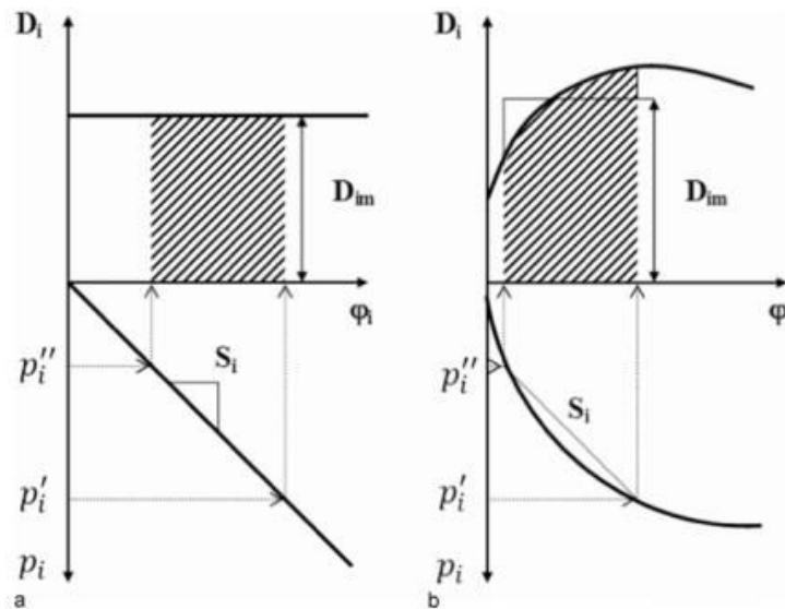
Figure 26a et 26b. Schémas représentatifs de l'évolution de la sorption et de la diffusion du mécanisme SD en fonction de la pression partielle pour un modèle perméabilité constante (a) et pour un modèle perméabilité variable (b) ( \varphi_i : fraction de concentration sorbée dans la membrane) [129].
