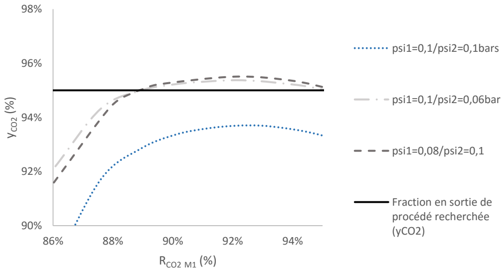
Figure 86. Détermination des rapports de pression du premier et second étage ( \psi_1 et \psi_2 ) du procédé de perméation gazeuse avec deux membranes physiques. Le taux de capture global ( R_{CO_2} ) est fixé à 85%.
