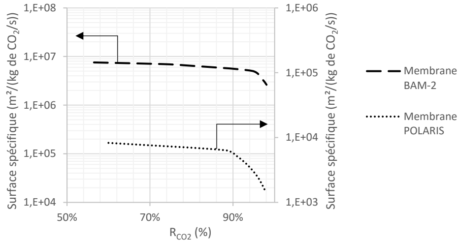
Figure 65. Comparaison de la surface spécifique de la membrane BAM-2 et de la membrane POLARIS avec une alimentation CO 2 /N 2 (15%/85% en base sèche et y CO 2 =70%)
