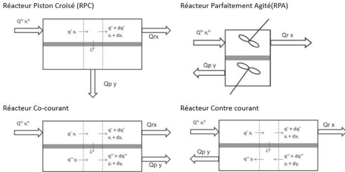
Figure 31. Les différents types d'écoulement intégrés dans MEMSIC
