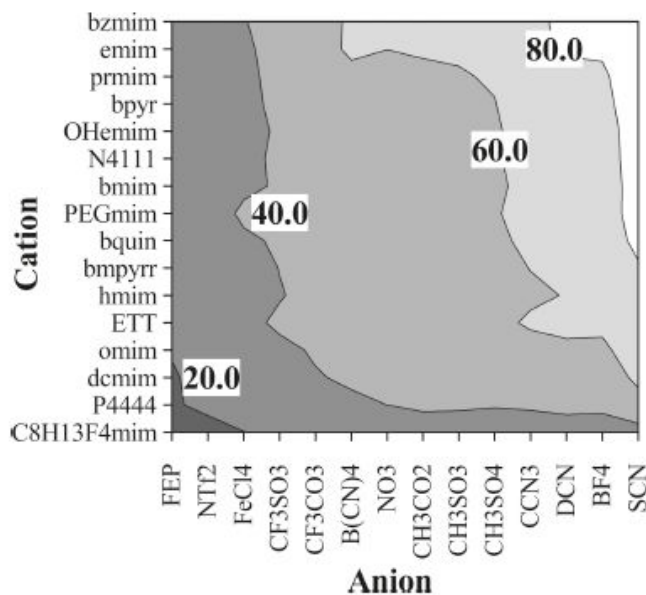
Figure 16. Sélectivité CO 2 /N 2 en fonction du choix de l'anion et du cation du liquide ionique [62]
