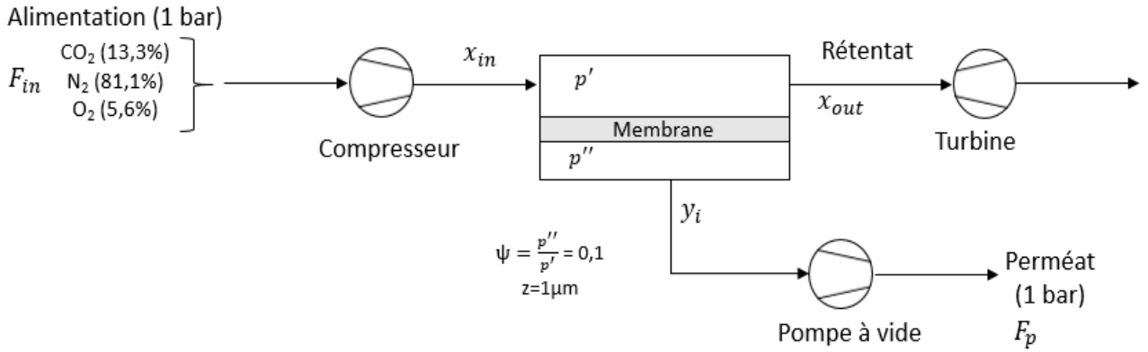
Figure 32. Schéma d'un procédé de perméation membranaire à un étage avec un compresseur, une pompe à vide et une turbine
