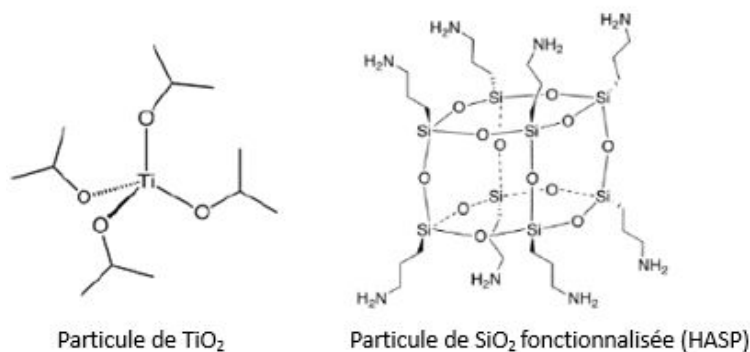
Figure 18. Description des différentes molécules dispersées dans les MMMs ou les membranes hybrides
