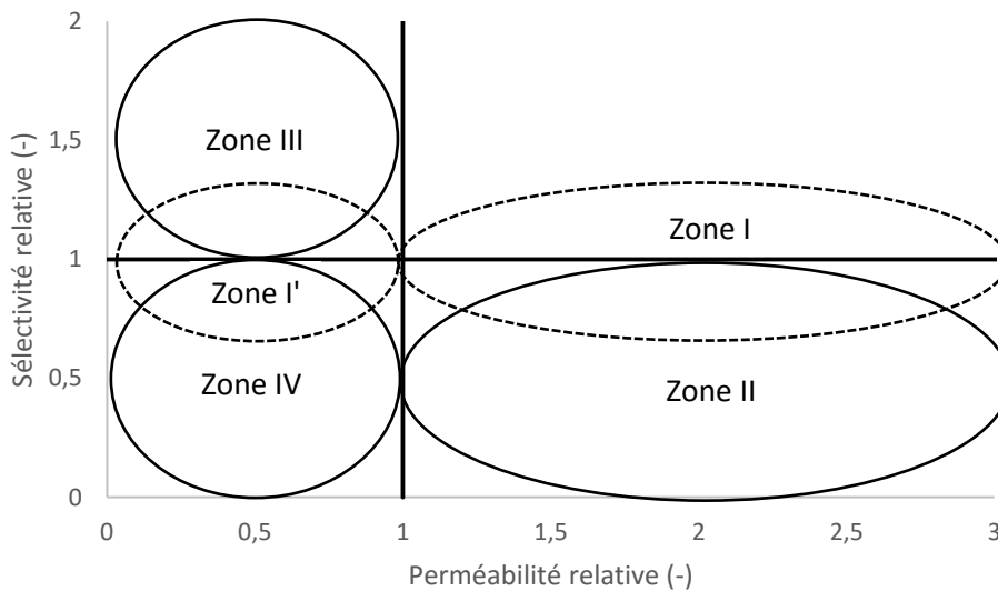
Figure 24. Impact des différentes interactions polymère-particule (Trait pointillé : cas idéal / trait plein : réalité)
