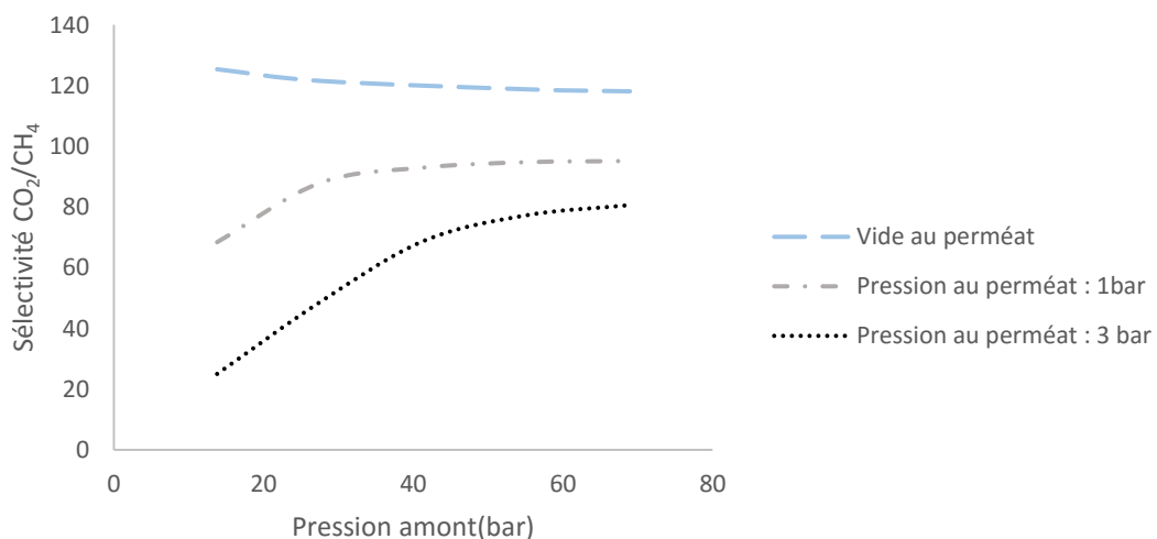
Figure 51. Evaluation de la sélectivité avec différents cas de pression amont/pression aval pour la séparation d'un binaire CO 2 /CH 4
