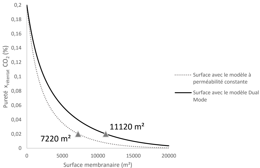
Figure 53. Evaluation de la surface spécifique de la membrane 6FDA-TAPDO (épaisseur 2 μm) en fonction de la fraction de CO 2 au rétentat. La composition du mélange binaire CO 2 /CH 4 est 30%/70% pour un régime d'écoulement piston croisé.
