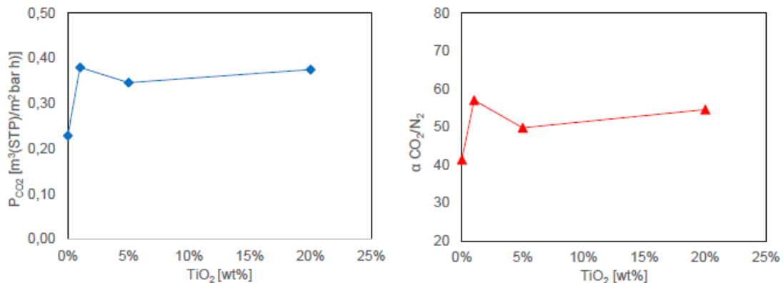
Figure 22. Perméance du \text{CO}_2 pur dans la MMM PVA/ \text{TiO}_2 (bleu) et sélectivité \text{CO}_2/\text{N}_2 en fonction de la fraction massique de \text{TiO}_2 [123]
