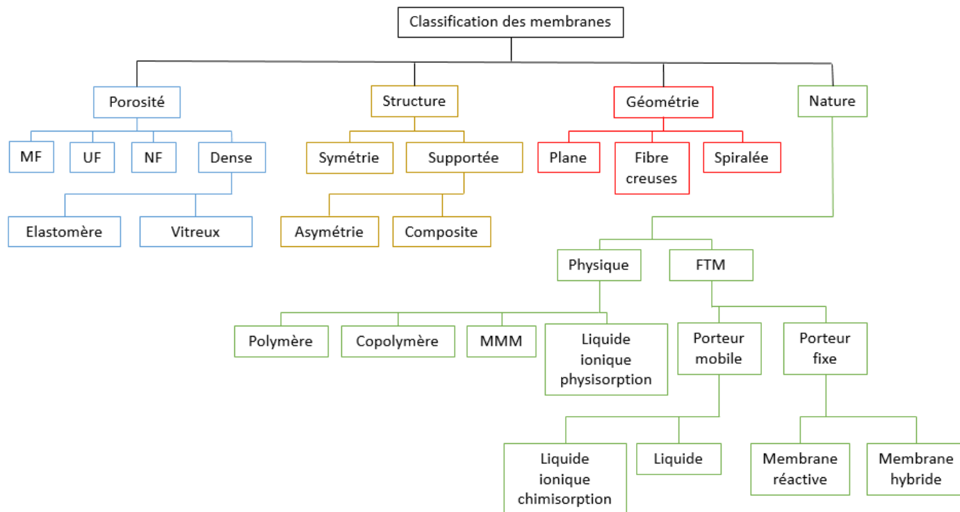
Figure 20. Classification des principales caractéristiques d'une membrane pour des applications en perméation gazeuse
