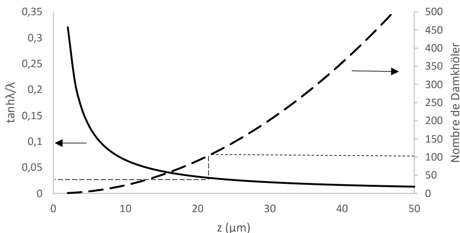
Figure 69. Evolution du nombre de Damköhler et du paramètre \frac{\tanh(\lambda)}{\lambda} pour la membrane BAM-1
