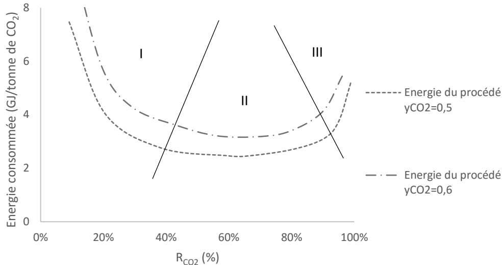
Figure 36. Variation de l'énergie dans une étape de pré-concentration avec une pureté de CO 2 constante à 50% et à 60% au perméat
