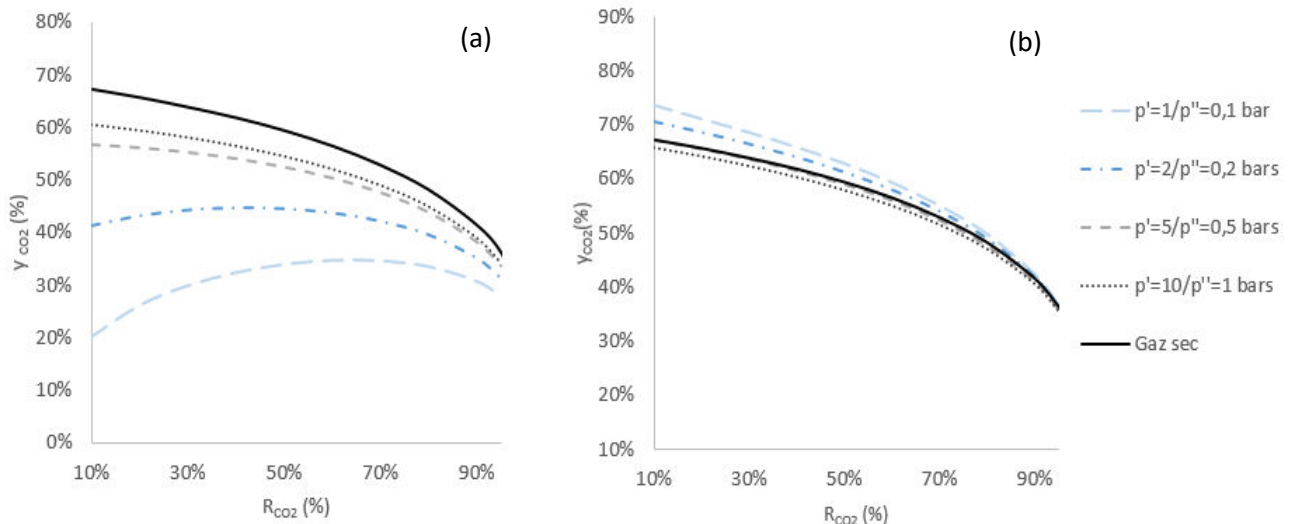
Figure 46a et 46b. Etude des courbes de pureté de la membrane Matrimid en condition sèche (trait plein) et saturée en vapeur d'eau (traits pointillés) pour un même rapport de pression ( \psi = 0,1 ) (a). Etude des courbes de pureté de la membrane Matrimid en condition humide en base sèche (b) pour un même rapport de pression ( \psi = 0,1 ).
