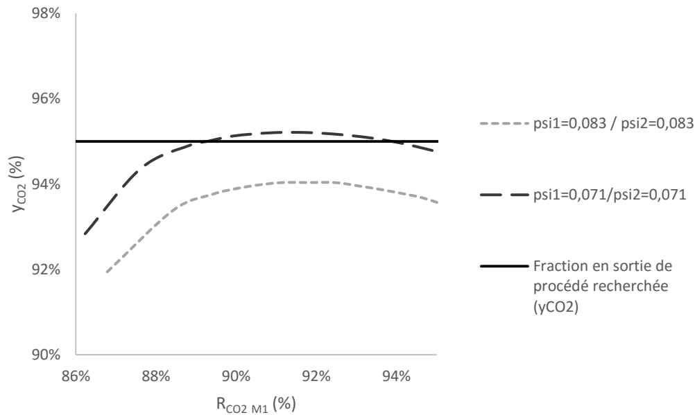
Figure 89. Détermination des rapports de pression du premier et second étage ( \psi_1 et \psi_2 ) du procédé de perméation gazeuse avec deux membranes chimiques. Le taux de capture global ( R_{CO_2} ) est fixé à 85%.
