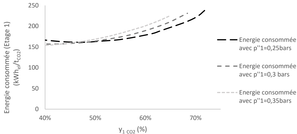
Figure 82. Evaluation de l'énergie consommée et détermination de la pression aval du premier module membranaire ( p''_1 ) pour un taux de capture en CO 2 ( R_{\text{CO}_2\text{ M1}} ) fixé à 90%.
