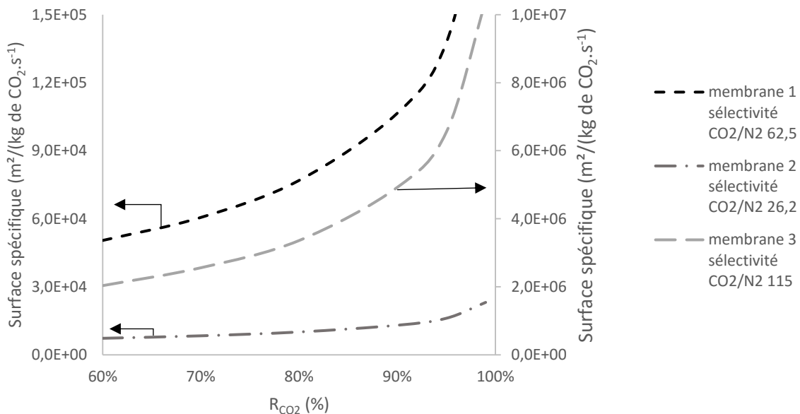
Figure 40. Estimation de la surface spécifique pour chaque membrane avec un rapport de pression égal ( \psi = 0,1 ; p' = 2 bar et p'' = 0,2 bar)
