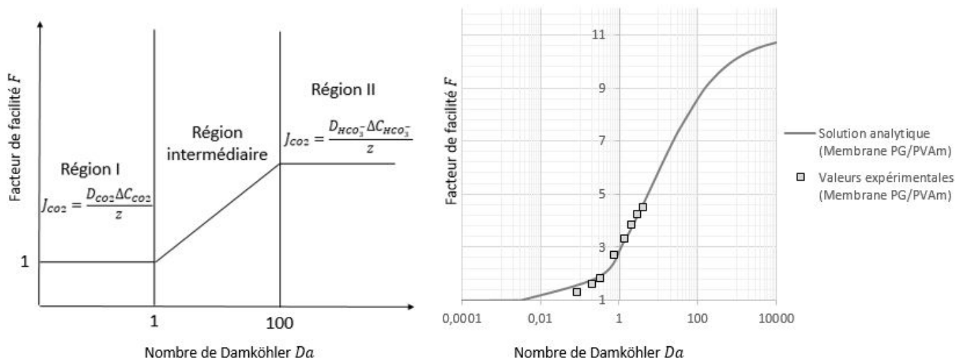
Figure 68a et 68b. Schéma de l'évolution du nombre de Damköhler dans une membrane réactive [15]. Evolution du nombre de Damköhler en fonction de l'épaisseur dans la membrane réactive PG/PVAm
