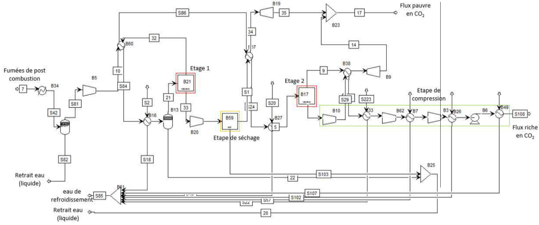
Figure 90. Schéma du procédé de perméation gazeuse à deux étages pour le captage du CO 2 en post combustion. Association d'une membrane à transport facilité
