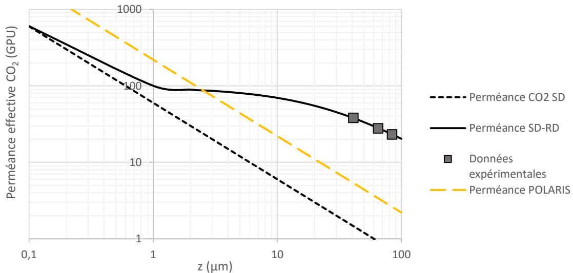
Figure 70. Evolution de la perméance effective entre une membrane PVA, une membrane POLARIS et la membrane BAM-1
