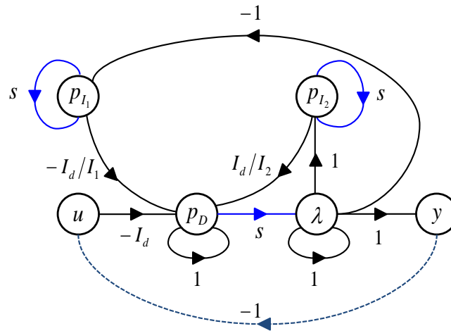
FIGURE D.7 – Digraphe du modèle de la figure D.5 en introduisant la variable d'état supplémentaire \lambda
