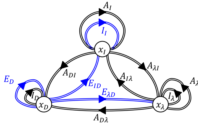
FIGURE D.2 – Remarque sur le digraphe générique obtenu à partir d'un modèle bond graph en appliquant les items 1 à 13 de la procédure D.1
