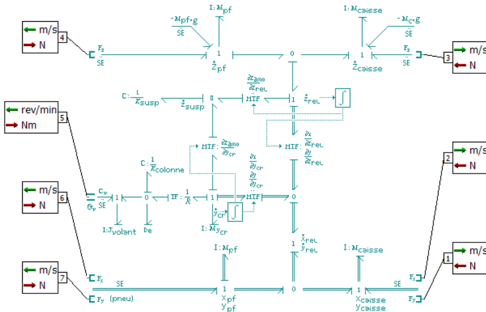
FIGURE F.5 – Implémentation du modèle multicorps quart de véhicule à 6 degrés de liberté dans le logiciel Amesim [Sie], détail de la causalité
