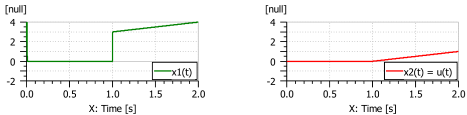
FIGURE 5.4 – Solution temporelle du système (5.41) pour l'entrée (5.47) [Dai89c]
