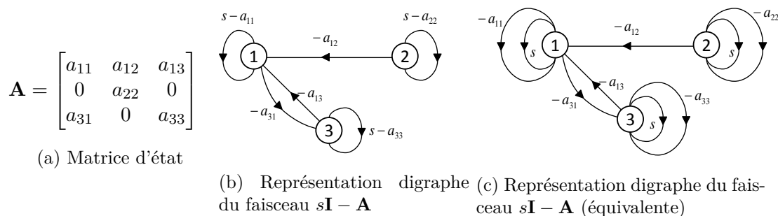
FIGURE C.3 – Exemple de représentation d'un faisceau s\mathbf{I} - \mathbf{A} pour le calcul du polynôme caractéristique par la procédure générique (théorème C.1) de calcul d'un déterminant en digraphe (le digraphe C.3c est la représentation explicitée du faisceau (s\mathbf{I} - \mathbf{A}) )
