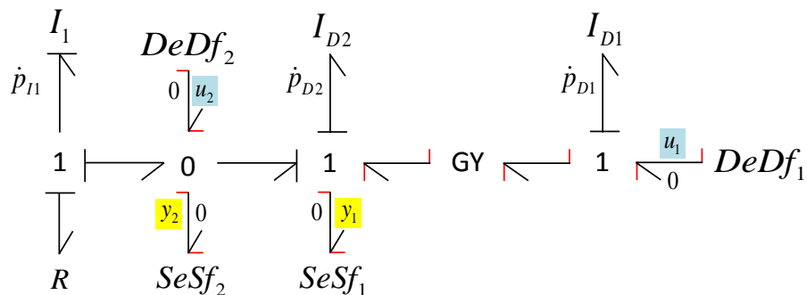
FIGURE 5.6 – Modèle bond graph comprenant un mode impulsionnel sur une variable d'énergie
