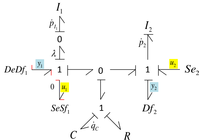
FIGURE 4.26 – Exemple d'un bond graph bicausal représentant un système direct singulier
