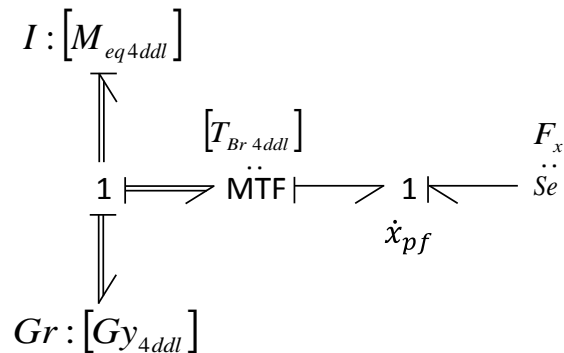
FIGURE G.8 – Transformation du bond graph de la figure G.1, septième étape (passage de l'élément inertiel dépendant I : M_{pf} à travers le MTF )
