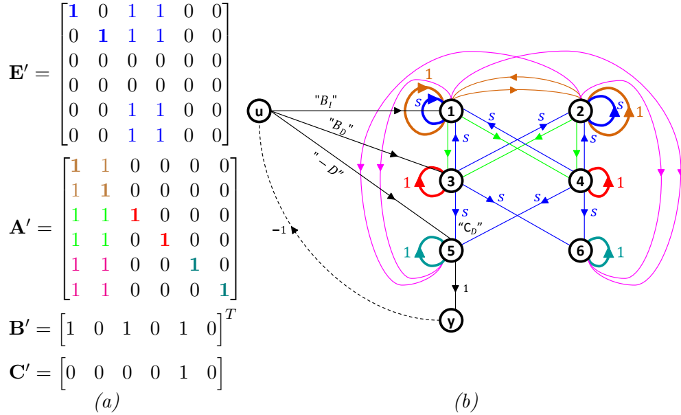
FIGURE C.11 – (a) Exemple de représentation issue de la forme (C.18) et (b) représentation digraphe associée \mathcal{G}(\Sigma'_d)
