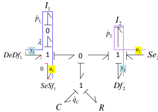
FIGURE 4.31 – Famille \mathcal{F}_{(1)}(\{u_1, u_2\}, \{y_1, y_2\}), 0 d'ordre minimal sur le bond graph 4.26
