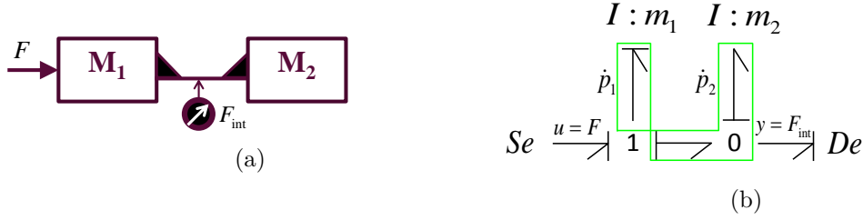
FIGURE 2.2 – Exemple de deux masses en liaison encastrement
