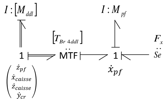
FIGURE G.7 – Transformation du bond graph de la figure G.1, sixième étape (application de la causalité)
