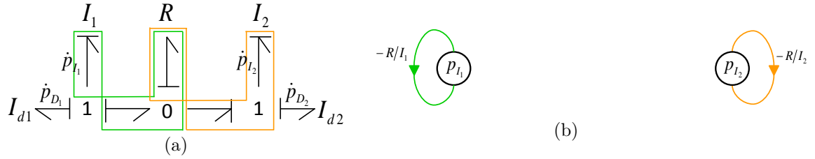
FIGURE D.11 – Exemple de correspondance entre cycles bond graph (a) et cycles digraphe (b) (sur l'exemple 1 page 311)
