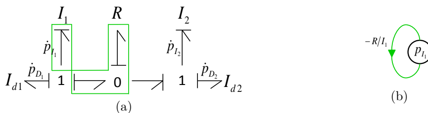
FIGURE D.10 – Exemple de correspondance entre cycle bond graph (a) et cycle digraphe (b) (sur l'exemple 1 page 311 )
