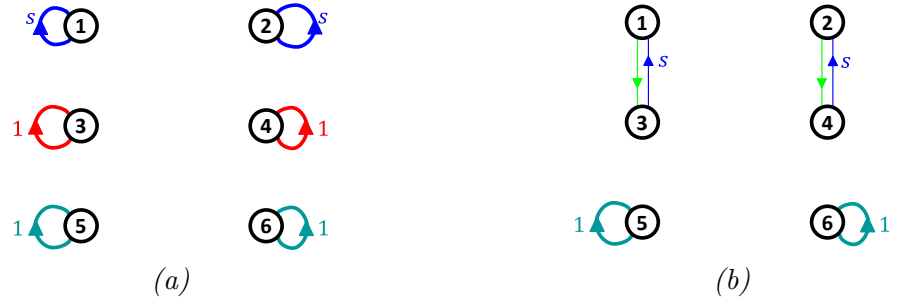
FIGURE C.10 – Exemples de familles directrices sur le digraphe \mathcal{G}(s\mathbf{E}' - \mathbf{A}') de la figure C.9 intervenant dans le calcul de \det(s\mathbf{E}' - \mathbf{A}') de (C.18)
