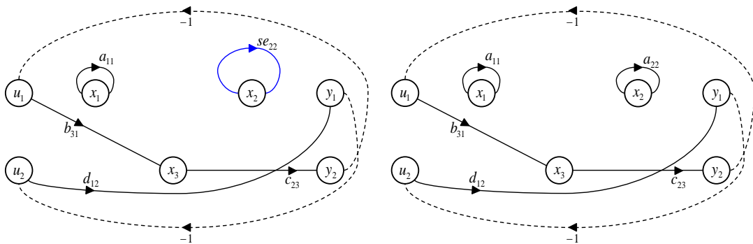
FIGURE 4.13 – Digraphe augmenté \mathcal{G}(\Sigma'_d) pour le calcul du déterminant de la matrice système (4.46)
