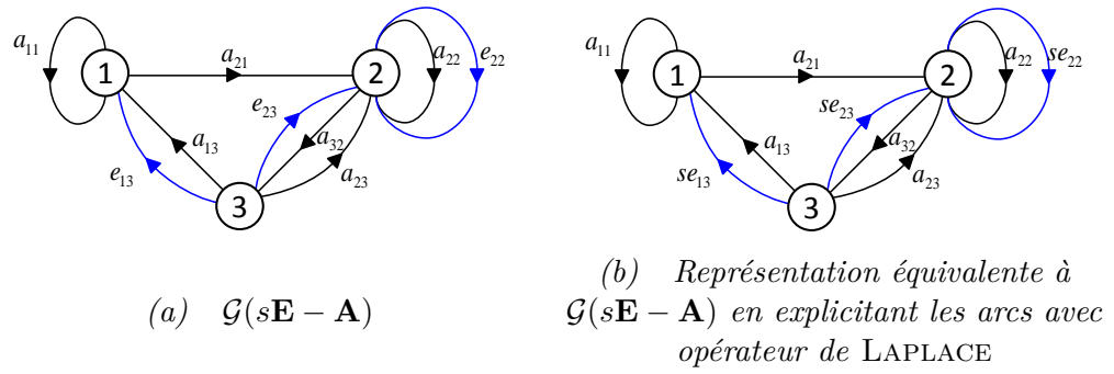
FIGURE C.5 – Représentations digraphe du système (C.12)
