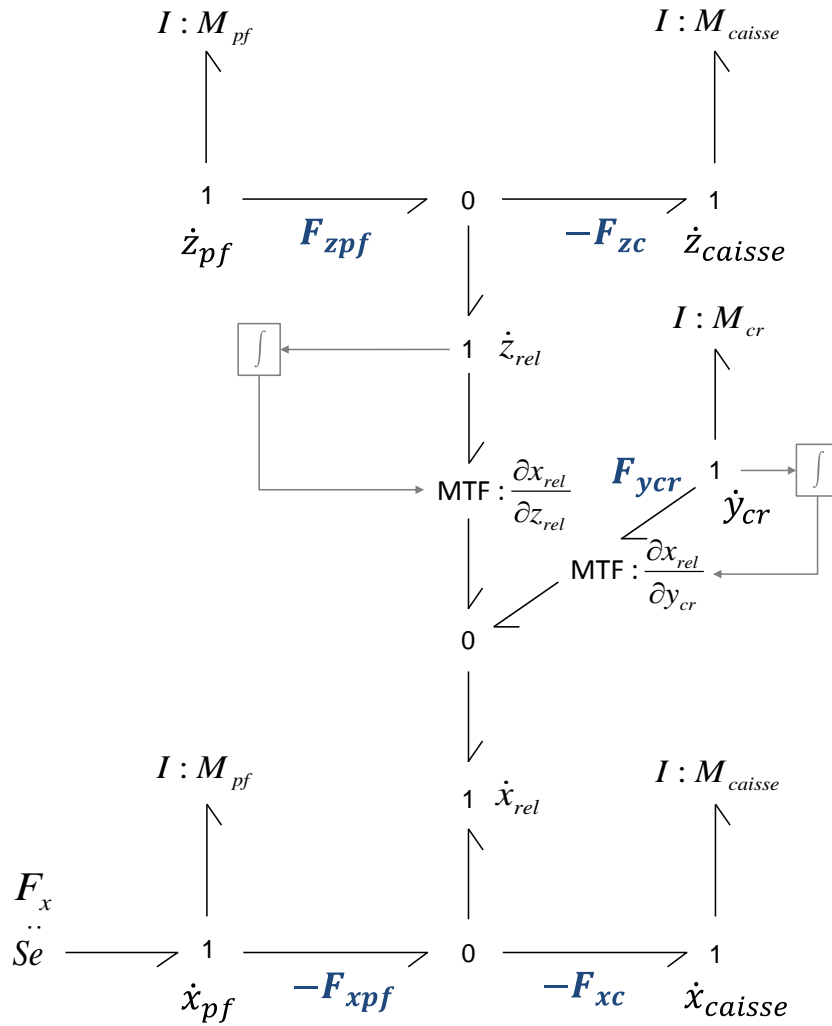
FIGURE G.1 – Représentation bond graph proposée en figure 1.9b page 18
