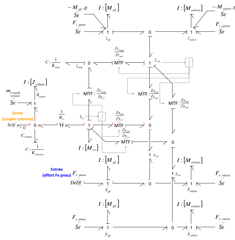
FIGURE F.9 – Modèle bicausal représentant le modèle inverse, d'ordre minimal, où la sortie est y = C_{colonne} et l'entrée est u = F_x pneu
