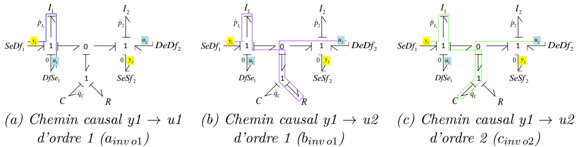
FIGURE 4.33 – Chemins causaux Sortie \rightarrow Entrée du bond graph du modèle inverse - (1 sur 4)
