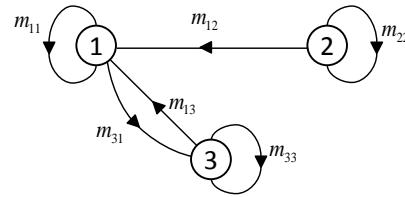
FIGURE C.1 – Calcul du déterminant de la matrice \mathbf{M} sur son digraphe associé \mathcal{G}(\mathbf{M})
