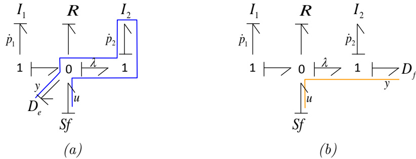
FIGURE 4.19 – Exemple de bond graph avec boucles causales d'ordre 0 et d'ordre -1
