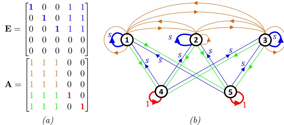
FIGURE C.7 – (a) exemple d'un faisceau (s\mathbf{E} - \mathbf{A}) issu d'un bond graph de la forme (C.13) et (b) représentation digraphe associée \mathcal{G}(s\mathbf{E} - \mathbf{A})
