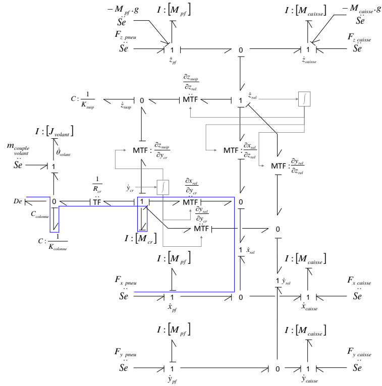
FIGURE F.8 – Chemin causal entrée/sortie a_{o2s_{iso}} , d'ordre minimal, sur le modèle direct
