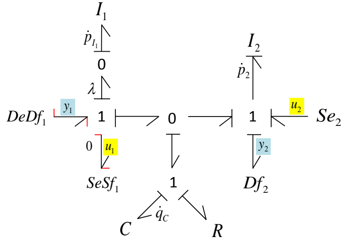
FIGURE A.8 – Système singulier représenté par un bond graph bicausale
