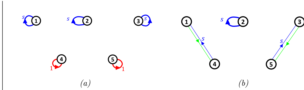
FIGURE C.8 – Exemples de familles directrices sur le digraphe \mathcal{G}(s\mathbf{E} - \mathbf{A}) de la figure C.7 pour le calcul de \det(s\mathbf{E} - \mathbf{A})
