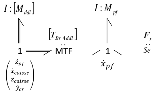
FIGURE G.6 – Transformation du bond graph de la figure G.1, cinquième étape (écriture utilisant des multi-liens)
