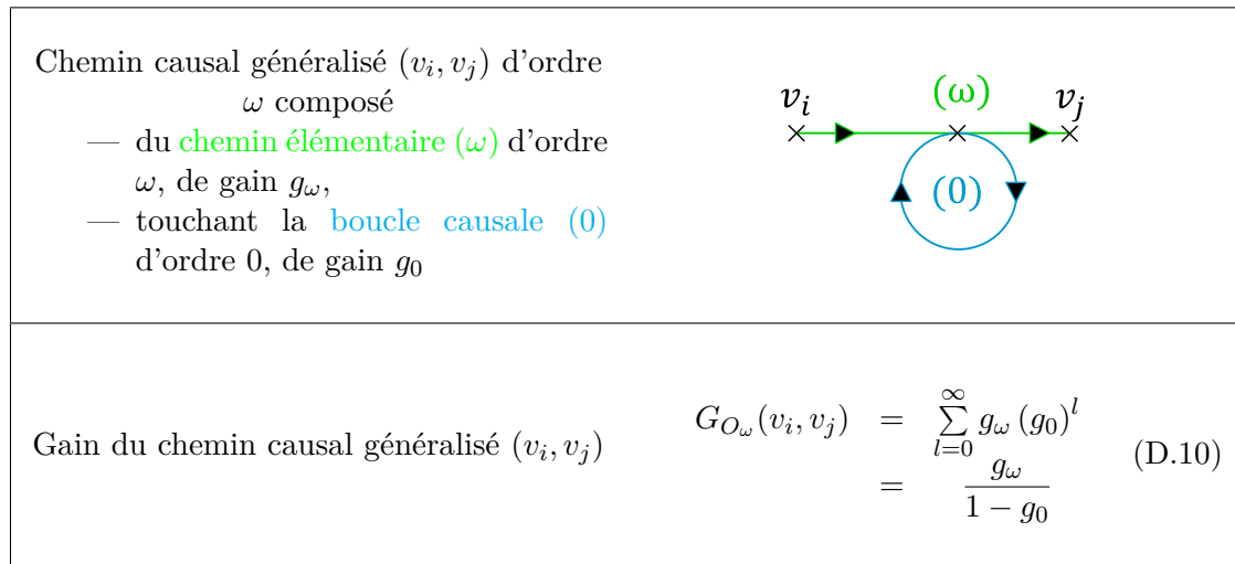
FIGURE D.9 – Détail du gain du chemin causal généralisé (v_i, v_j) , utilisant le graphe des chemins causaux [Mas88] [FN97]
