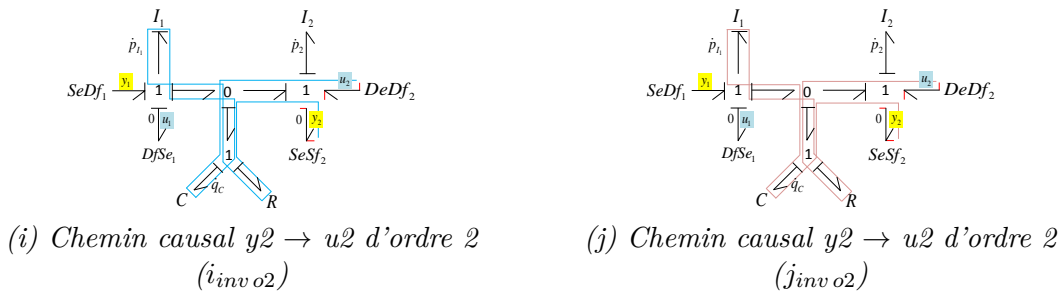
FIGURE 4.36 – Chemins causaux Sortie \rightarrow Entrée du bond graph du modèle inverse - (4 sur 4)
