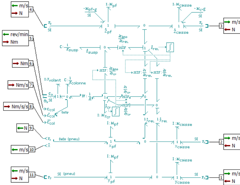
FIGURE F.13 – Implémentation du modèle multicorps quart de véhicule inverse dans le logiciel Amesim [Sie]
