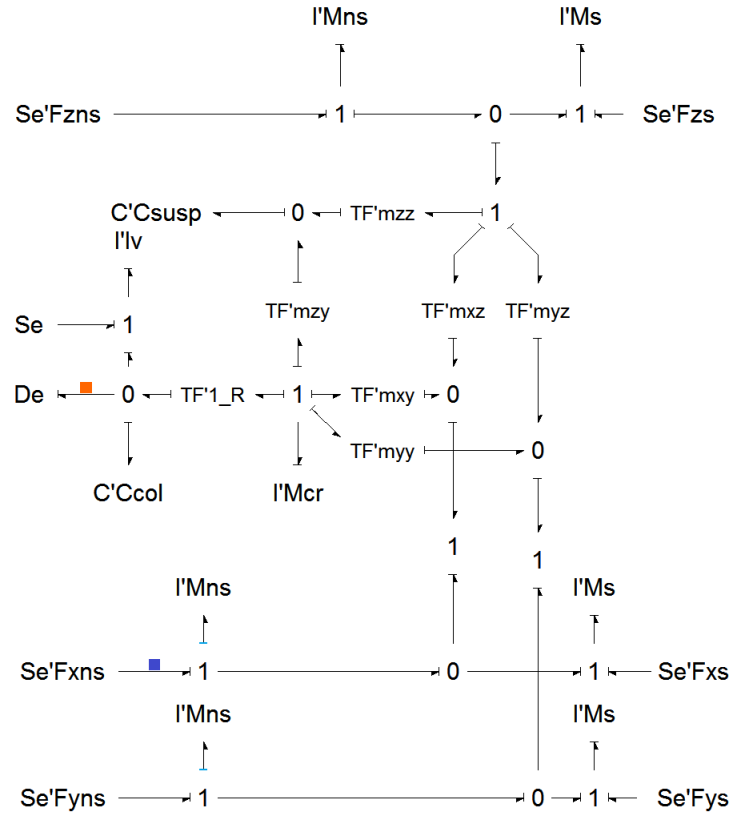
FIGURE F.4 – Implémentation du modèle multicorps linéarisé quart de véhicule à 6 degrés de liberté dans le logiciel MS1 [MS1]
