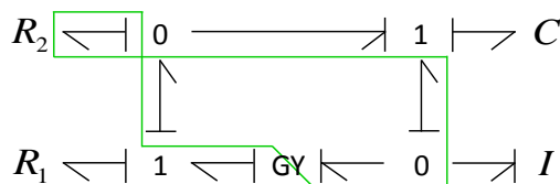
FIGURE A.3 – Boucle causale d'ordre 0 de classe 3 dans la classification de VAN DIJK [vD94]
