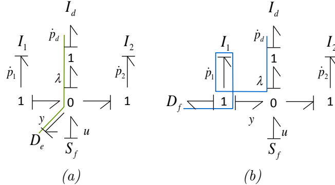
FIGURE 5.5 – Exemple de bond graph avec plusieurs boucles causales d'ordre 0 de classe 1
