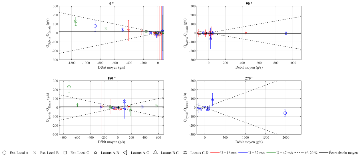
FIGURE V.23 – Écart entre les débits de fuite mesurés et calculés avec le code SYLVIA pour le réseau de ventilation à l'arrêt (70 kW injectés dans le local A)
