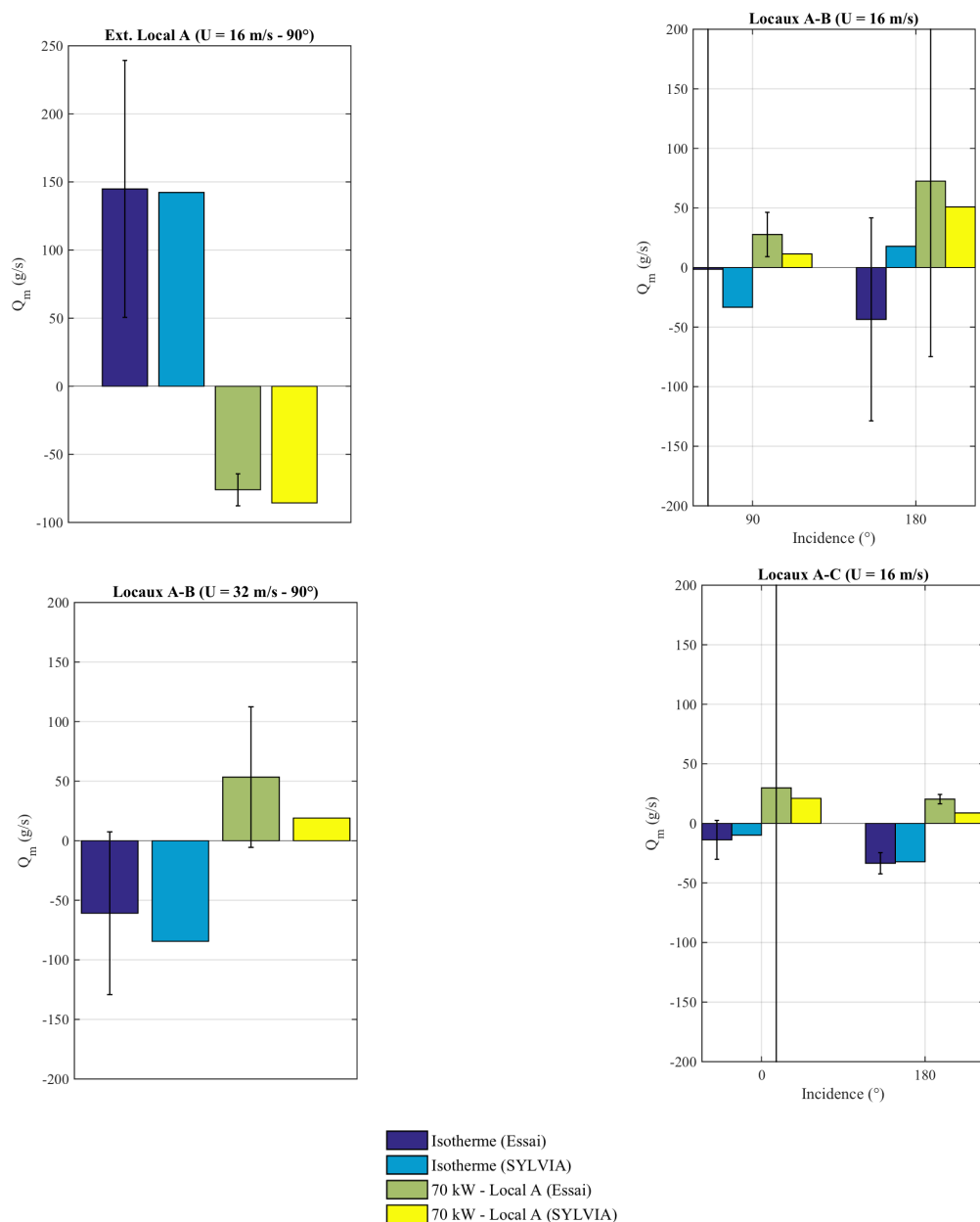
FIGURE V.32 – Valeur des débits de fuite pour la configuration isotherme et en présence d'une puissance thermique de 70 kW injectée dans le local A avec le réseau de ventilation à l'arrêt
