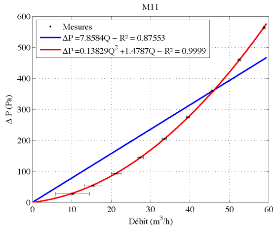
FIGURE C.9 – Loi débit-pressure du filtre d'extraction du local C
