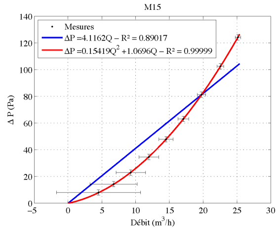
FIGURE C.10 – Loi débit-pressure du filtre d'extraction du local D
