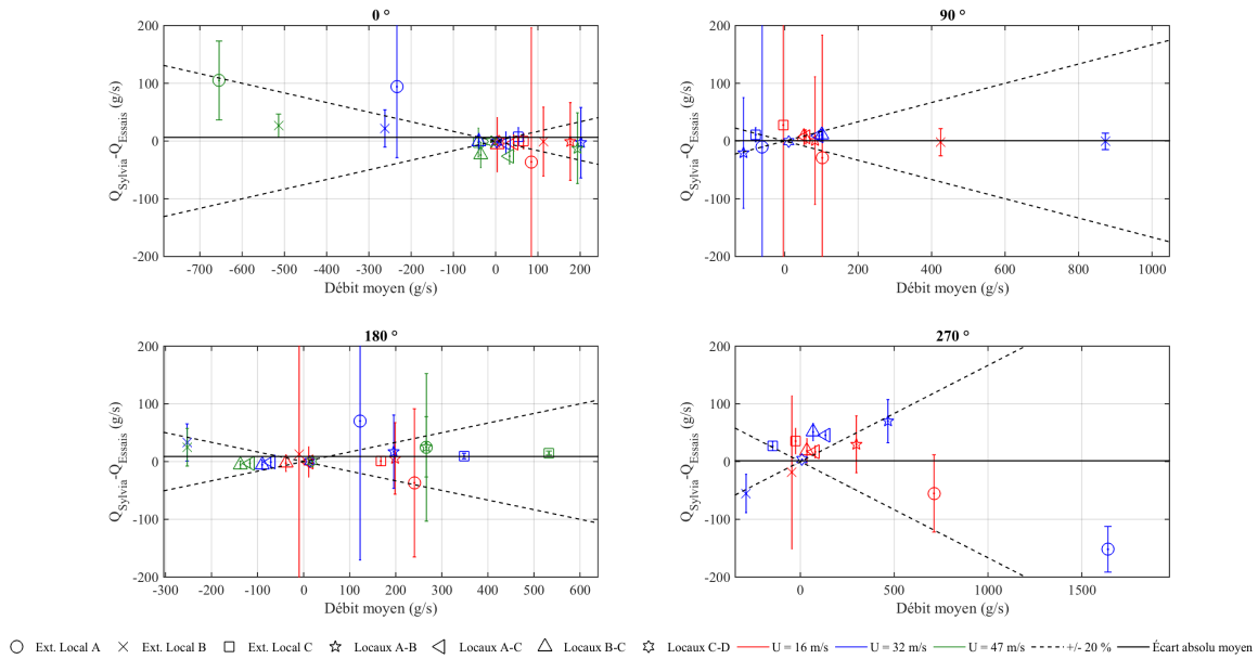
FIGURE D.15 – Écart entre les débits de fuite mesurés et calculés avec le code SYLVIA pour le réseau de ventilation en fonctionnement (24 kW injectés dans le local C)
