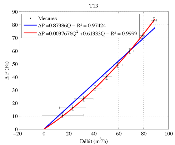
FIGURE C.12 – Loi débit-pressure du filtre d'extraction procédé
