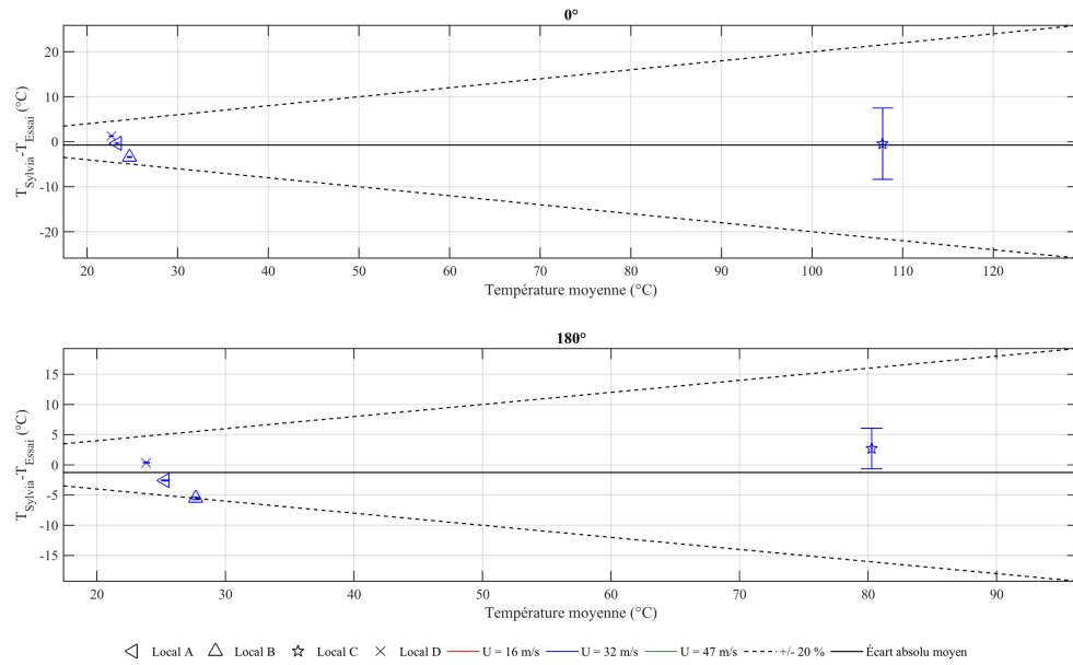
FIGURE D.20 – Écart entre les températures intérieures des locaux mesurées et calculées avec le code SYLVIA pour le réseau de ventilation en fonctionnement (60 kW injectés dans le local C)
