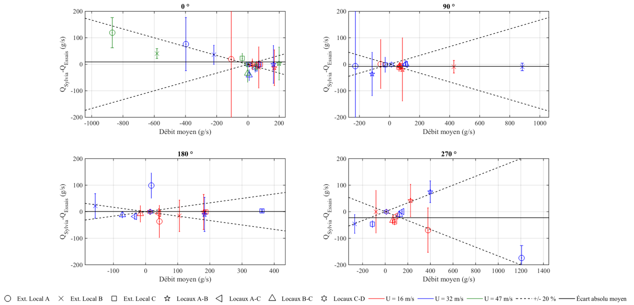
FIGURE V.18 – Écart entre les débits de fuite mesurés et calculés avec le code SYLVIA pour le réseau de ventilation en fonctionnement (70 kW injectés dans le local A)
