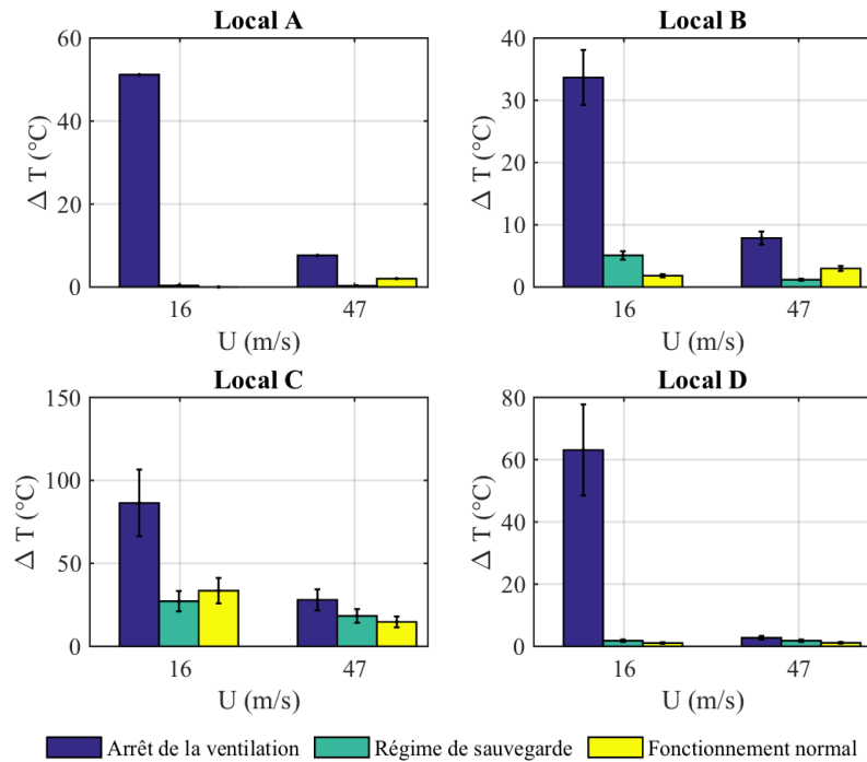
FIGURE IV.29 – Variation de température dans les locaux pour une puissance thermique de 24 kW injectée dans le local C et une incidence du vent de 0°
