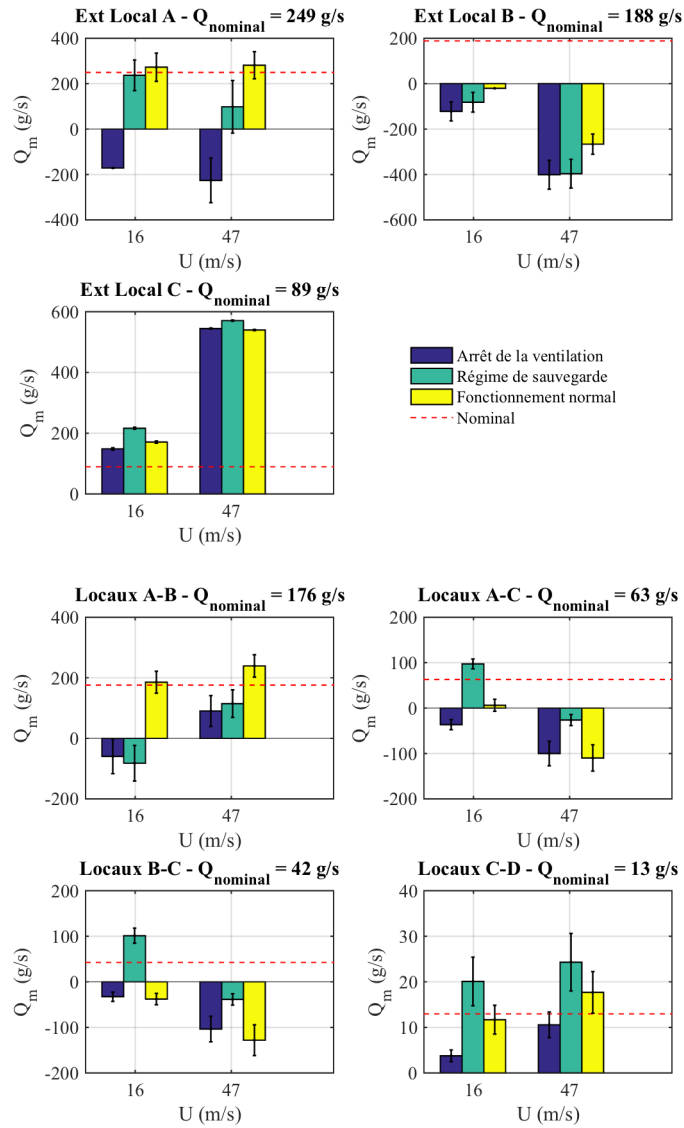
FIGURE B.6 – Valeur des débits de fuite pour une puissance thermique de 24 kW injectée dans le local C et une incidence du vent de 180^\circ
