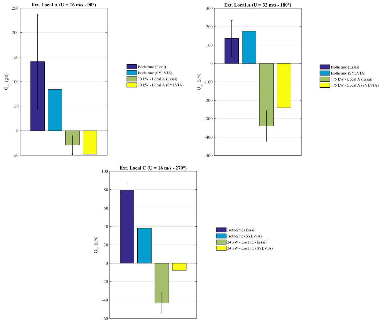
FIGURE V.31 – Valeur des débits de fuite avec inversion du sens d’écoulement pour la configuration isotherme et en présence d’une puissance thermique injectée dans le local A ou dans le local C avec le réseau de ventilation en fonctionnement
