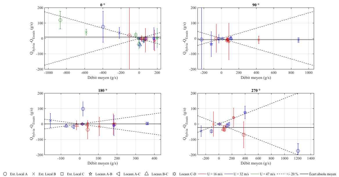
FIGURE D.5 – Écart entre les débits de fuite mesurés et calculés avec le code SYLVIA pour le réseau de ventilation en fonctionnement (70 kW injectés dans le local A)
