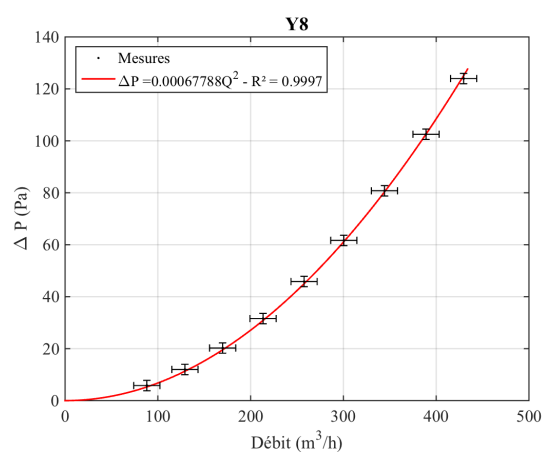
FIGURE C.30 – Cheminée d'extraction
