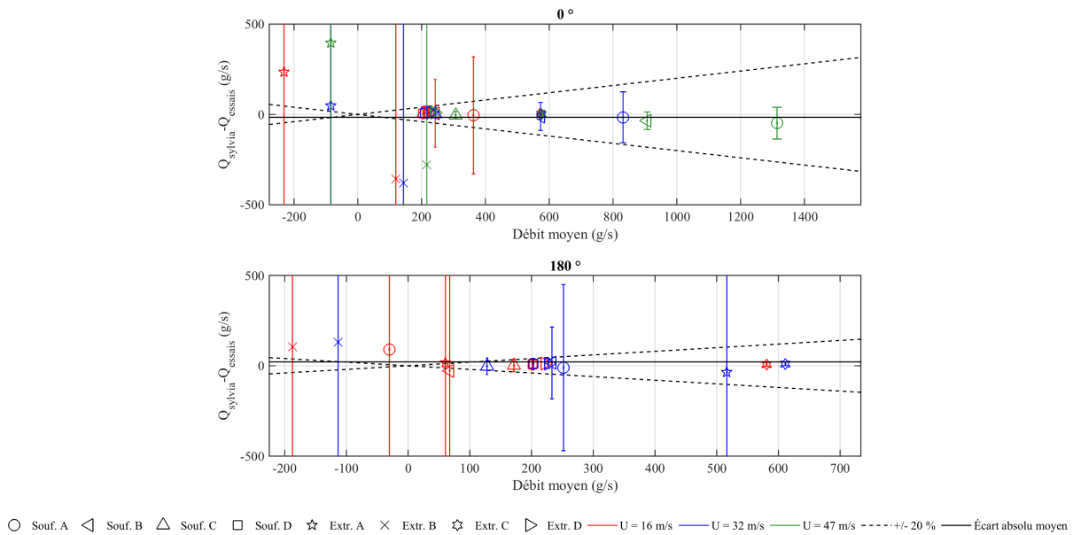
FIGURE V.15 – Écart entre les débits de ventilation mesurés et calculés avec le code SYLVIA pour le réseau de ventilation en régime de sauvegarde (configuration isotherme)
