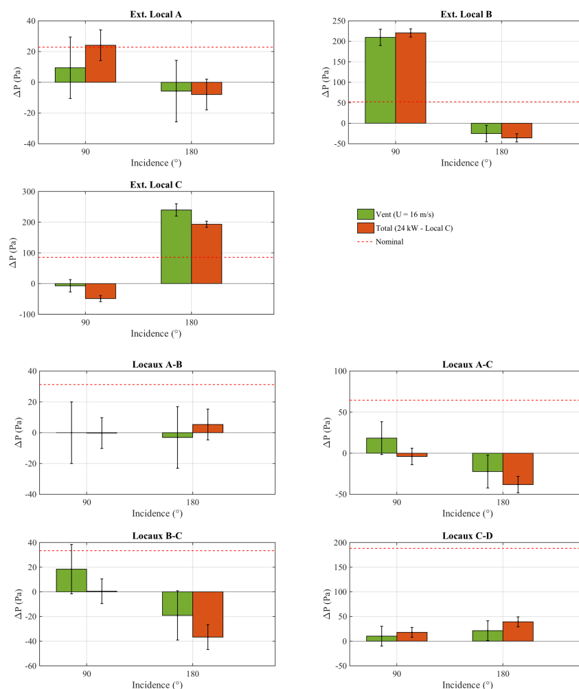
FIGURE IV.19 – Valeur des différences de pression au niveau des fuites pour une puissance thermique de 24 kW injectée dans le local C et le réseau de ventilation à l'arrêt
