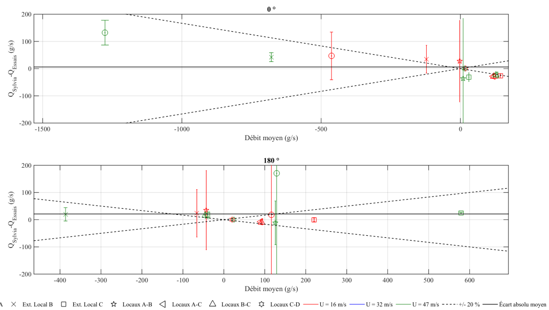
FIGURE D.38 – Écart entre les débits de fuite mesurés et calculés avec le code SYLVIA pour le réseau de ventilation en régime de sauvegarde (24 kW injectés dans le local C)
