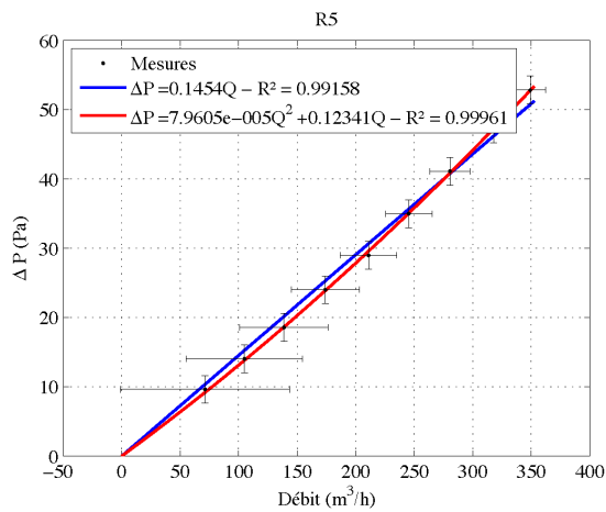
FIGURE C.11 – Loi débit-pressure du filtre d'extraction d'ambiance
