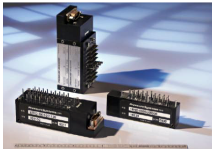
FIGURE III.7 – Capteurs de pression PSI permettant une mesure synchrone de 32 voies de pression à une fréquence d'acquisition de 200 Hz.
