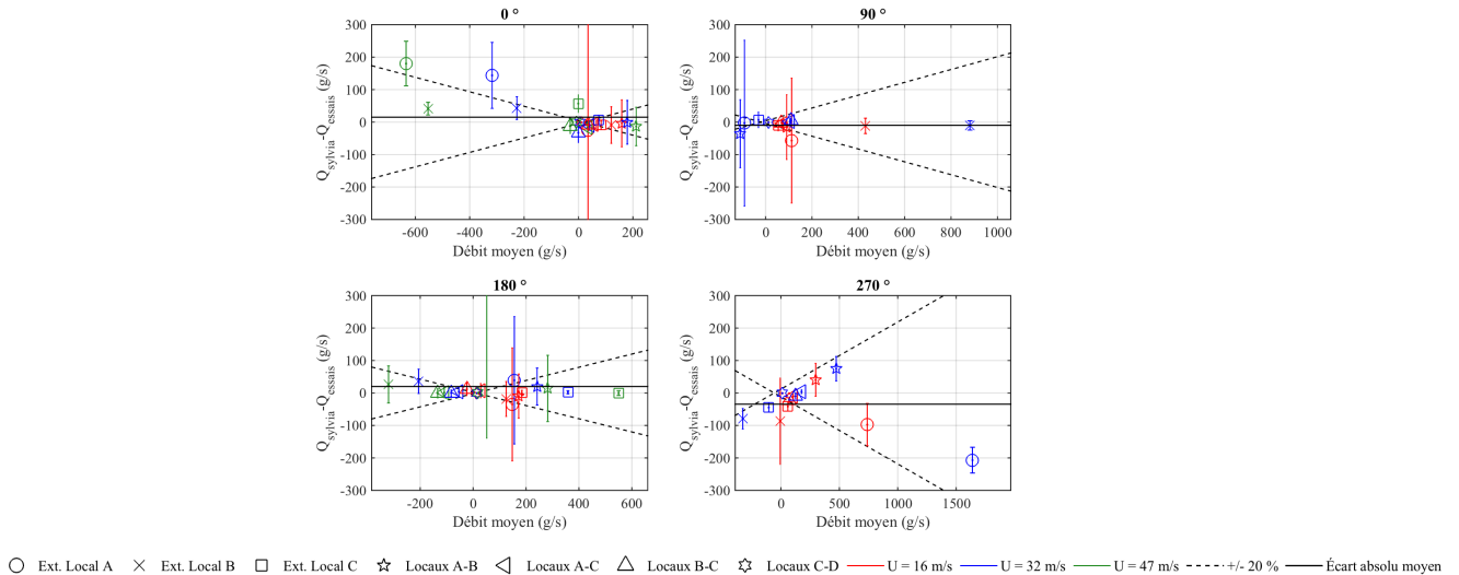
FIGURE V.5 – Écart entre les débits de fuite mesurés et calculés avec le code SYLVIA pour le réseau de ventilation en fonctionnement (configuration isotherme)
