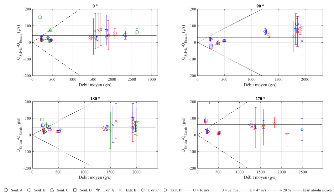
FIGURE D.17 – Écart entre les débits de ventilation mesurés et calculés avec le code SYLVIA pour le réseau de ventilation en régime en fonctionnement (24 kW injectés dans le local C)
