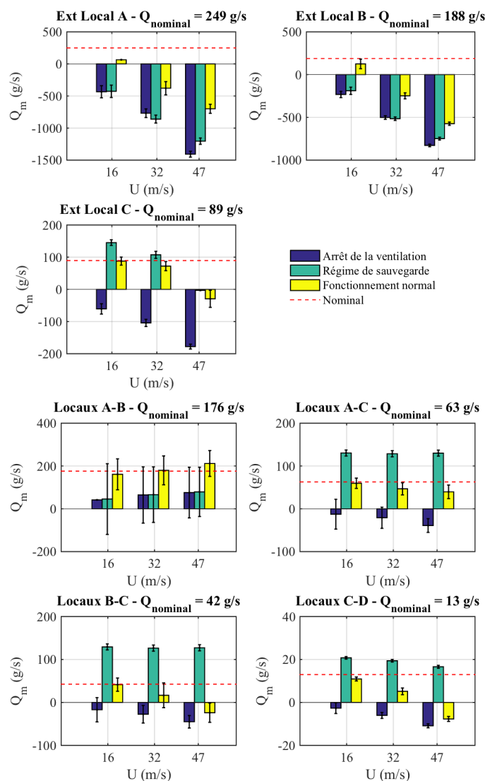
FIGURE IV.7 – Valeur des débits de fuite pour la configuration isotherme (sans source de chaleur) et une incidence du vent de 0^\circ
