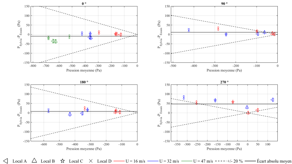
FIGURE V.17 – Écart entre les pressions intérieures des locaux mesurées et calculées avec le code SYLVIA pour le réseau de ventilation en fonctionnement (70 kW injectés dans le local A)
