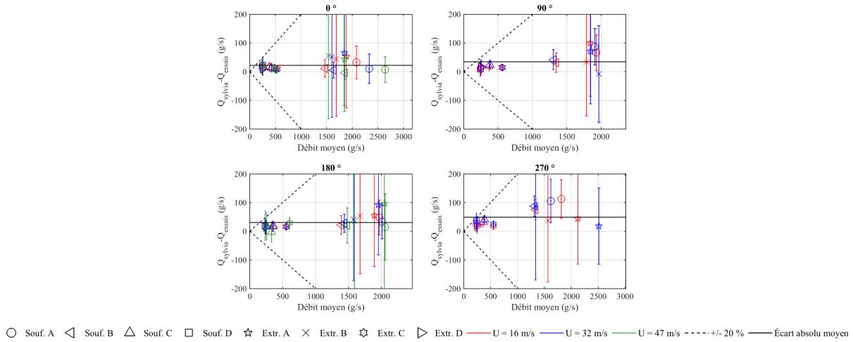
FIGURE V.7 – Écart entre les débits de ventilation mesurés et calculés avec le code SYLVIA pour le réseau de ventilation en fonctionnement (configuration isotherme)
