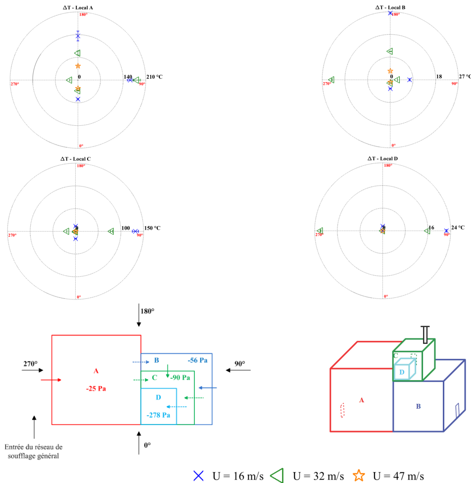
FIGURE IV.18 – Variation de température dans les locaux pour une puissance thermique de 70 kW injectée dans le local A et le réseau de ventilation à l'arrêt
