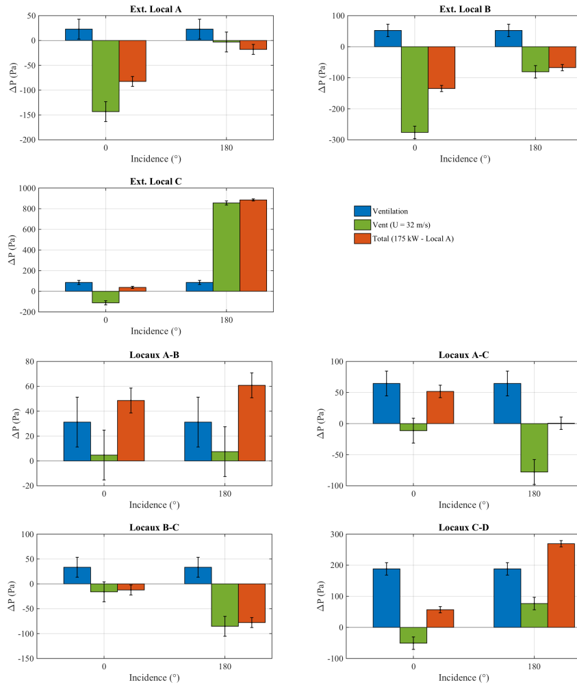
FIGURE IV.11 – Valeur des différences de pression au niveau des fuites pour une puissance thermique de 175 kW injectées dans le local A et une vitesse de vent de 32 m/s
