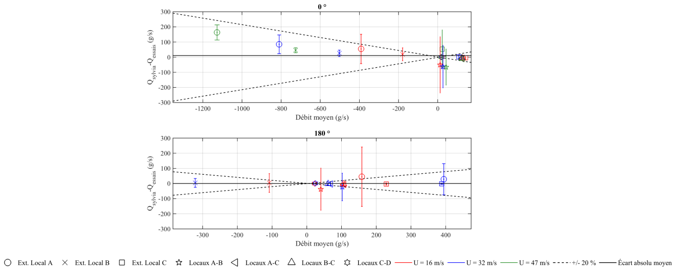
FIGURE V.14 – Écart entre les débits de fuite mesurés et calculés avec le code SYLVIA pour le réseau de ventilation en régime de sauvegarde (configuration isotherme)
