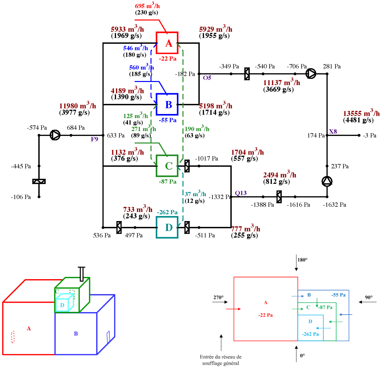
FIGURE V.2 – Configuration numérique nominale de la maquette obtenue avec le code SYLVIA
