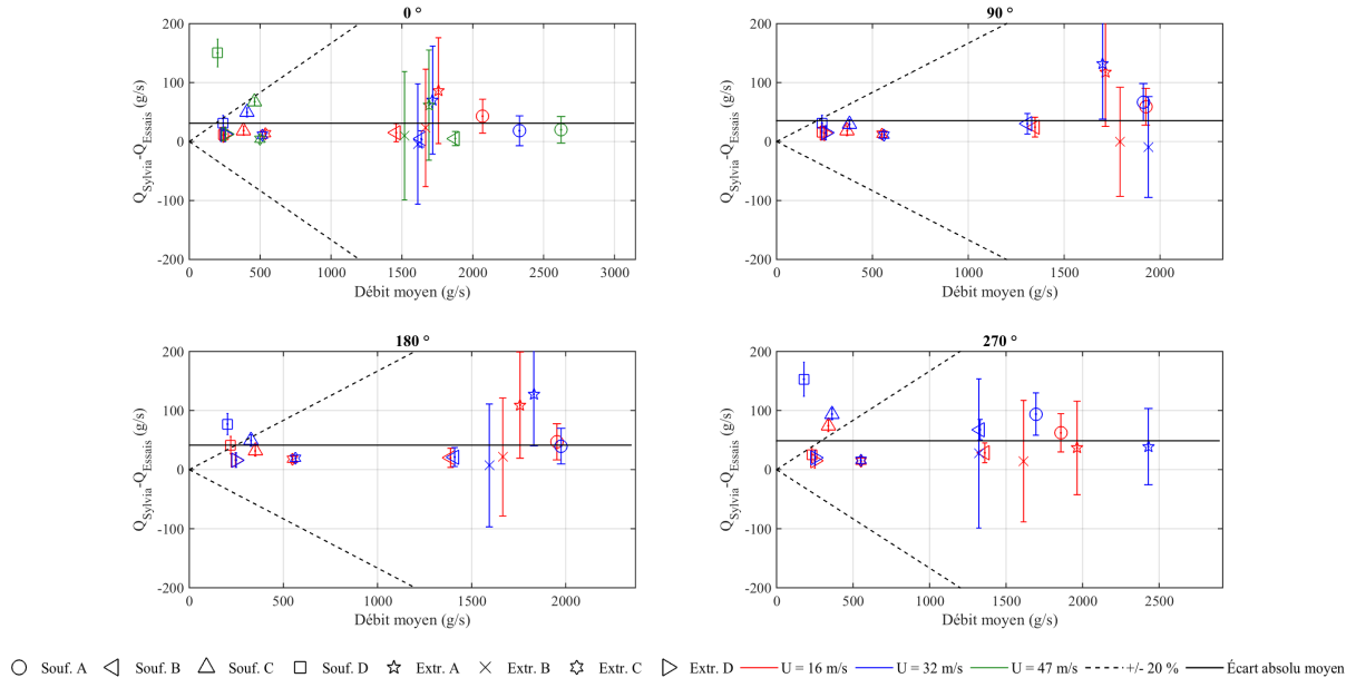
FIGURE V.19 – Écart entre les débits de ventilation mesurés et calculés avec le code SYLVIA pour le réseau de ventilation en fonctionnement (70 kW injectés dans le local A)
