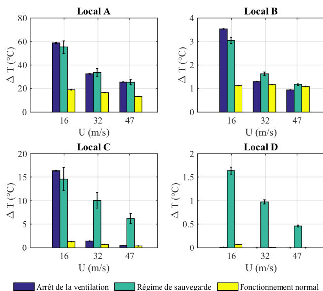
FIGURE B.4 – Variation de température dans les locaux pour une puissance thermique de 70 kW injectée dans le local A et une incidence du vent de 0^{\circ}
