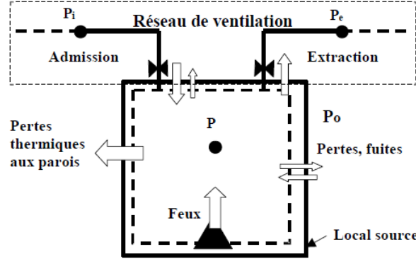
FIGURE I.5 – Flux pris en compte dans la modélisation d'un incendie dans un local confiné et ventilé mécaniquement (Prétre et al., 2012)
