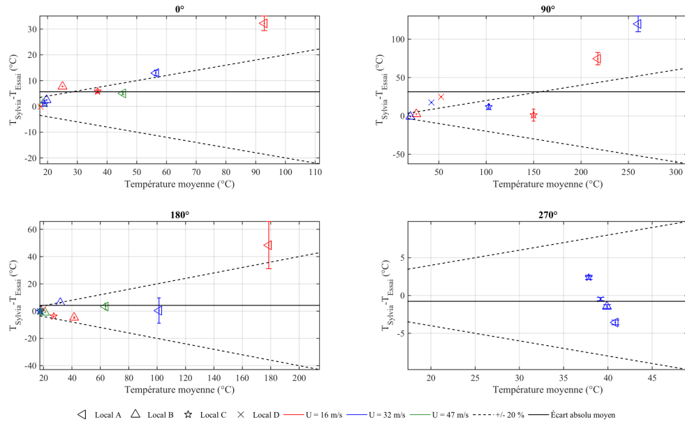
FIGURE D.25 – Écart entre les températures intérieures des locaux mesurées et calculées avec le code SYLVIA pour le réseau de ventilation à l'arrêt (70 kW injectés dans le local A)
