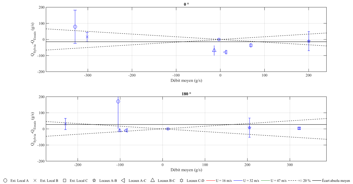
FIGURE D.16 – Écart entre les débits de fuite mesurés et calculés avec le code SYLVIA pour le réseau de ventilation en fonctionnement (60 kW injectés dans le local C)
