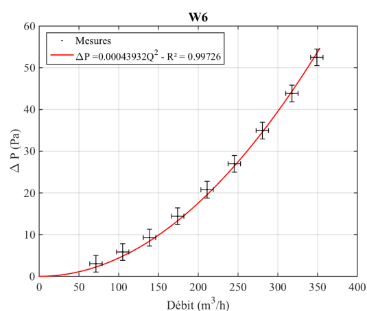
FIGURE C.28 – Aval du ventilateur d'extraction d'ambiance
