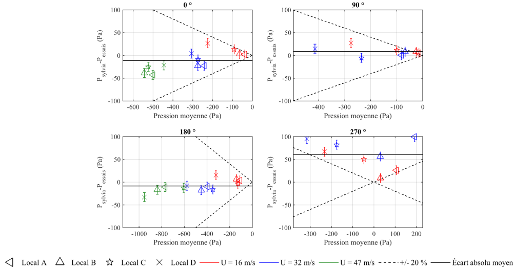
FIGURE V.4 – Écart entre les pressions intérieures des locaux mesurées et calculées avec le code SYLVIA pour le réseau de ventilation en fonctionnement (configuration isotherme)
