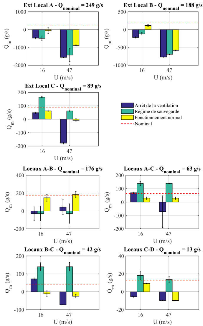
FIGURE B.5 – Valeur des débits de fuite pour une puissance thermique de 24 kW injectée dans le local C et une incidence du vent de 0^\circ
