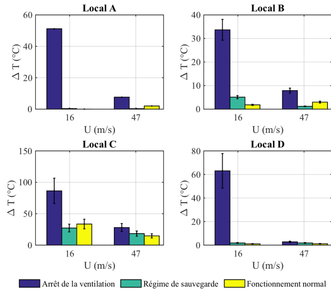
FIGURE B.7 – Variation de température dans les locaux pour une puissance thermique de 24 kW injectée dans le local C et une incidence du vent de 0°
