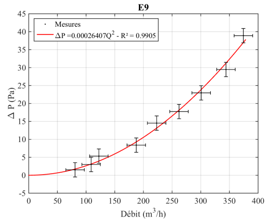
FIGURE C.14 – Soufflage général
