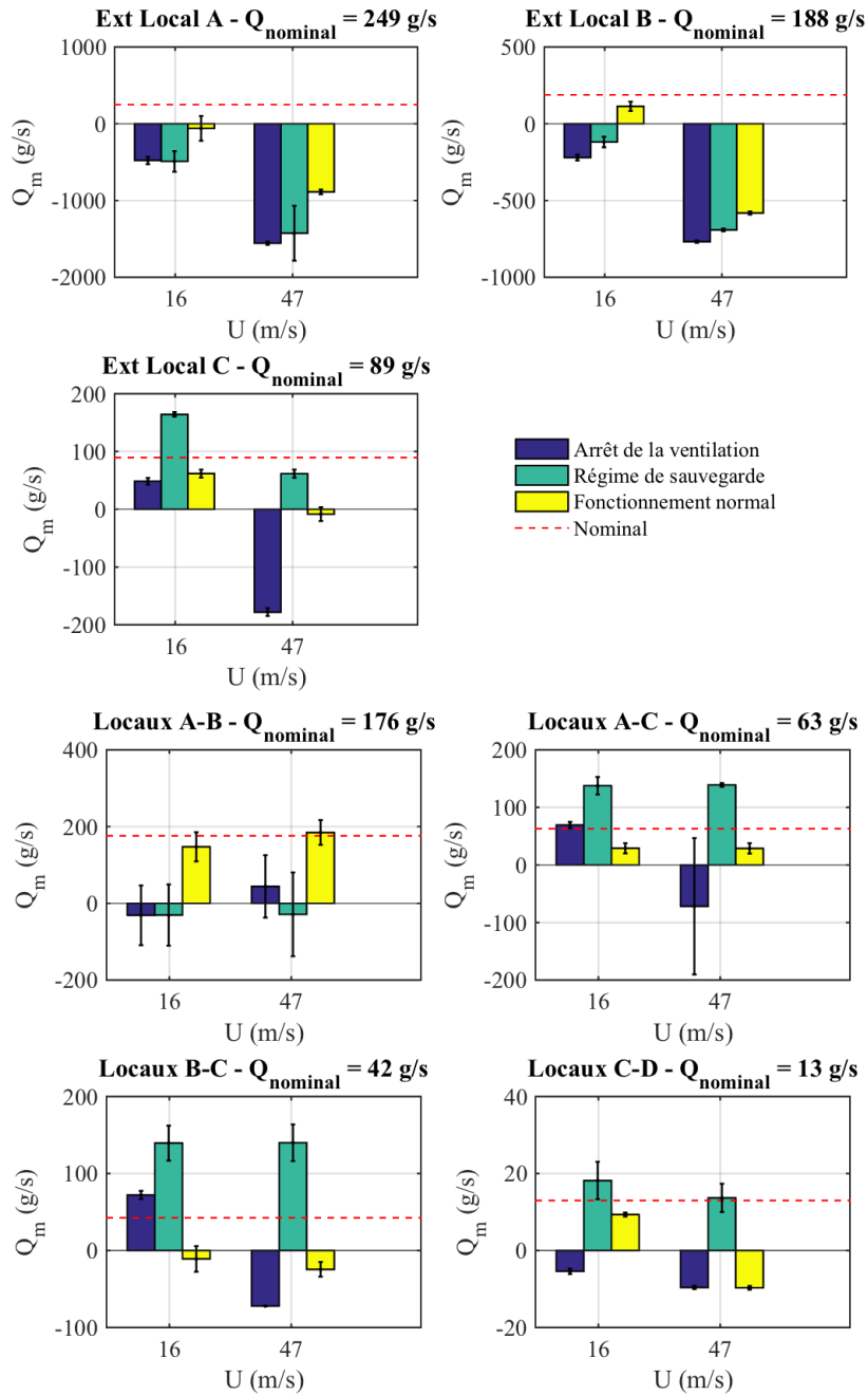
FIGURE IV.28 – Valeur des débits de fuite pour une puissance thermique de 24 kW injectée dans le local C et une incidence du vent de 0^\circ
