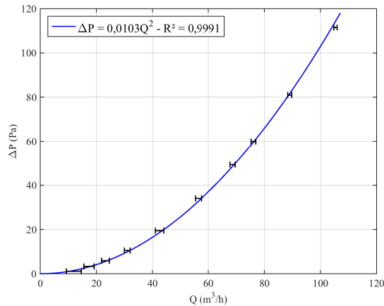
FIGURE III.17 – Loi débit-pression expérimentale des pertes de charge du ventilateur à l’arrêt
