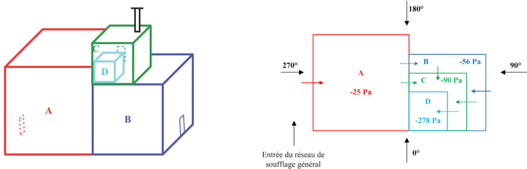
FIGURE E.2 – Configuration avec le réseau de ventilation en régime de sauvegarde pour une puissance thermique de 70 kW injectée dans le local A, une incidence du vent de 180° et une vitesse du vent de 32 m/s
