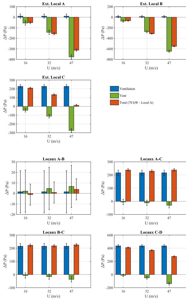
FIGURE IV.22 – Valeur des différences de pression au niveau des fuites pour une puissance thermique de 70 kW injectée dans le local A et une incidence du vent de 0°
