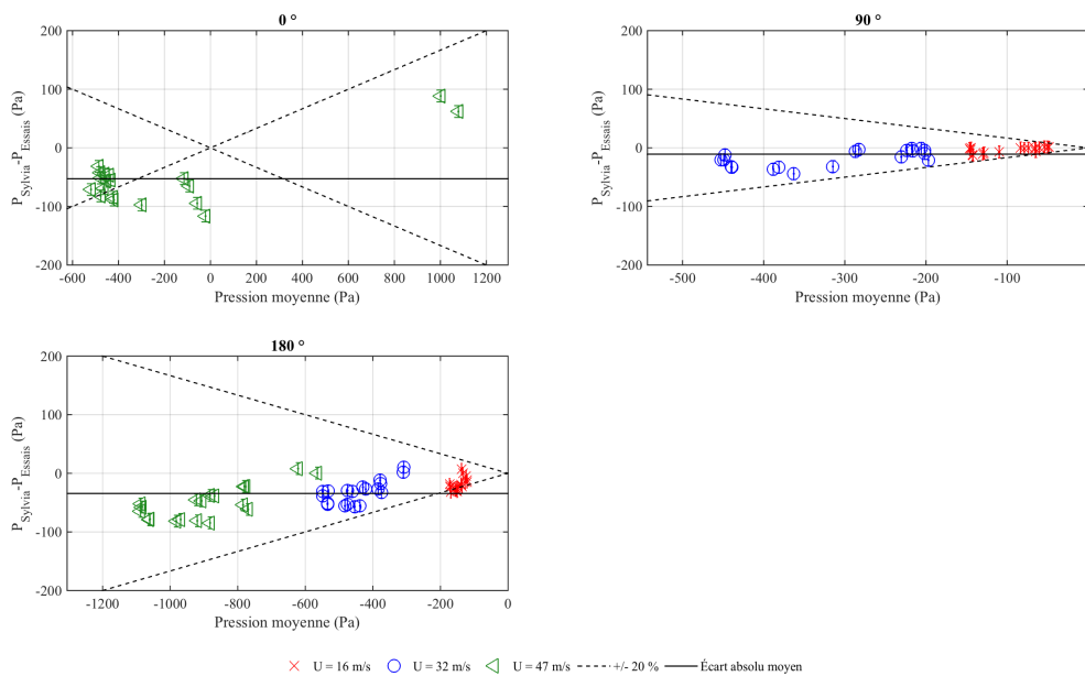
FIGURE D.26 – Écart entre les pressions aux nœuds du réseau de ventilation mesurées et calculées avec le code SYLVIA pour le réseau de ventilation à l'arrêt (24 kW injectés dans le local C)
