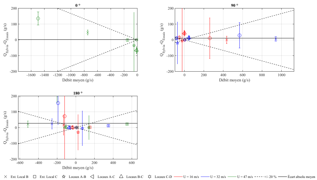
FIGURE D.28 – Écart entre les débits de fuite mesurés et calculés avec le code SYLVIA pour le réseau de ventilation à l'arrêt (24 kW injectés dans le local C)
