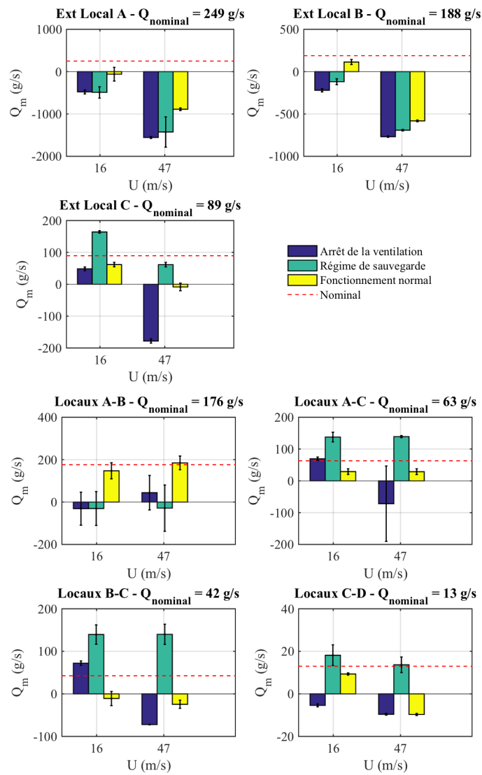
FIGURE B.5 – Valeur des débits de fuite pour une puissance thermique de 24 kW injectée dans le local C et une incidence du vent de 0°
