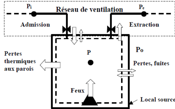
FIGURE I.5 – Flux pris en compte dans la modélisation d'un incendie dans un local confiné et ventilé mécaniquement (Prétrell et al. , 2012)
