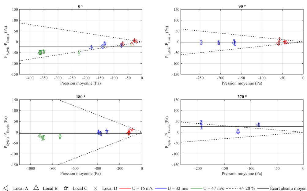
FIGURE V.22 – Écart entre les pressions intérieures des locaux mesurées et calculées avec le code SYLVIA pour le réseau de ventilation à l'arrêt (70 kW injectés dans le local A)
