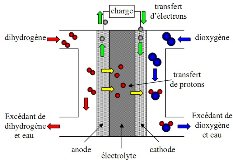
FIGURE 1.4: Principe de fonctionnement d'une PEMFC
