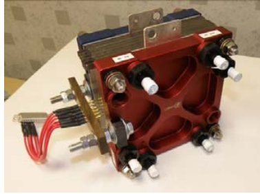
FIGURE 3.7: Stack cinq cellules BZ100 de UBzM
