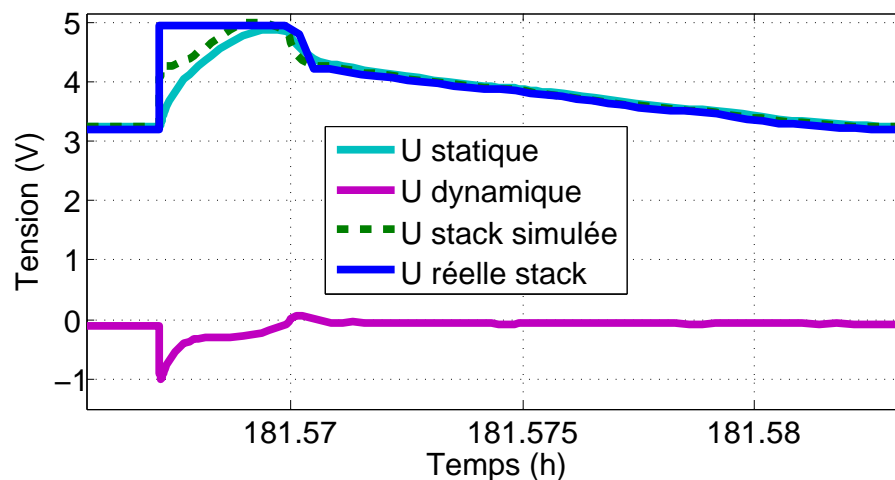
FIGURE 3.10: Tensions statique et dynamique simulées
