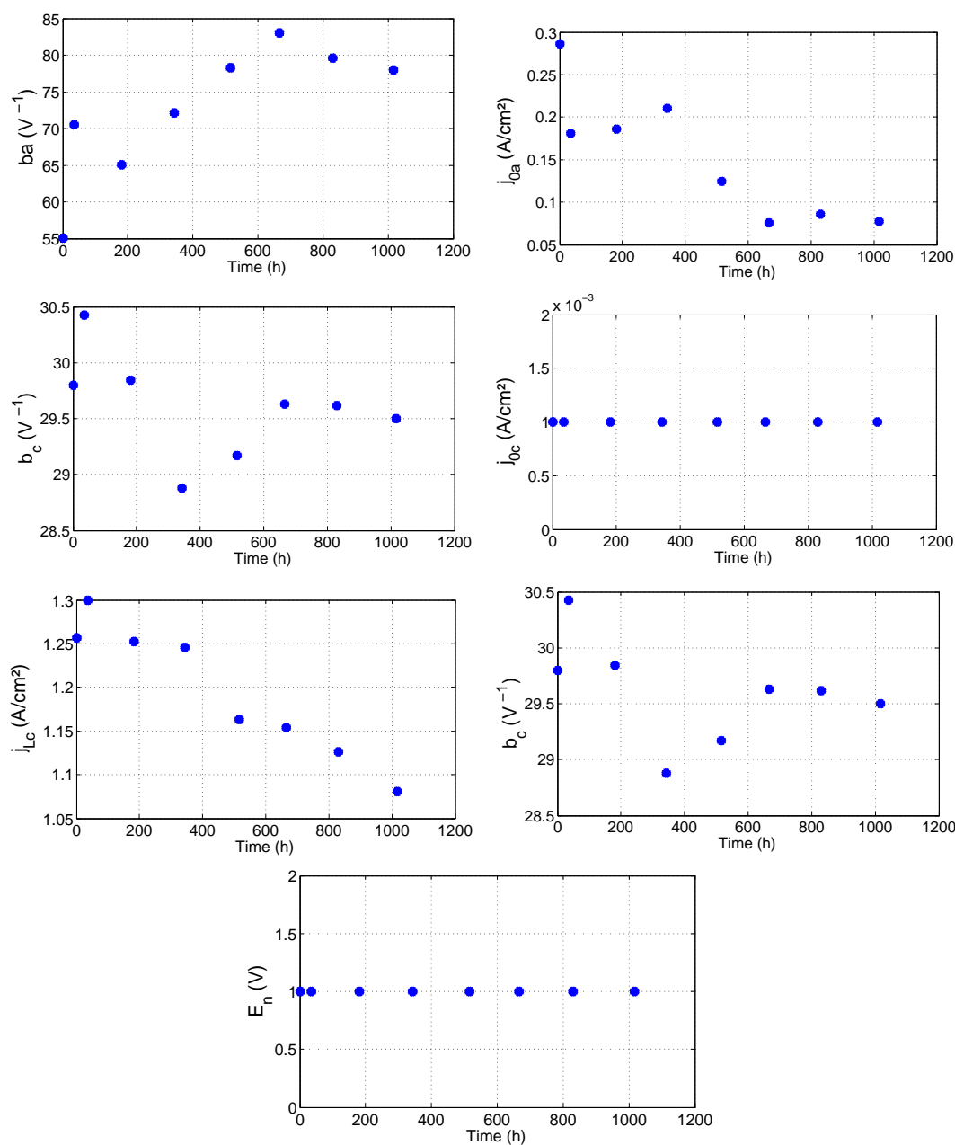
FIGURE 3.3: Évolution temporelle des valeurs atteintes par les paramètres statiques
