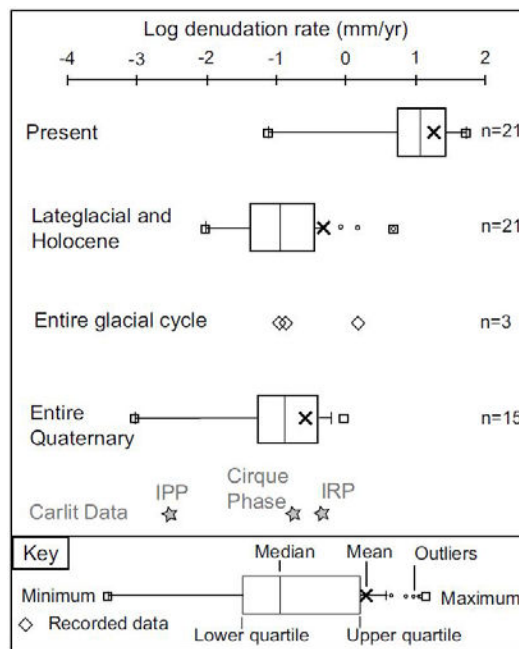
Figure 1.13. Taux mondiaux de dénudation de glaciers en fonction de l'intervalle de temps considéré [extrait de Delmas et al., 2009]. Les taux de dénudation sont obtenus à partir de la mesure des volumes sédimentaires accumulés aux marges et à l'exutoire des glaciers (IPP : ice progression phase ; IRP : ice recession phase ).
