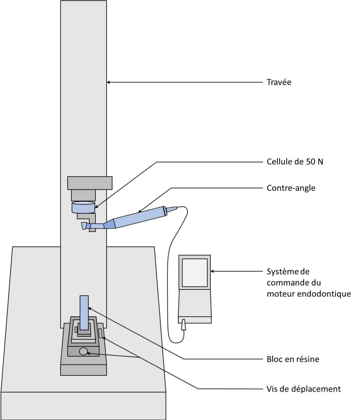
Figure 3.1. Schéma du banc d'essais servant aux manipulations en P/R.
