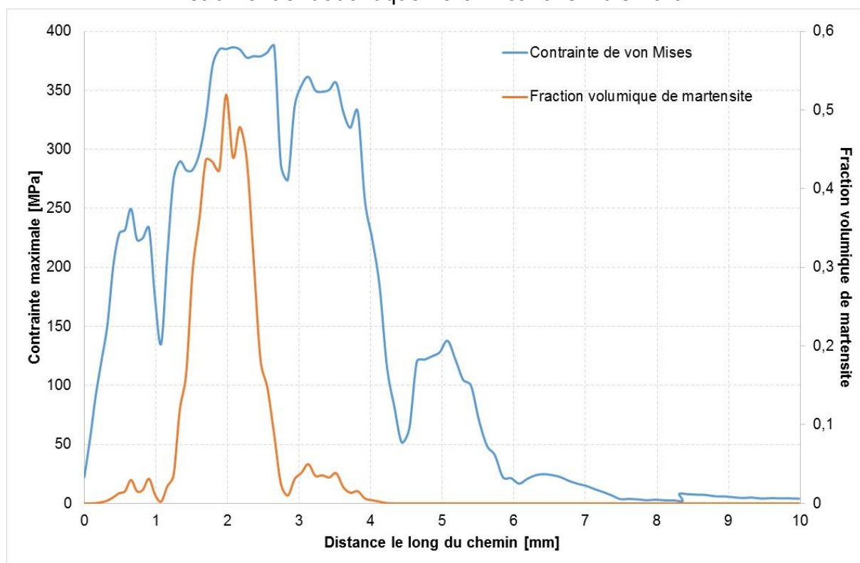
Figure 4.7c. Courbes des contraintes maximales de von Mises et de la fraction volumique de martensite à la fin de l'étape 1 (pénétration + torsion de 20°) pour le couple instrument endodontique 30-04 / canal simulé 25-04.
