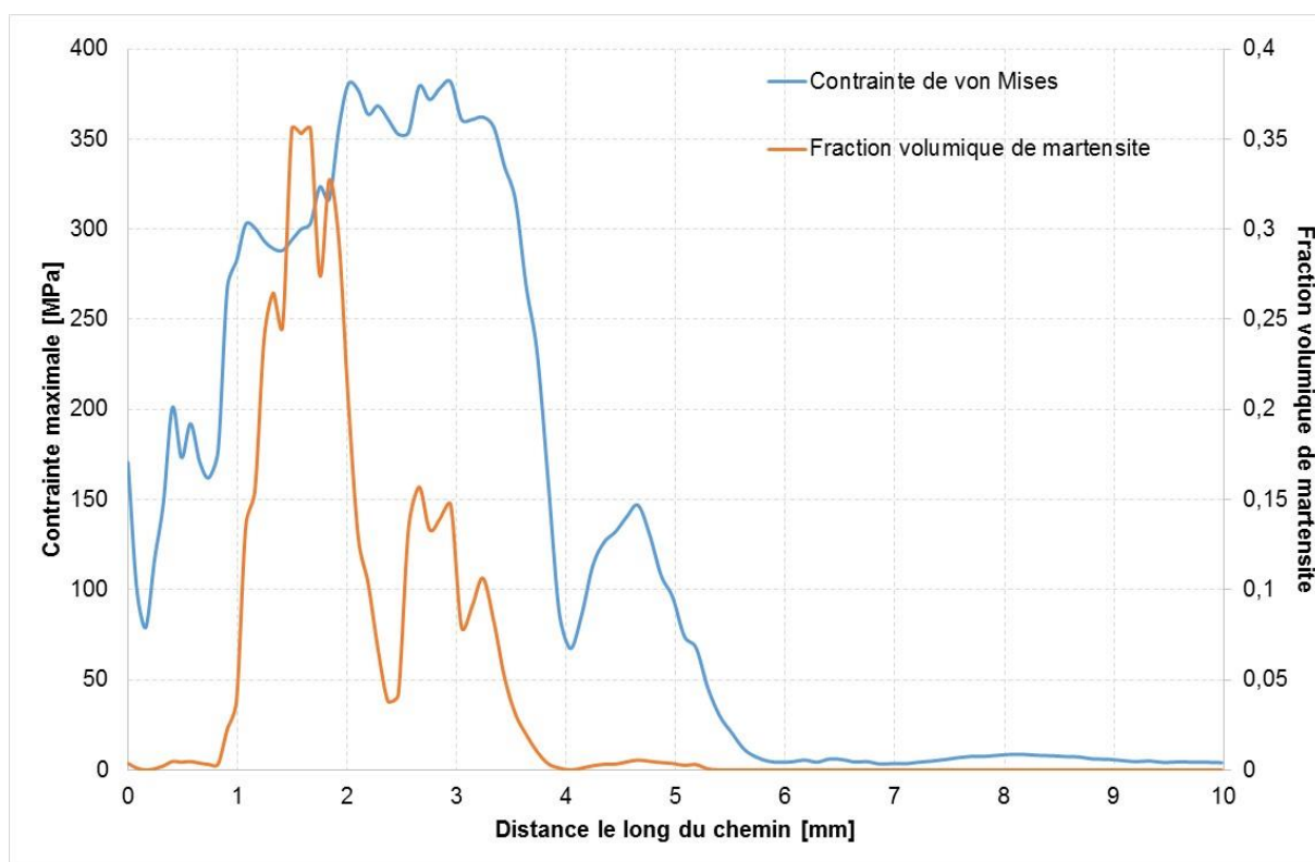
Figure 4.7b. Courbes des contraintes maximales de von Mises et de la fraction volumique de martensite à la fin de l'étape 1 (pénétration canalaire) pour le couple instrument endodontique 25-04 / canal simulé 20-04.
