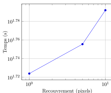
FIGURE 4.17 – Temps d'exécution de l'estimation du flot optique par rapport à la taille du recouvrement.
