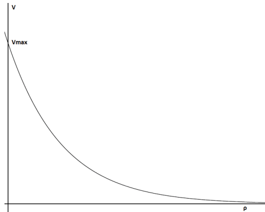
FIGURE 1.3 – Représentation schématique de la vitesse d'Underwood.
