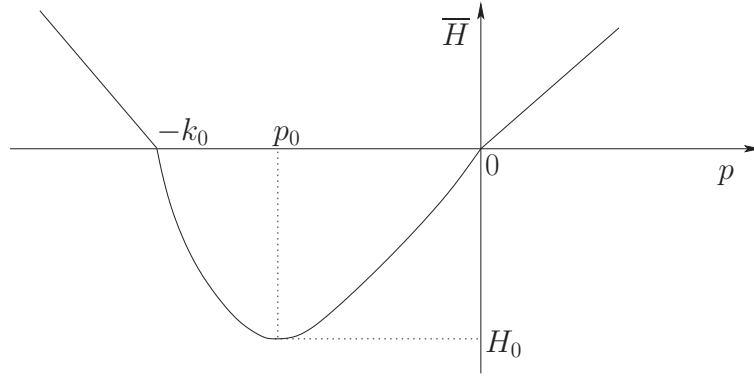
FIGURE 1.9 – Représentation schématique de \bar{H} .
