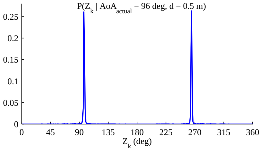
Figure A.2: Distribution de l'AoA mesuré quand la source réelle est à 96° et 0,5 m de l'antenne.
