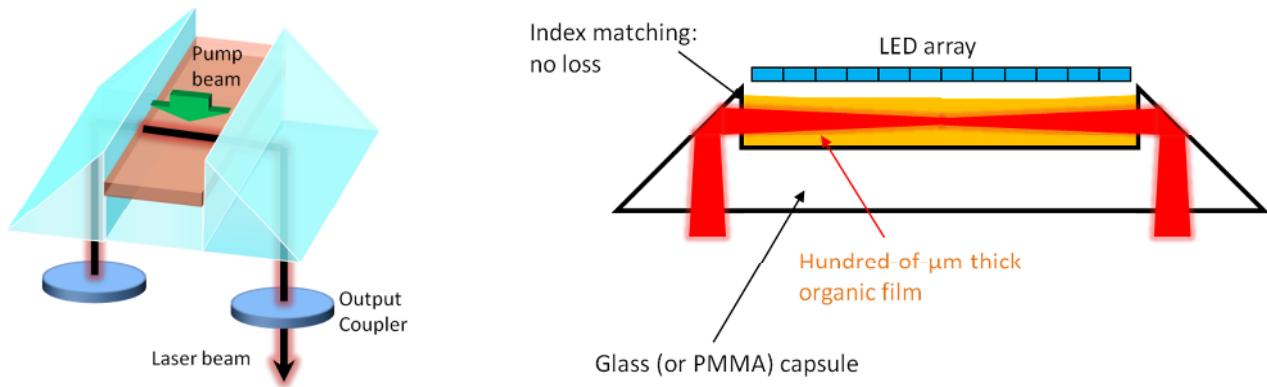
Figure 37 : géométrie proposée dans le projet ANR Edelweis
