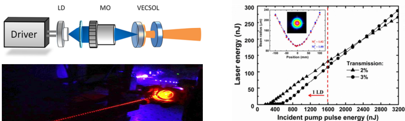
Figure 34 : à gauche, schéma de principe et photo du VECSOL pompé par diode. À droite, performances obtenues avec une ou deux diodes lasers de pompe et différents coupleurs de sortie.
