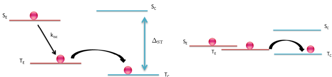
Figure 40 : management des triplets par l'ajout de molécule « charognard ». A gauche, methode « classique » utilisant des molécules à grand splitting \Delta_{ST} , à gauche notre proposition avec des molécules à TADF.
