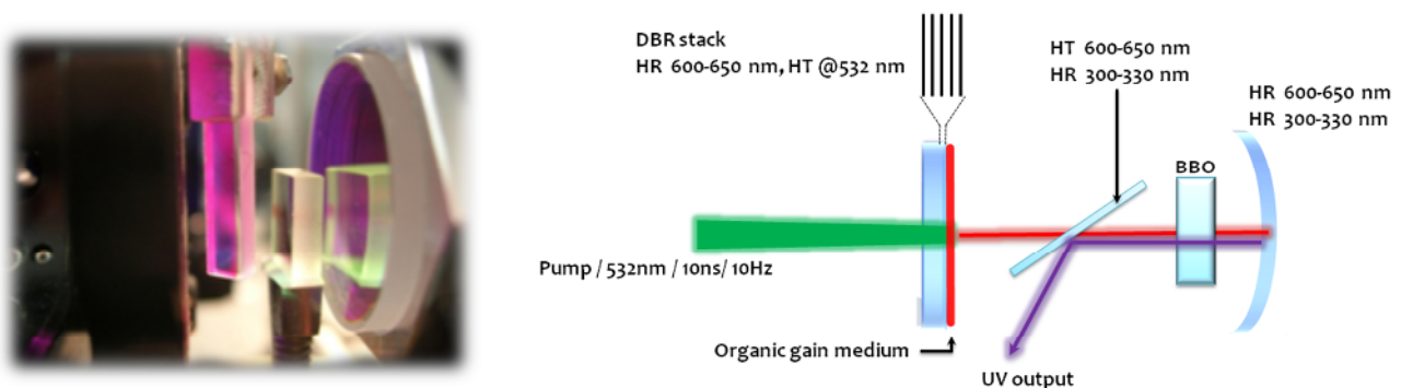
Figure 30 : schéma du VESOUL, un VEC SOL doublé intracavité. À gauche, photo du système en vue latérale.
