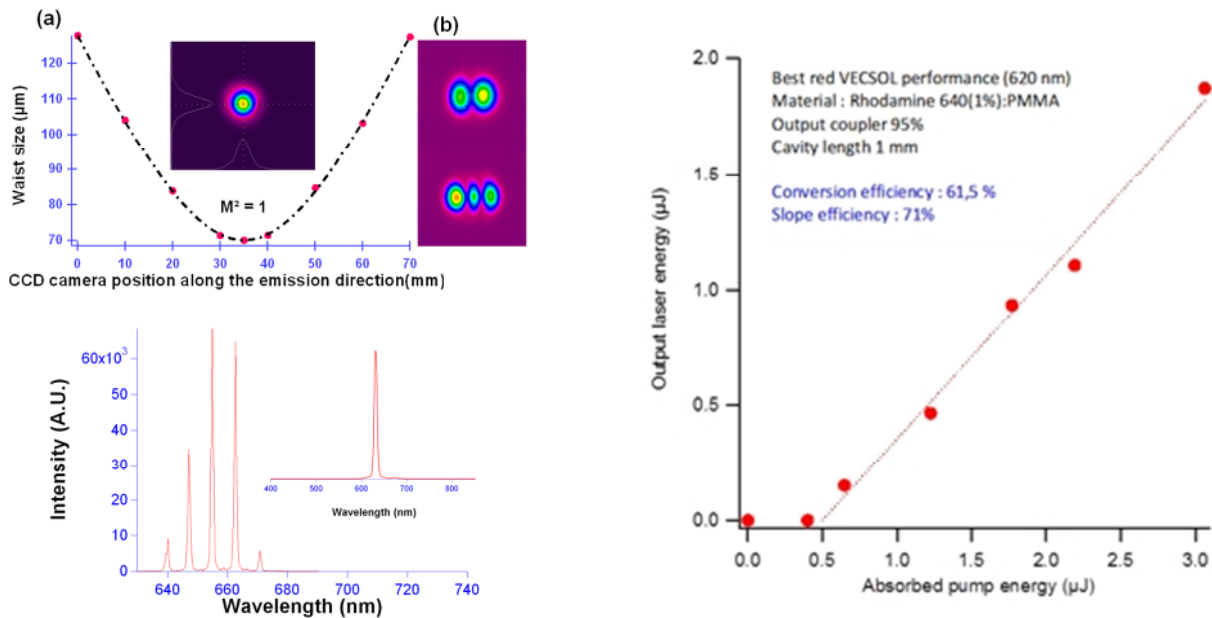
Figure 29 : en haut à gauche : Profil du faisceau de sortie du VEC SOL et mesure du M^2 (en insert : autres modes transverses obtenus via un léger désalignement de la cavité) ; en bas à gauche : spectre du VEC SOL avec une couche de 18 μm d'épaisseur (en insert, spectre mono-pic obtenu en réduisant l'épaisseur à 2 μm). A droite : efficacité du VEC SOL pour un coupleur de sortie optimisé de R=95\% et une cavité ultra-courte.
