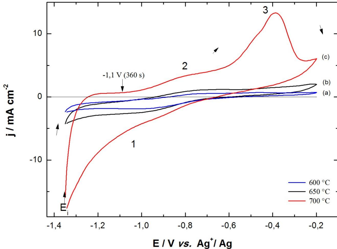
Figure 4.17 : Effet de la température sur \text{Li}_2\text{CO}_3\text{-Na}_2\text{CO}_3\text{-K}_2\text{CO}_3 sous une atmosphère de 100 % \text{CO}_2 , P(\text{CO}_2) = 1 bar. Voltampérogrammes cycliques enregistrés avec une électrode d'or ( S = 2 \text{ cm}^2 ) après une pré-électrolyse à -1,1 \text{ V} (360 s) à différentes températures (a) 600 \text{ }^\circ\text{C} , (b) 650 \text{ }^\circ\text{C} et (c) 700 \text{ }^\circ\text{C} . E_i = -1,35 \text{ V vs. Ag}^+/\text{Ag} , v = 100 \text{ mV s}^{-1} .
