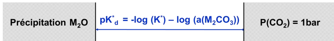
Figure 1.5 : Domaine d'oxoacidité dans les carbonates fondus.
