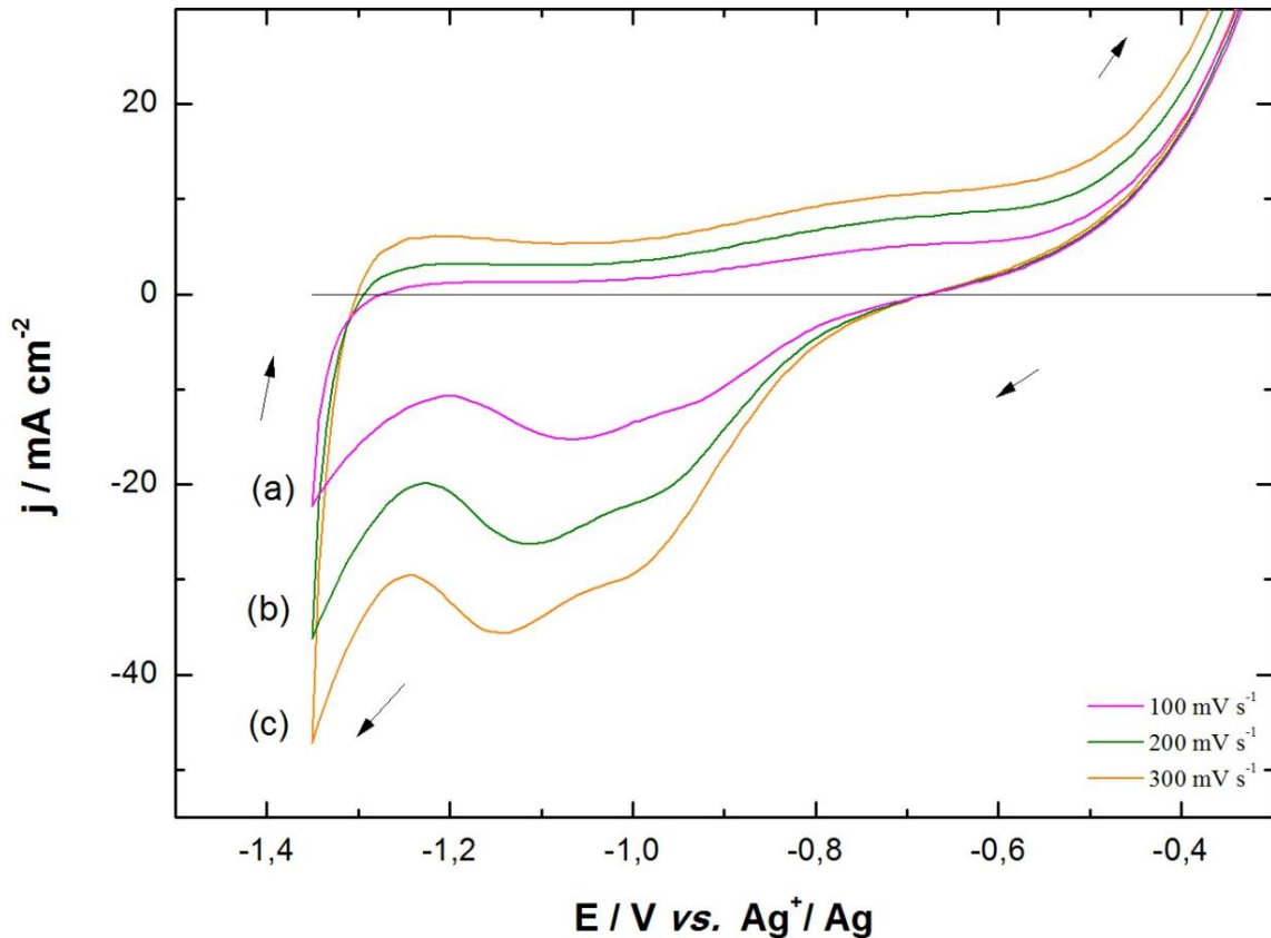
Figure 4.26 : Voltampérogrammes cycliques à une électrode carbone graphique ( S = 2,8 \text{ cm}^2 ) dans \text{Li}_2\text{CO}_3\text{-K}_2\text{CO}_3 à 650 \text{ }^\circ\text{C} sous P \text{ totale} = 1 \text{ bar} avec P(\text{Argon})=P(\text{CO}_2) = 0,5 \text{ bar} pour différentes vitesses, v à différentes vitesses (a) 100 \text{ mV s}^{-1} , (b) 200 \text{ mV s}^{-1} (c) 300 \text{ mV s}^{-1} , (d) 100 \text{ mV s}^{-1} (e) 200 \text{ mV s}^{-1} , (f) 300 \text{ mV s}^{-1} , (g) 400 \text{ mV s}^{-1} , (h) 500 \text{ mV s}^{-1} . E_i = -0,2 \text{ V vs. Ag}^+/\text{Ag} .
