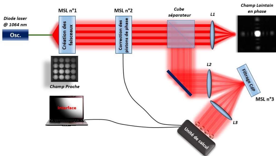
Figure III-17 : Schéma descriptif du banc modèle expérimental ayant permis la démonstration du principe de la méthode de phasage PIM.
