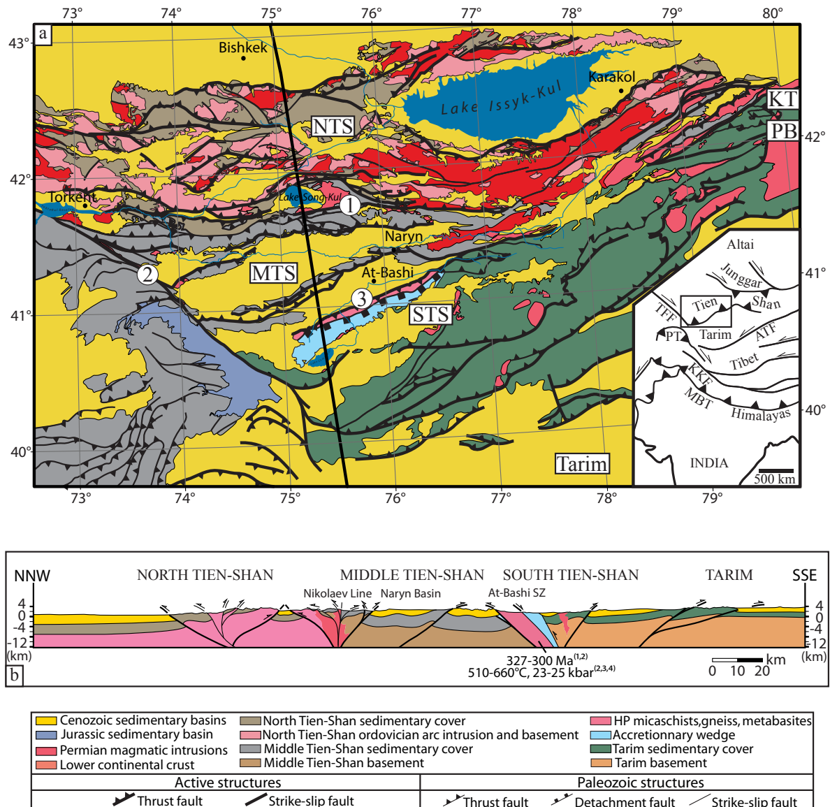
Figure 1-4 : Carte géologique du Tien Shan (modifiée d'après Jukov et al., 2008). Le trait noir épais indique la localisation de la coupe. NTS : North Tien Shan. MTS: Middle Tien Shan. STS: South Tien Shan. KT: Khan Tengri. PB: Pobeda. 1: Nikolaev Line, 2: Faille de Talas Ferghana, 3: Zone de suture d'At-Bashi.
