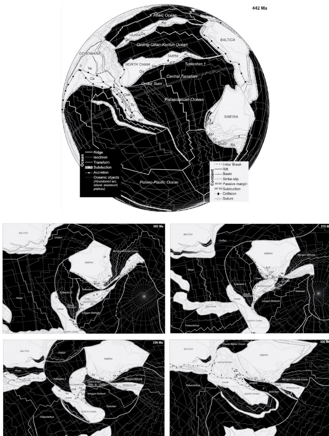
Figure I-2 : Reconstruction des mouvements des plaques tectoniques qui constituent aujourd'hui la CAOAB du Silurien au Carbonifère supérieur (Wilhem et al., 2012)
