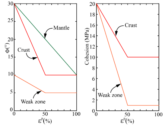
Figure III-2 : Diminution de la friction (à gauche) et de la cohésion (à droite) en fonction de la déformation plastique \epsilon jusqu'à un maximum de déformation plastique accumulée \epsilon_{\infty} pour différentes phases
