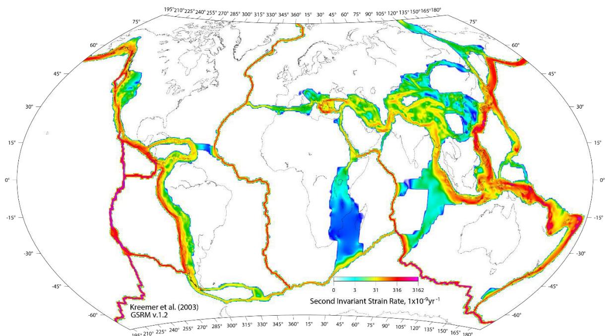
Figure 1 : Carte des vitesses de déformation à la surface de la Terre (Kreemer et al., 2003)
