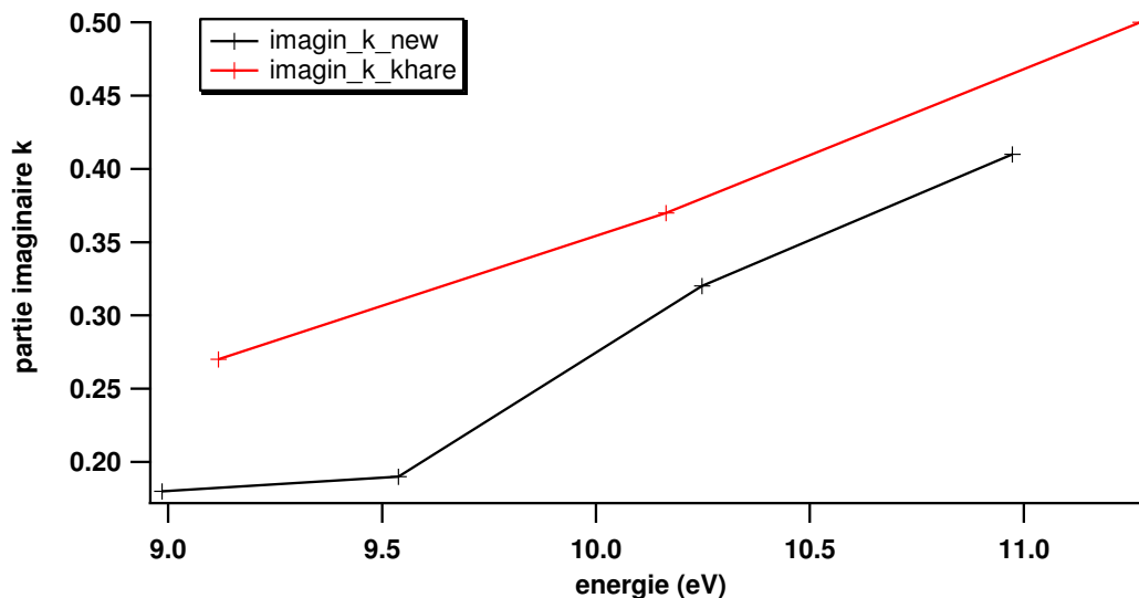
Figure 82. Comparaison des parties imaginaires des indices optiques VUV obtenues pour des films organiques de type tholins entre (Khare et al. 1984) (courbe rouge) et notre étude (Gavilan, communication personnelle) (courbe noire).
