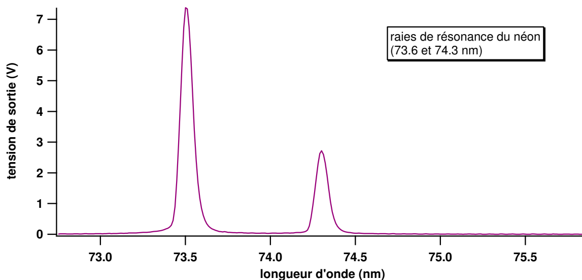
Figure 16. Les deux raies de résonance principales du néon à 73.6 nm et 74.3 nm, mesurées par notre système d'acquisition. Le signal de sortie est donc ici en volts. Pour ces intensités mesurées, la pression en néon est de 1.5 mbar et la puissance micro-onde de 70 W.
