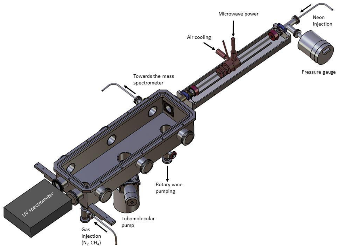
Figure 17. Schéma descriptif du montage expérimental de la source VUV (à droite) couplée sans séparation au réacteur APSIS (au centre) avec le spectromètre UV (face au hublot de sortie, à gauche).
