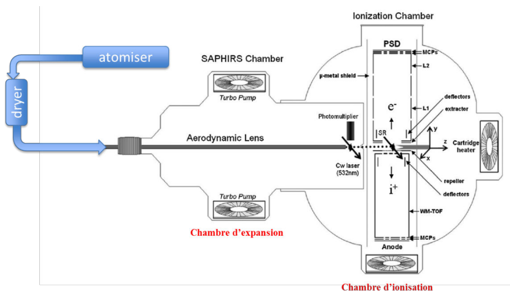
Figure 58. Schéma du dispositif d'ionisation des nanoparticules sur la plateforme SAPHIRS de la ligne DESIRS. La lentille aérodynamique permet l'injection de nanoparticules libres dans la chambre d'ionisation sous vide où arrive de façon perpendiculaire le rayonnement synchrotron VUV. Les électrons et/ou les ions ainsi créés sont séparés par un champ électrique constant pour atteindre les détecteurs sensibles en position. Tiré de (Gaie-Levrel et al. 2011).
