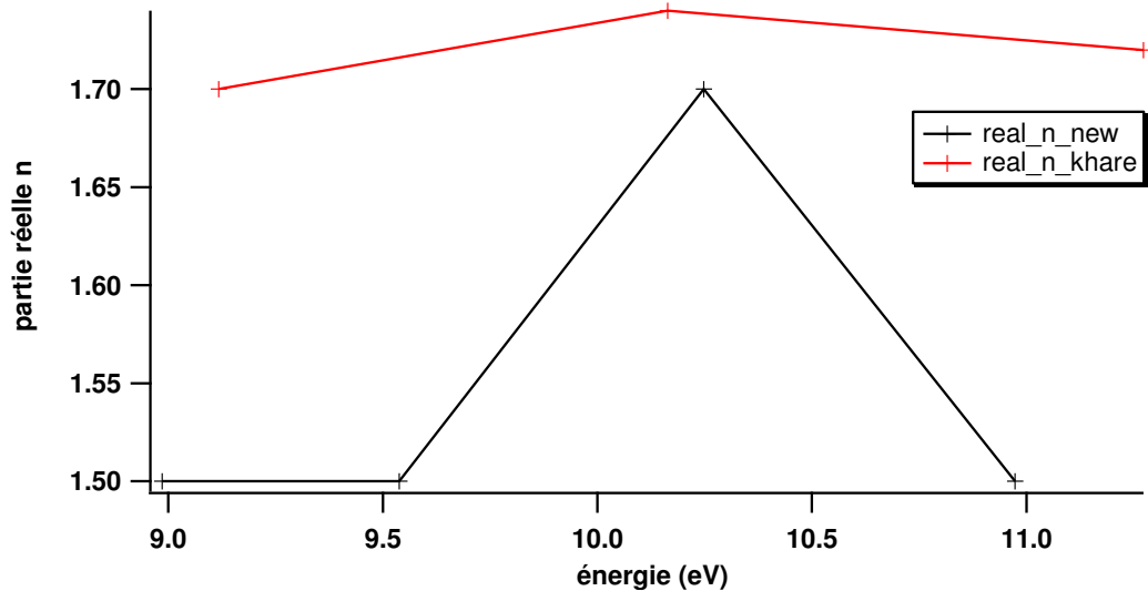
Figure 81. Comparaison des parties réelles des indices optiques VUV obtenues pour des films organiques de type tholins entre (Khare et al. 1984) (courbe rouge) et notre étude (Gavilan, communication personnelle) (courbe noire).
