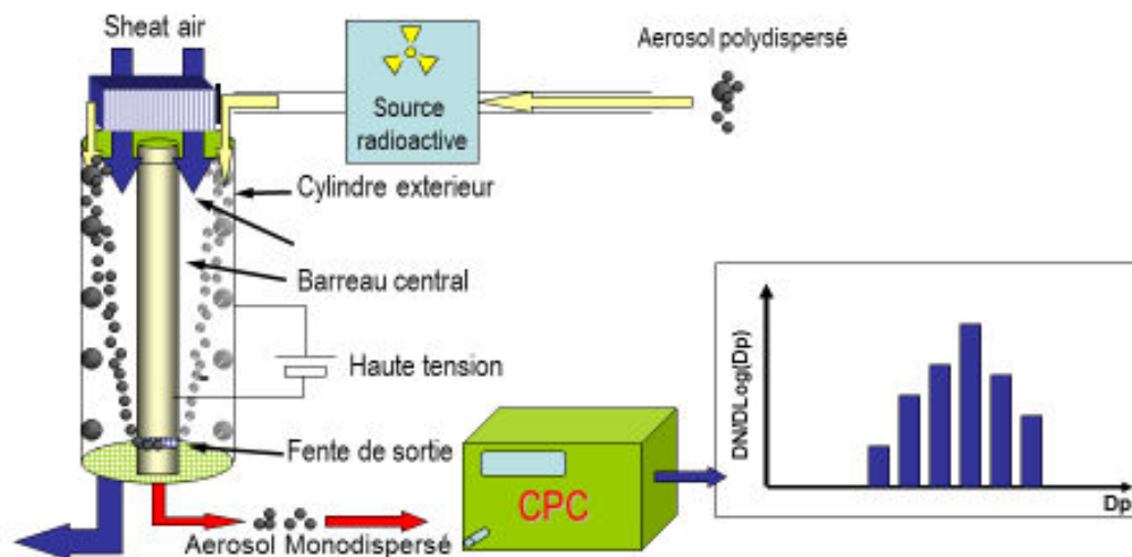
Figure 51. Schéma de fonctionnement d'un SMPS : le DMA (analyse de la mobilité) couplé au CPC (compteur de nanoparticules) pour obtenir la distribution en taille.
