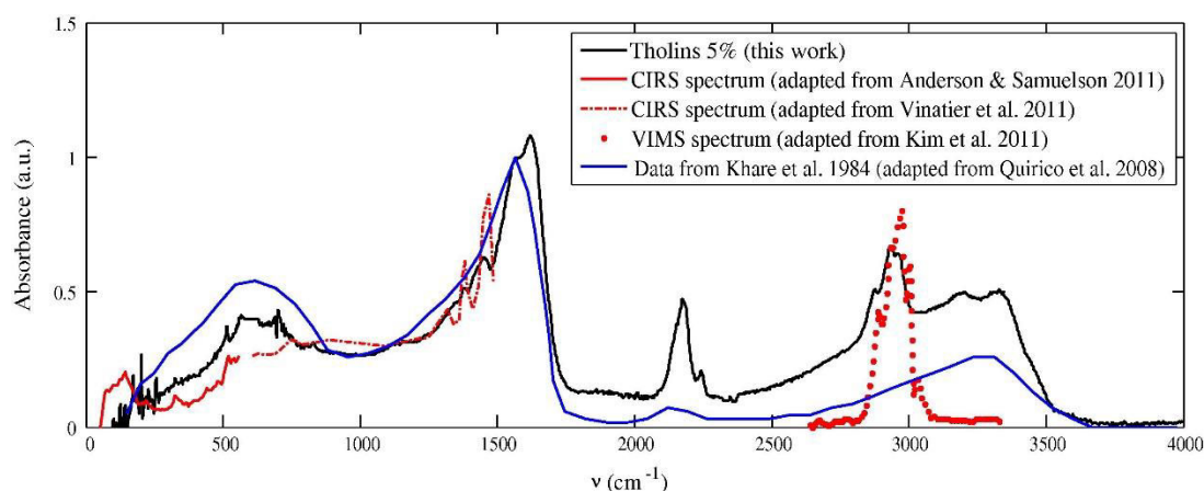
Figure 50. Spectre d'absorption des tholins dans l'infra-rouge lointain et moyen provenant de (Gautier et al. 2012). La courbe noire représente la signature des tholins à 5% de PAMPRE, la courbe bleue provient des données de (Khare et al. 1984), les données de Cassini-CIRS de (Anderson & Samuelson 2011) et (Vinatier et al. 2011) ainsi que celles de Cassini-VIMS (Kim et al. 2011) sont représentées avec les lignes rouges (pleines et pointillées).
