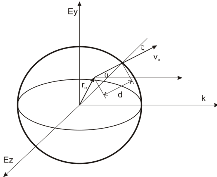
Figure 78. Schéma de photoémission élastique d'un électron provenant de la position r_e dans une nanoparticule sphérique.
