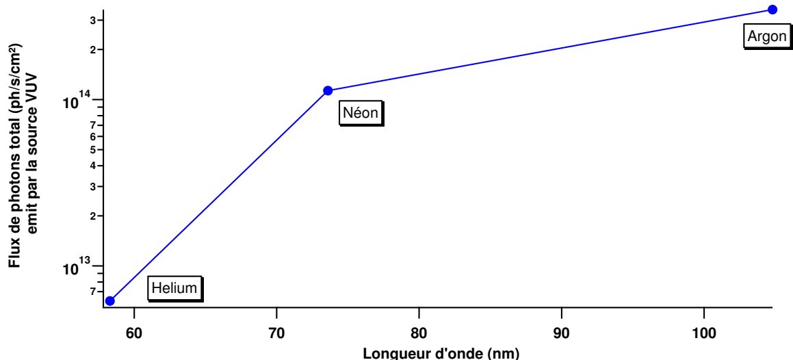
Figure 24. Flux de photons ( ph. s^{-1}. cm^{-2} ) délivrés par la source VUV aux différentes longueurs d'onde d'émission des gaz rares utilisés dans la décharge.
