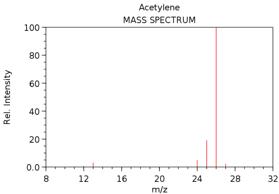
Figure 38. Spectre de masse de l'acétylène C_2H_2 (NIST)
