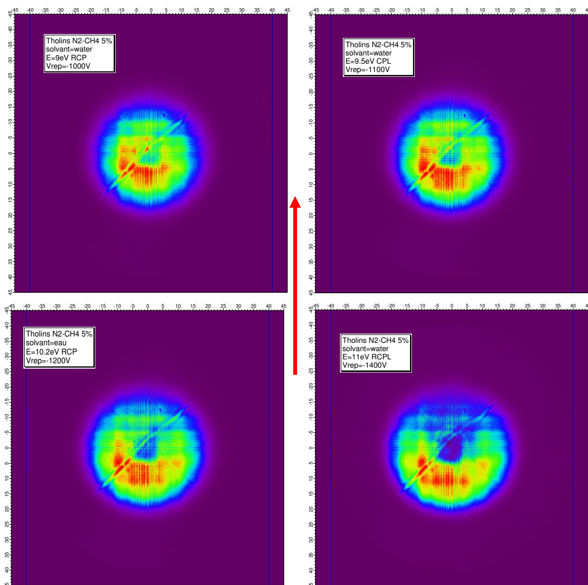
Figure 74. On retrouve les asymétries avant/arrière à différentes énergies d'irradiation. Ici de gauche à droite et de bas en haut: 9 eV, 9.5 eV, 10.2 eV et 11 eV. La flèche rouge sur le côté indique le sens de propagation de la lumière VUV.
