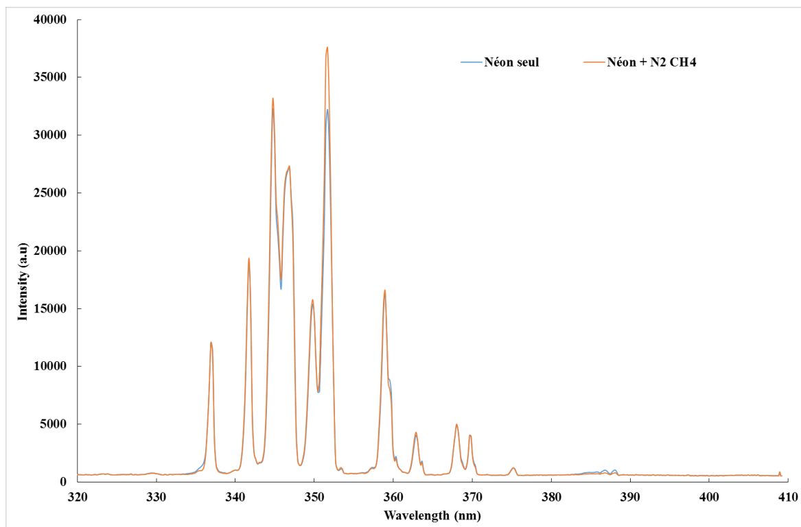
Figure 19. Spectre d'émission d'une décharge néon non couplée au réacteur APSIS (courbe bleue) comparé au spectre de la décharge branchée au réacteur (courbe orange) : le fait que les deux coïncident parfaitement indique que dans cette configuration expérimentale N_2 ne subit aucune excitation électronique, donc le plasma ne pénètre pas dans le réacteur.
