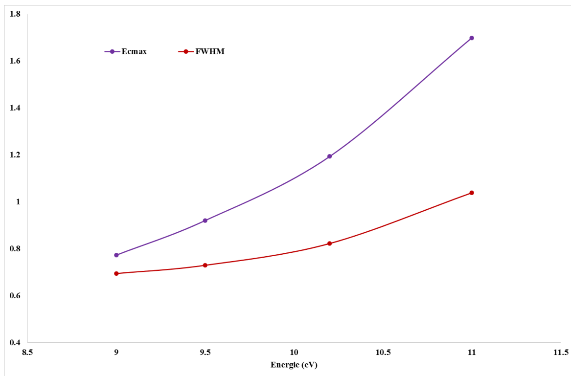
Figure 64. Evolution du pic d'énergie cinétique et de la FWHM en fonction de l'énergie des photons
