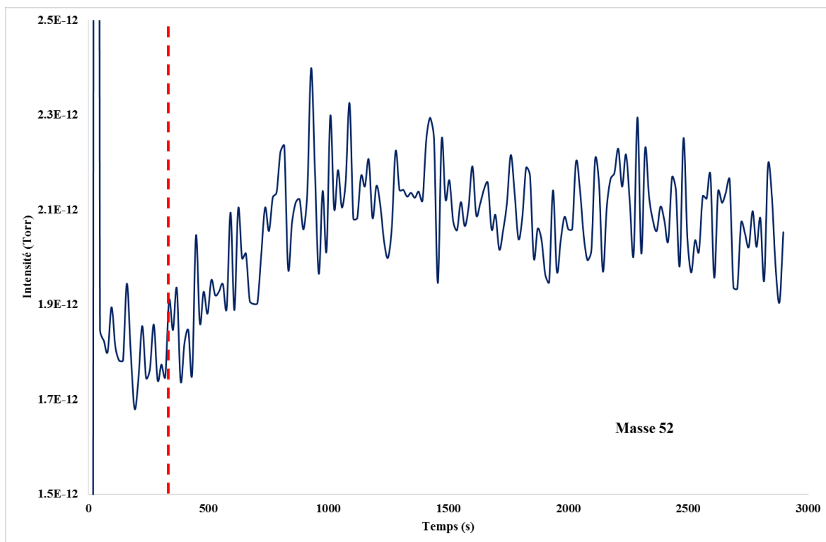
Figure 32. Suivi MID de la masse m/z 52 pour une irradiation à 73.6 nm.
