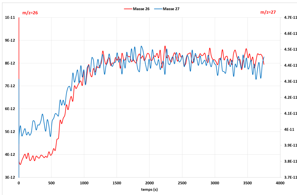
Figure 42. Suivi MID des masses m/z 26 (courbe rouge, échelle de gauche) et m/z 27 (courbe bleue, échelle de droite).
