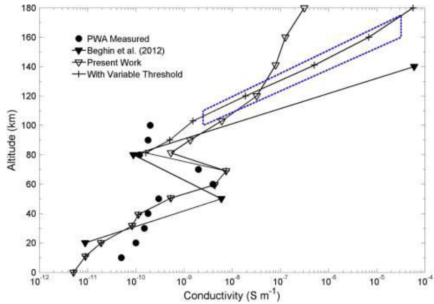
Figure 67. Comparaison entre différents profils de conductivité dans l'atmosphère de Titan, dont les données de l'instrument PWA/Huygens et les valeurs de (Mishra et al. 2014) qui fait varier le seuil d'ionisation en fonction de l'altitude.
