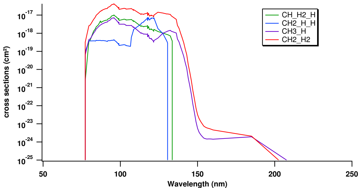
Figure 40. Sections efficaces partielles de dissociation du méthane CH 4 . Données de la base du SWRI : http://phidrates.space.swri.edu/
