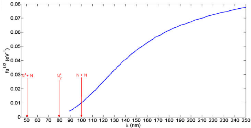
Figure 10. Fonction de distribution des électrons d'un plasma d'azote pur similaire à celui de PAMPRE calculé par (Alves et al. 2012) et adapté par (Fleury 2016). Les barres rouges marquent les seuils d'activation des réactions de dissociation et d'ionisation de N_2 .
