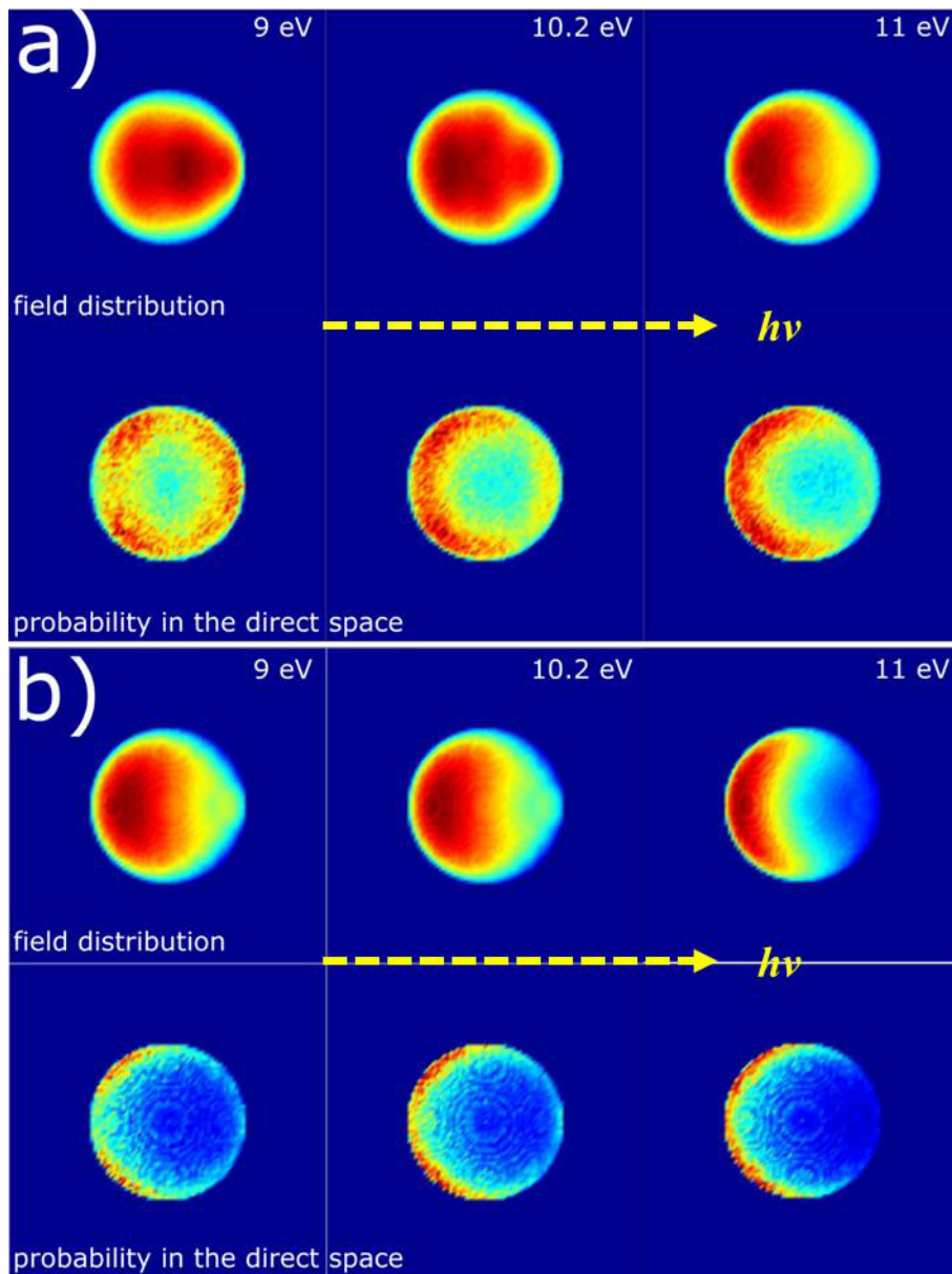
Figure 77. Distribution du champ électrique |\vec{E}(x, y, z)|^2 et probabilités de photoémission pour des nanoparticules de tholins sphériques aux différentes énergies et aux deux diamètres majoritaires 140 nm (a) et 360 nm (b). Les flèches jaunes pointillées indiquent l'axe de propagation de la lumière ( h\nu ).
