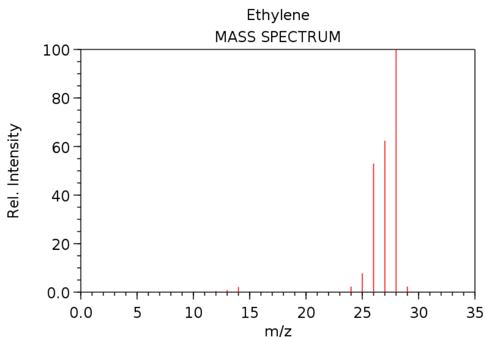
Figure 37. Spectre de masse de l'éthylène C_2H_4 (NIST)
