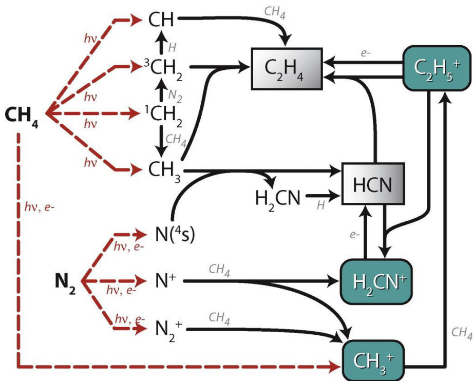
Figure 43. Schéma de formation de HCN et C 2 H 4 à partir des photolyses de N 2 et CH 4 . (De La Haye et al. 2008)
