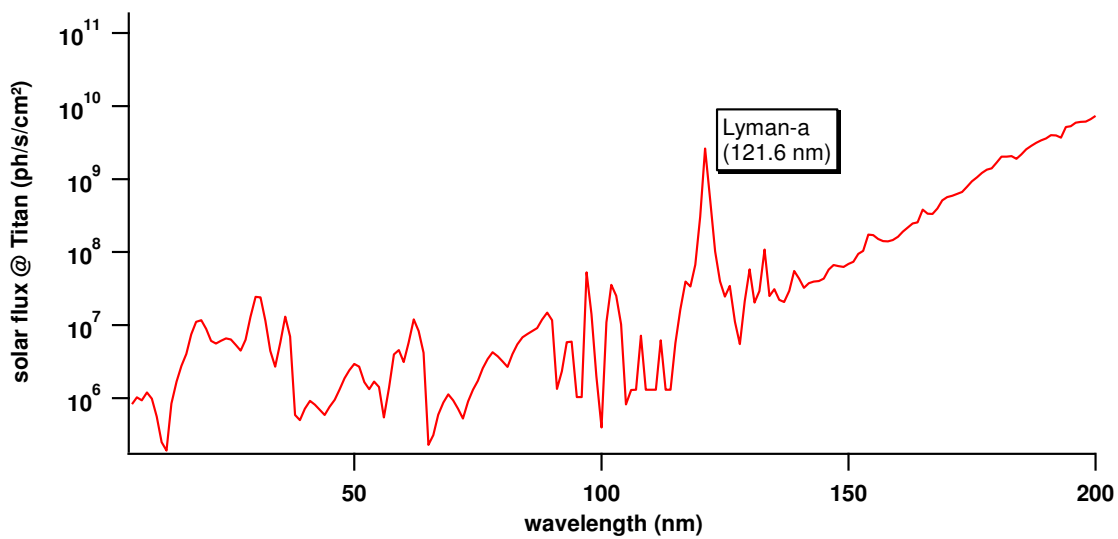
Figure 46. Flux solaire VUV jusqu'à 200 nm à la distance de Titan (10 UA).
