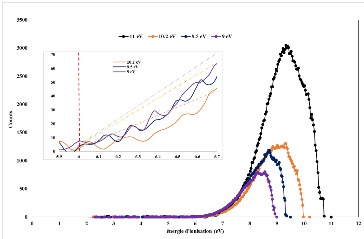
Figure 62. Spectre de photoélectrons pour différentes énergies de photons (11, 10.2, 9.5 et 9 eV). On remarque sur le zoom dans l'encadré que l'énergie minimale nécessaire pour obtenir des « coups » sur le détecteur, correspondant aux électrons produits, est d'environ 6.0 \pm 0.1 eV.
