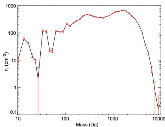
Figure 44. Spectre en masse ( m/z ) fourni par l'instrument CAPS à bord de Cassini à une altitude de 1000 km. Des ions lourds, jusqu'à 8 000 Da, et de charge négative sont observés. Ces tailles correspondent aux agrégats de PAHs précurseurs des aérosols (Waite et al. 2007).
