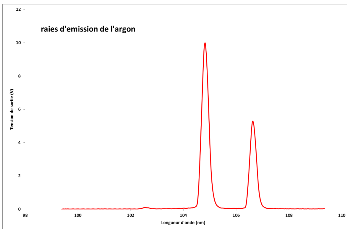
Figure 20. Spectre des raies d'émission principales de l'argon à 104.8 et 106.6 nm.
