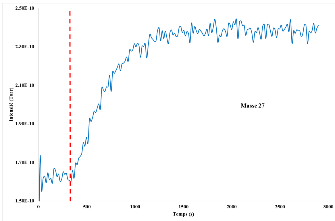
Figure 31. Suivi MID de la masse m/z 27 pour une irradiation à 73.6 nm.
