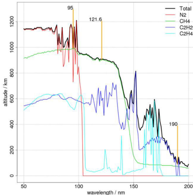
Figure 47. Profils \tau(\lambda)=1 du rayonnement VUV dans la haute atmosphère de Titan pour les composés principaux à savoir N_2 , CH_4 , C_2H_2 et C_2H_4 à partir de leurs profils de densités respectifs ainsi que leurs sections efficaces d'absorption. La courbe noire représente l'absorption totale.
