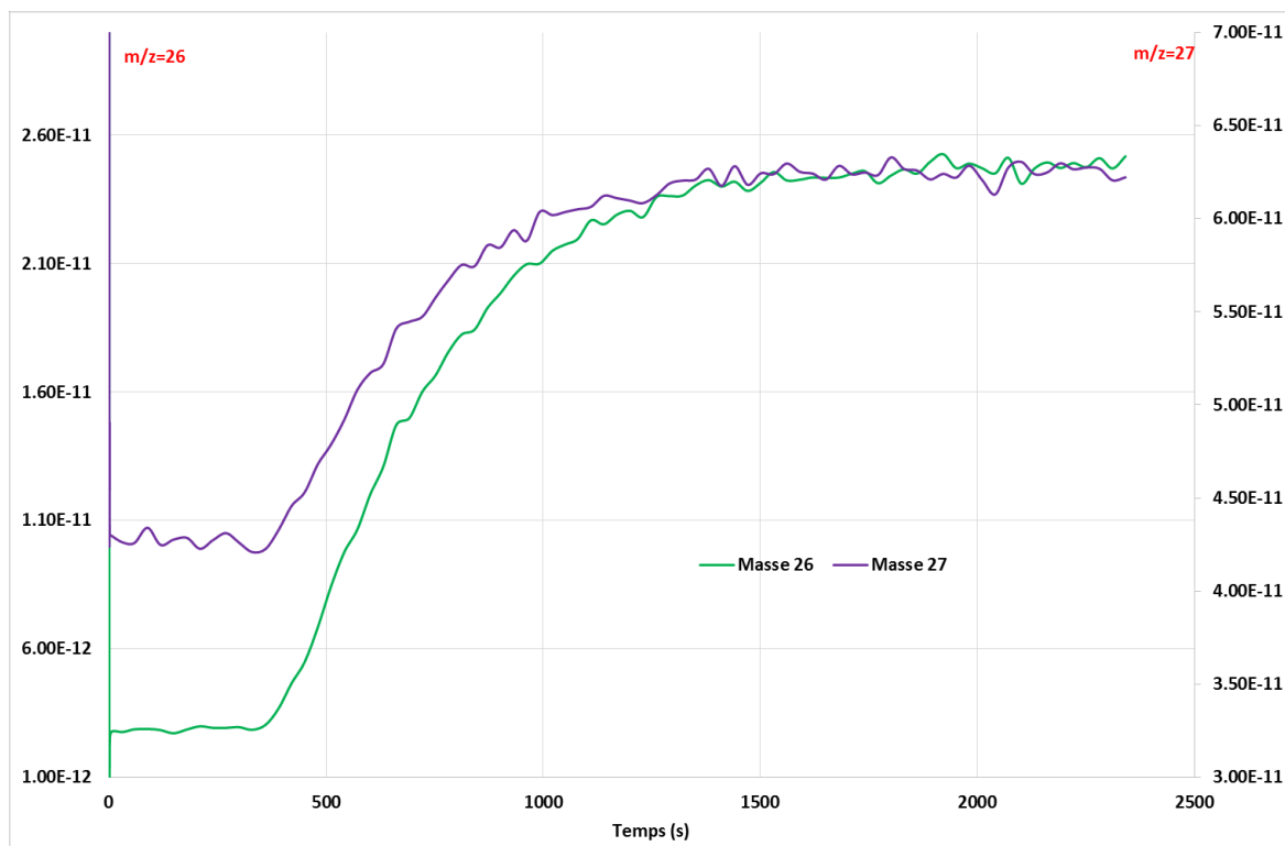
Figure 34. Suivi MID des masses m/z 26 (courbe verte, échelle de gauche) et m/z 27 (courbe violette, échelle de droite) pour une irradiation à 58.4 nm.
