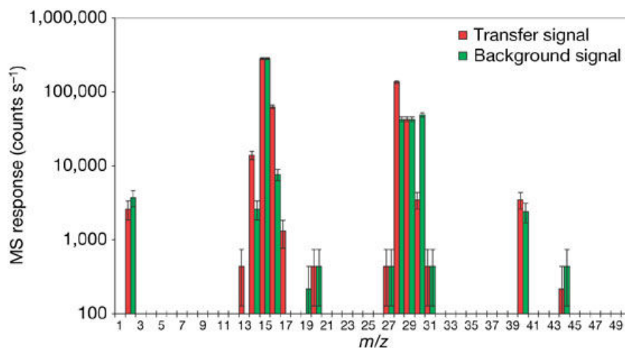
Figure 6. Spectre de masse du gaz issu de la pyrolyse des aérosols dans l'instrument ACP publié dans (Israël et al. 2005).
