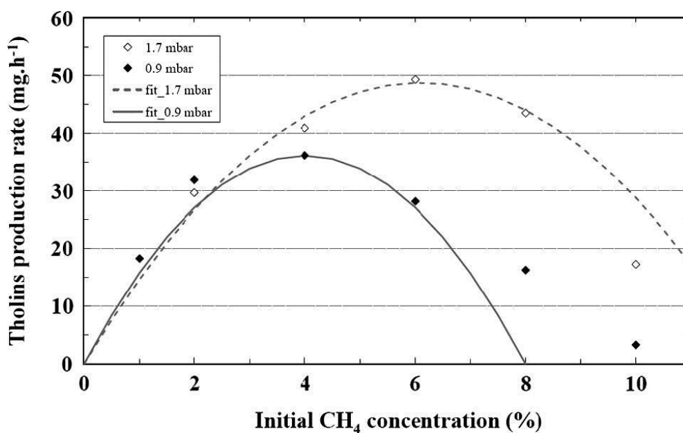
Figure 48. Taux de production des tholins dans PAMPRE en fonction de la concentration initiale en méthane dans le mélange réactif du plasma. Les mesures et les fits ont été fait à deux pressions 0.9 mbar et 1.7 mbar et présentent le même comportement parabolique.
