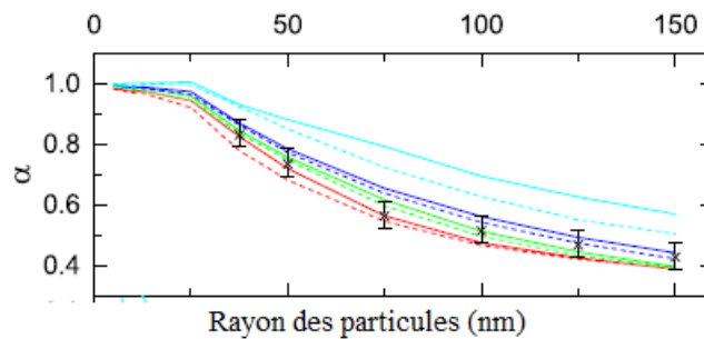
Figure 84. Comparaison entre les sorties du modèle de (Goldmann et al. 2015) et leurs résultats expérimentaux à 10 eV (croix noires) en fonction du rayon des nanoparticules. Les différentes courbes correspondent aux modèles avec différents LPMI entre 0.2 (rouge, pointillée) et 10 nm (courbe cyan, pleine).
