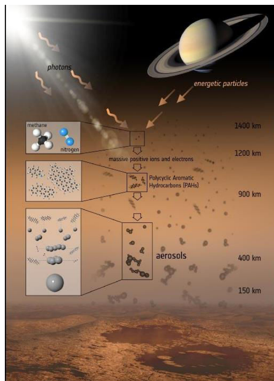
Figure 4. Schéma de formation des aérosols dans la haute atmosphère de Titan.
