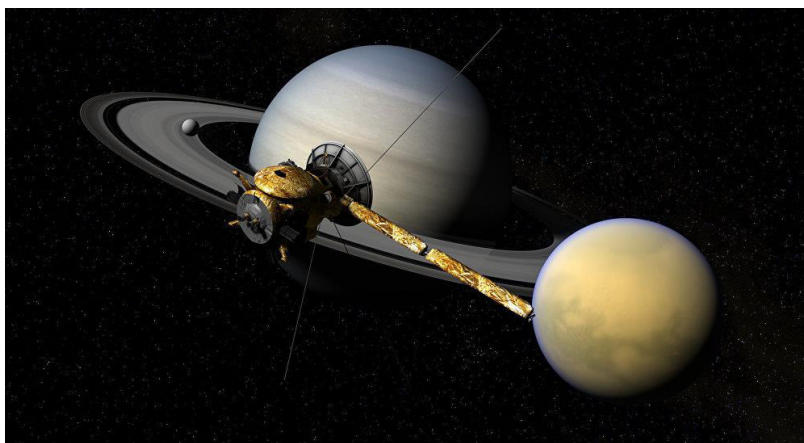
Figure 2. Vue d'artiste de la sonde Cassini autour du système Saturnien (ici : Titan, Encelade et Saturne)
