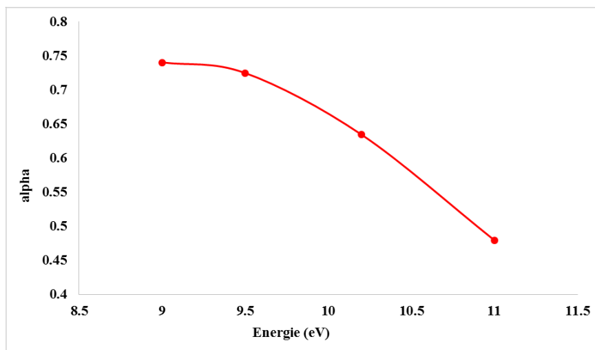
Figure 75. Dépendance en énergie du paramètre d'asymétrie \alpha mesuré expérimentalement pour les tholins N_2-CH_4 injectés dans SAPHIRS avec la distribution en taille de la Figure 73.
