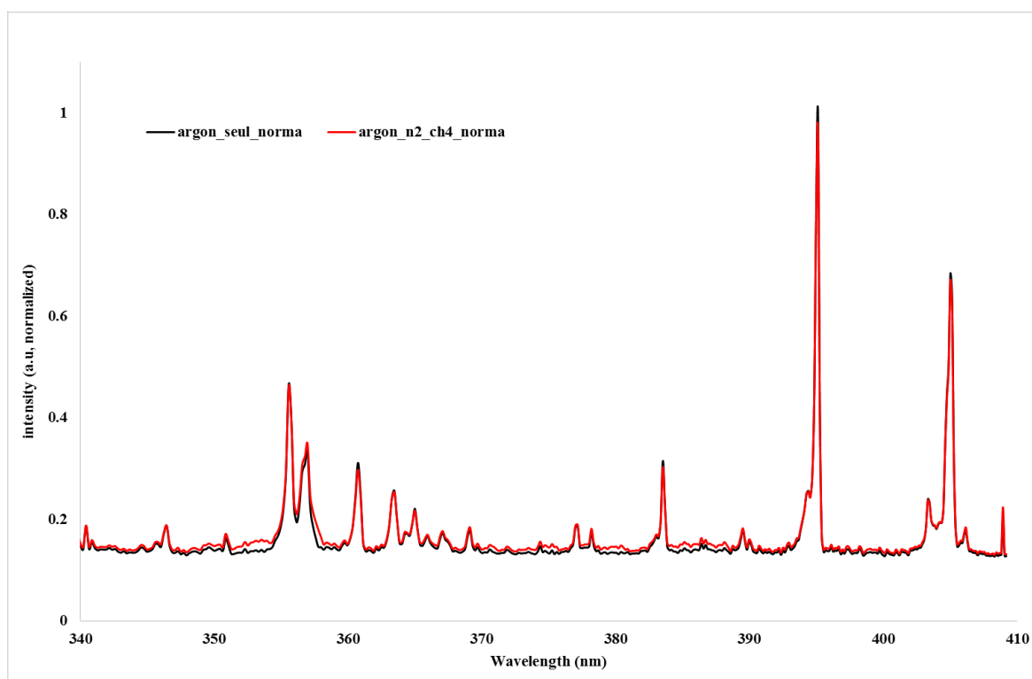
Figure 21. Spectre d'émission UV de l'argon seul (courbe noire) puis de l'argon face au mélange N_2 - CH_4 dans les conditions d'utilisation pour de la photochimie sur APSIS (courbe rouge). L'intensité est normalisée.
