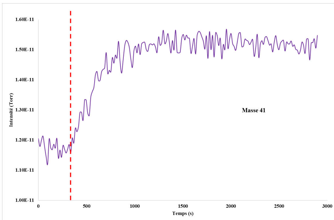
Figure 30. Suivi MID de la masse m/z 41 pour une irradiation à 73.6 nm.
