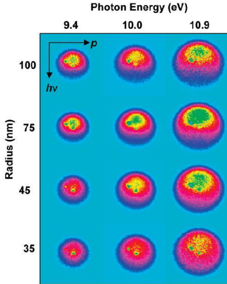
Figure 71. Images de la photoionisation VUV de nanoparticules de NaCl de différentes tailles (échelle verticale) et pour différentes énergies (échelle horizontale). La dépendance en taille et en énergie de l'asymétrie \alpha est ici très claire. Extrait de (Wilson et al. 2007).
