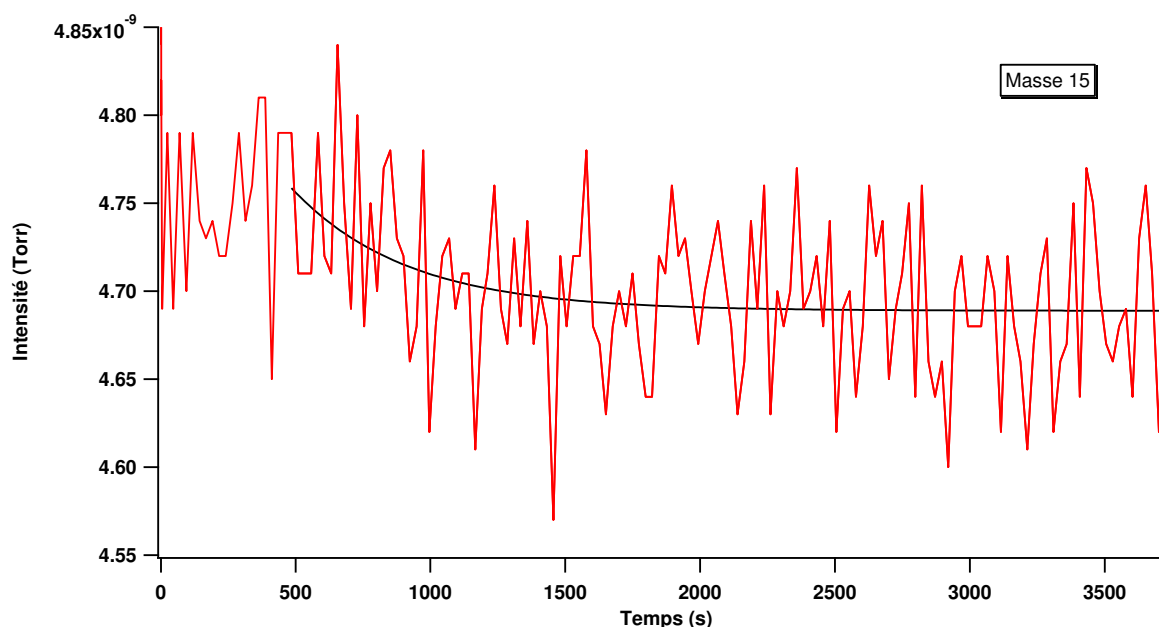
Figure 41. Suivi temporel de la consommation de méthane, via son fragment \text{CH}_3^+ à m/z = 15 uma, pour une irradiation à 104.8 nm.
