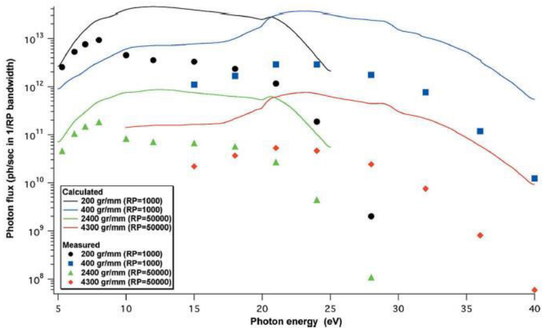
Figure 54. Flux de photons délivré par la ligne DESIRS du synchrotron SOLEIL en polarisation linéaire verticale et en fonction de l'énergie des photons. Les symboles (points, carrés, triangles, losanges) correspondent au flux mesuré par une photodiode AXUV 100 (comme pour le monochromateur VUV du Chapitre 1) ; tandis que les lignes pleines représentent les simulations optiques. Tiré de (Nahon et al. 2012).
