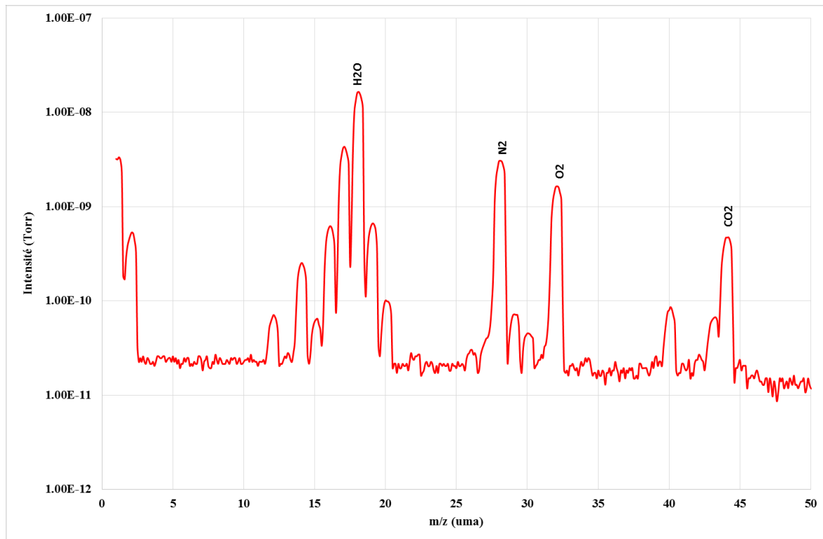
Figure 27. Spectre de masse du SM HIDEN isolé sur lui-même. On reconnaît les signatures de l'eau et de l'air résiduels qu'il faut prendre en compte lors de l'étude des spectres.
