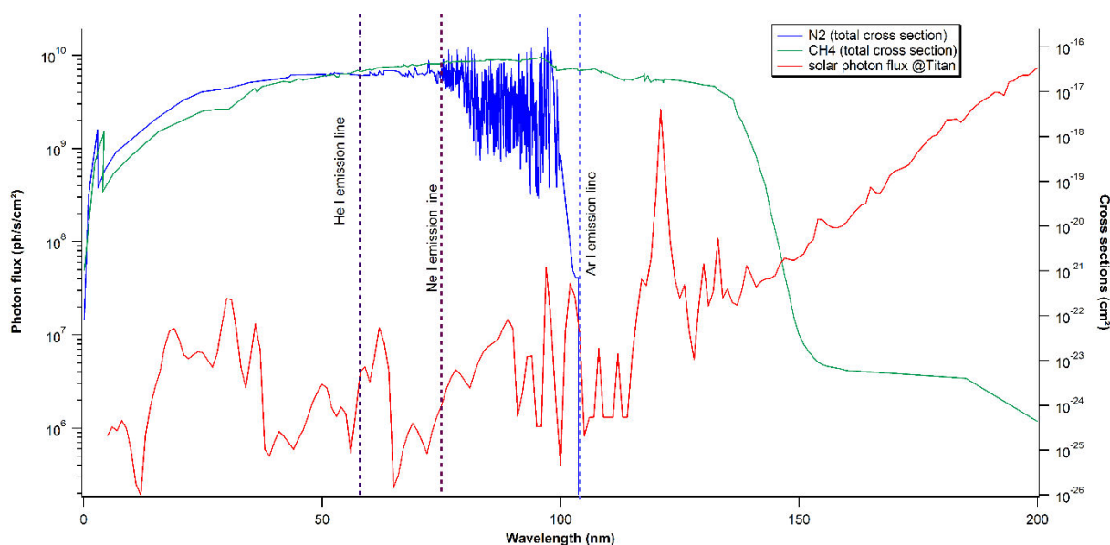
Figure 14. Raies d'émission principales disponibles avec notre source VUV de laboratoire pour l'hélium, le néon et l'argon (lignes verticales et pointillées). Elles sont ici mises en perspective par rapport aux sections efficaces de nos réactifs N_2 (courbe bleue) et CH_4 (courbe verte), ainsi que par rapport au flux solaire incident à la distance moyenne de Titan (courbe rouge).
