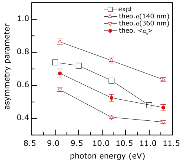
Figure 83 Comparaison entre les valeurs d'asymétrie \alpha calculées par le modèle aux deux diamètres majoritaires à 140 (triangles haut rouges) et 360 nm (triangles bas rouges) par rapport aux données expérimentales (carrés noirs). Les points rouges représentent la moyenne des asymétries générées par les deux diamètres et se superposent aux données expérimentales. Les indices optiques utilisés ici sont ceux de (Khare et al. 1984).
