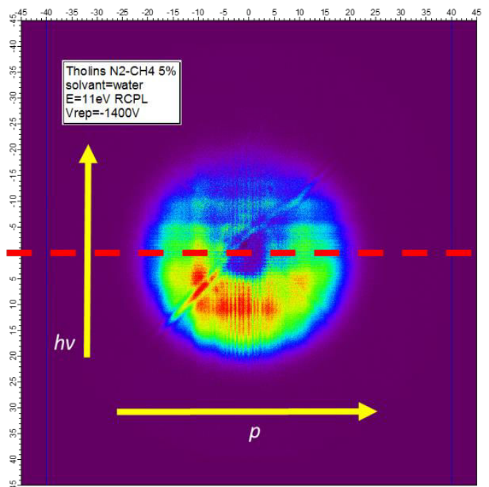
Figure 69. Projection 2D de la photo-émission des nanoparticules de tholins à 11 eV obtenue avec le VMI sur SAPHIRS. La ligne rouge pointillée sépare le détecteur de position en deux demi disques symétriques par rapport à l'axe de propagation de la lumière indiqué, lui, par la flèche jaune ( h\nu ). La seconde flèche jaune ( p ) indique la direction de propagation des nanoparticules.
