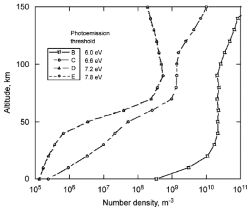
Figure 66. Profils de densités de photoélectrons en fonction de l'altitude associés à des seuils d'ionisation des aérosols entre 6 et 7.8 eV (Borucki & Whitten 2008). Les courbes à 7.2 et 7.8 eV sont confondues.
