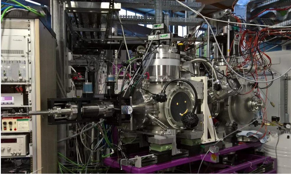
Figure 57. L'enceinte expérimentale SAPHIRS sur la branche A de DESIRS. A gauche se trouve la lentille aérodynamique d'injection de l'échantillon. A droite se trouvent les chambres d'expansion et d'ionisation. Le faisceau synchrotron arrive par derrière.
