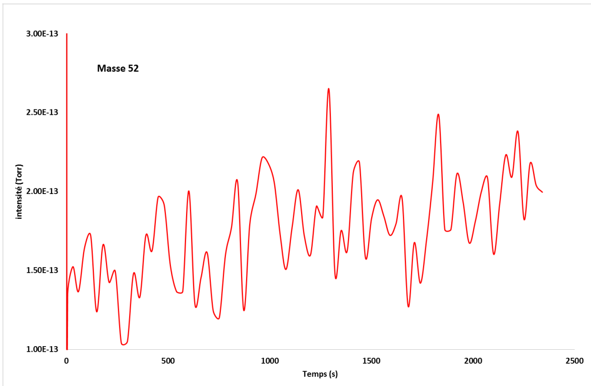
Figure 35. Suivi MID de la masse m/z 52 pour une irradiation à 58.4 nm.
