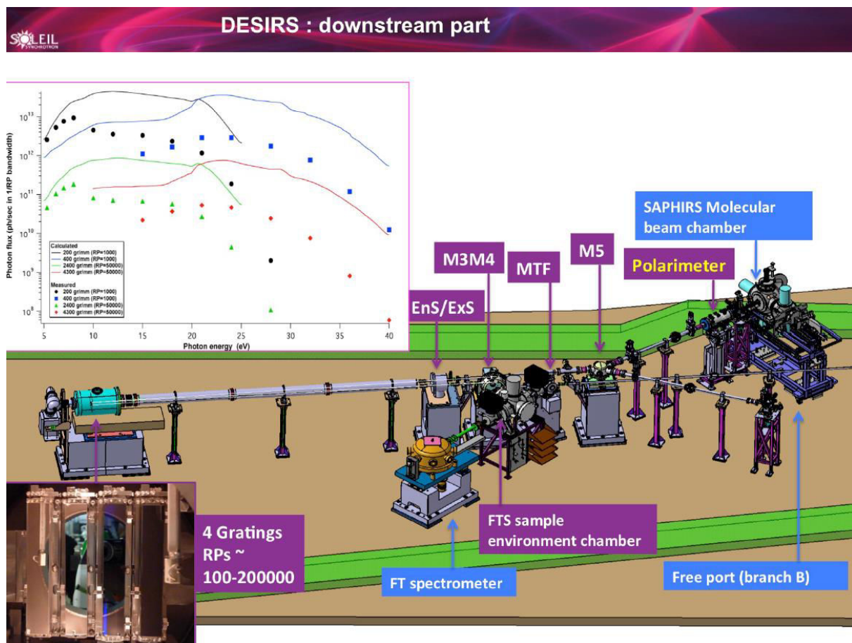
Figure 56. Aval de la ligne DESIRS avec les quatre réseaux (zoom en bas à gauche), les différents miroirs et la branche SAPHIRS.
