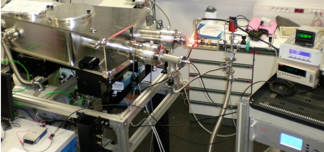
Figure 15. Photo du montage de calibration de la source VUV branchée sur le monochromateur VUV (à gauche).
