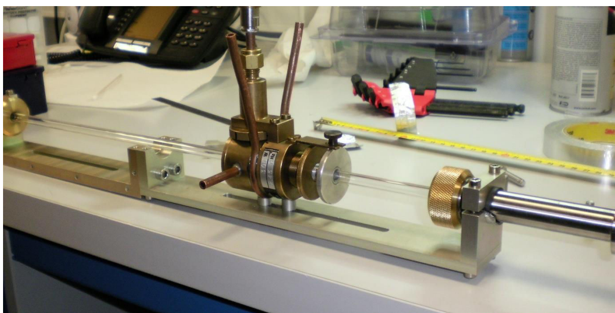
Figure 13. Photographie de notre lanceur d'onde type « surfatron ». L'onde micro-onde arrive par l'antenne branchée en haut de l'appareil ; les deux piquages latéraux permettent la circulation du système de refroidissement (ici de l'eau). L'onde de surface se déplace le long des parois du tube de quartz placé au centre du surfatron et où s'effectue la décharge.
