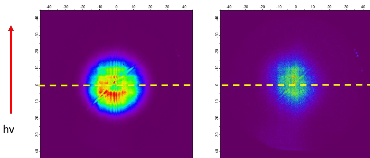
Figure 70. (A) Image brute non corrigée de la distribution des électrons issus de la photoionisation des tholins à 9 eV. On remarque bien que l'image n'est pas symétrique par rapport à l'axe de propagation de la lumière. (B) Image du blanc (eau) toujours à 9 eV. L'absence d'asymétrie avant/arrière est corrélée à l'absence de nanoparticules. Notons que l'image (B) n'est plus circulaire car la région d'interaction devient très étendue (le gaz résiduel photoionisé n'est pas confiné)
