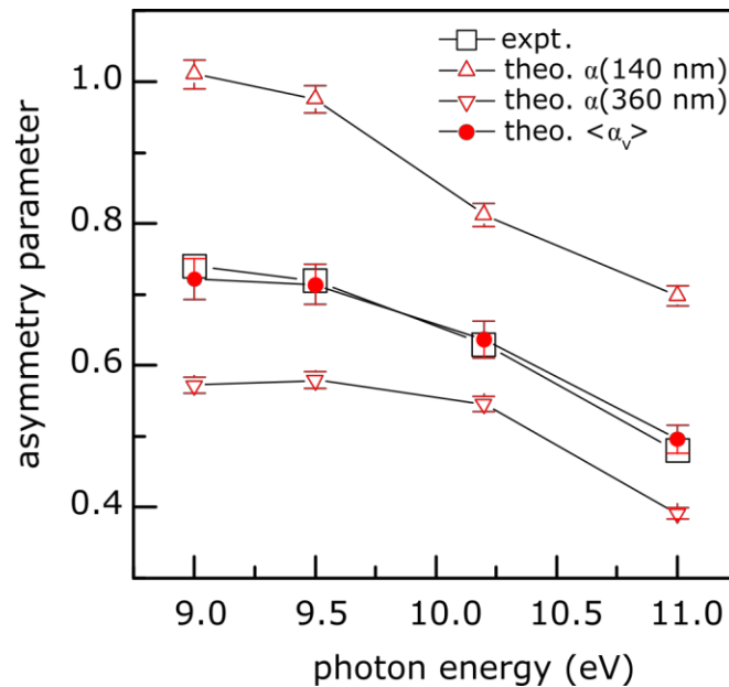
Figure 80. Comparaison entre les valeurs d'asymétrie \alpha calculées par le modèle aux deux diamètres majoritaires à 140 (triangles haut rouges) et 360 nm (triangles bas rouges) par rapport aux données expérimentales (carrés noirs). Les points rouges représentent la moyenne pondérée des asymétries générées par les deux diamètres et se superposent aux données expérimentales. Les indices optiques utilisés ici sont ceux de L. Gavilan.
