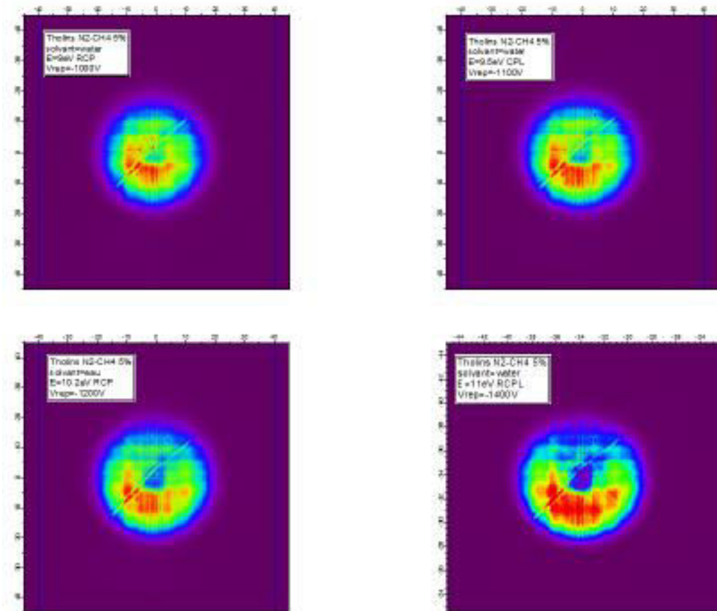
Figure 61. Images corrigées des blancs obtenues pour nos expériences à 9 eV (haut, gauche), 9.5 eV (haut, droit), 10.2 eV (bas, gauche) et 11 eV (bas, droit).
