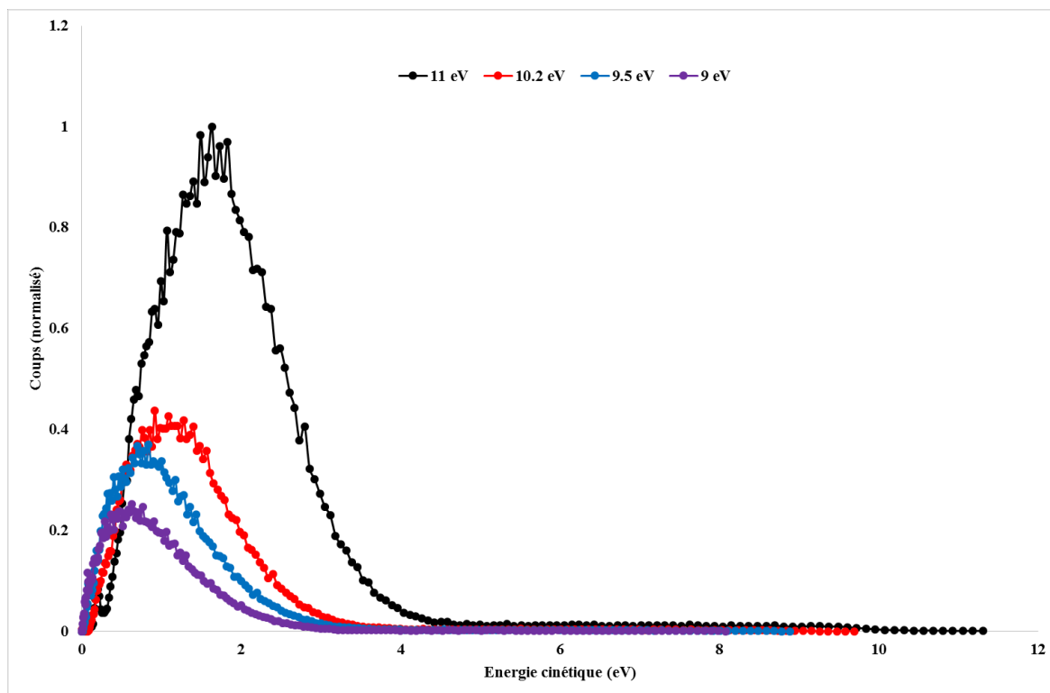
Figure 63. Distribution en énergie cinétique des électrons issus d'une photo-ionisation à différentes énergies incidente.
