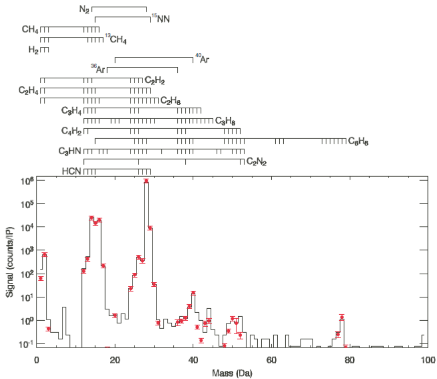
Figure 3. Spectre de masse provenant des mesures INMS du flybys T a entre 1174 et 1230 km d'altitude. Les segments au-dessus représentent les différents fragments de dissociation des espèces dus à la mesure par spectrométrie de masse. Extrait de (Waite et al. 2005).
