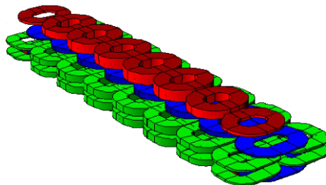
Figure 55. Schéma de l'onduleur OPHELIE 2 illustrant les trois jeux de bobines rouges, bleues et vertes
