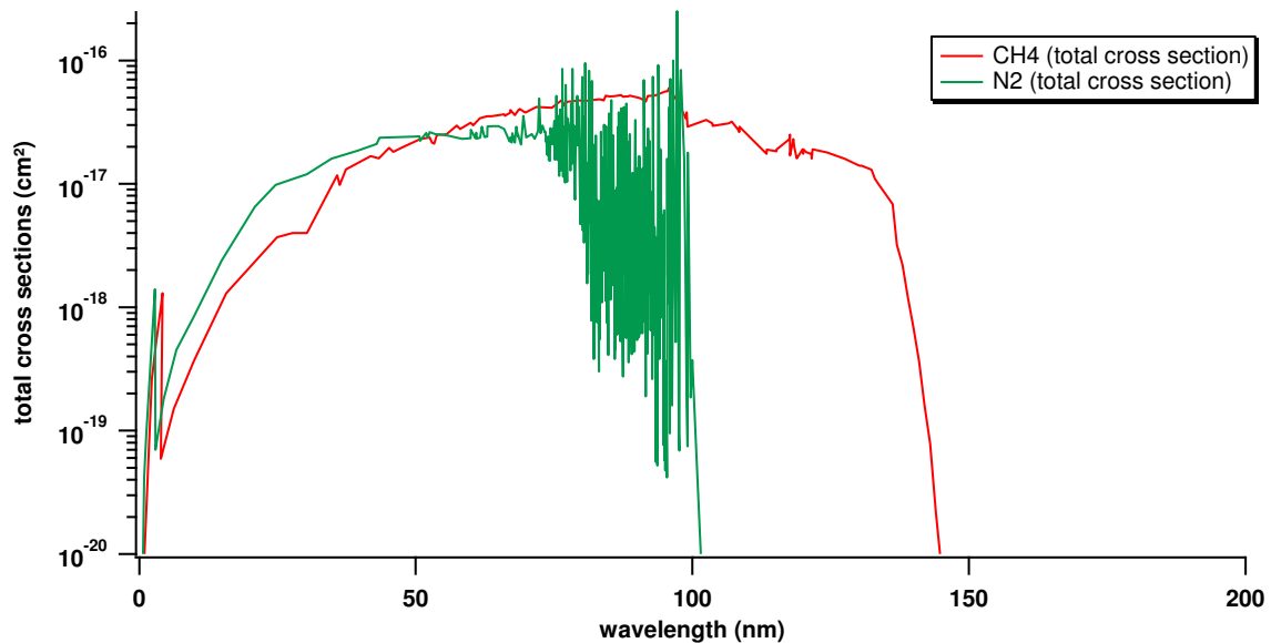
Figure 8. Sections efficaces totales d'absorption du méthane \text{CH}_4 (courbe rouge) et de l'azote moléculaire \text{N}_2 (courbe verte). La coupure est nette pour \text{N}_2 à 100 nm, la molécule devient alors totalement transparente pour des longueurs d'onde supérieures. La diminution est plus progressive pour le méthane, la valeur de sa section efficace devenant quasi négligeable à partir de 150 nm. (Données de la base de données du SWRI : http://phidrates.space.swri.edu/ )
