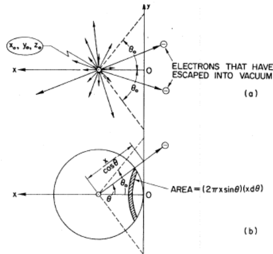
Figure 72. Processus de photoémission et d'échappement des photoélectrons dans le vide décrit dans (Krolikowski & Spicer 1969). La longueur des flèches indique le LPM des électrons avec une vitesse initiale donnée. Seuls les électrons dans le cône pointillé pourront s'échapper.
