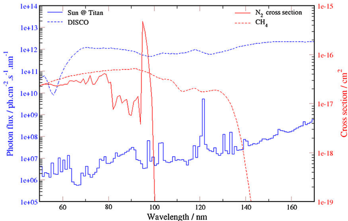
Figure 11. Comparaison entre les flux de photons solaire (ligne bleue, pleine) et celui délivré par la ligne DISCO du synchrotron SOLEIL (ligne bleue, pointillée). En rouge sont tracées les sections efficaces de N_2 et CH_4 .
