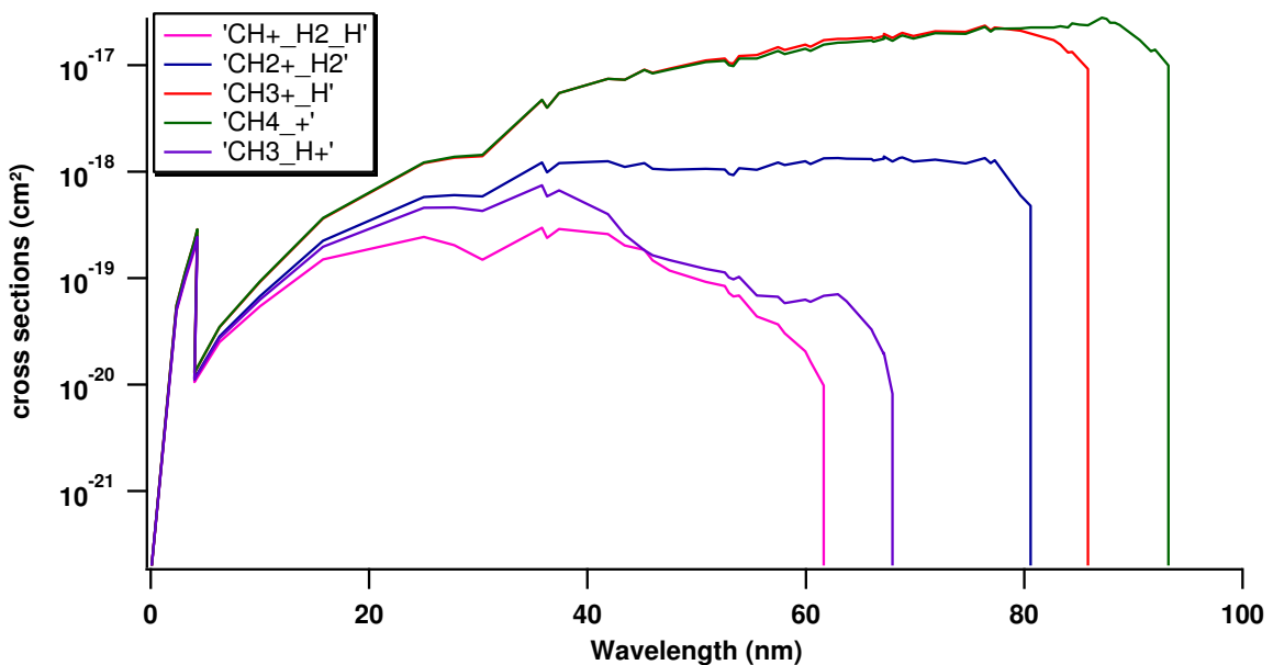
Figure 26. Sections efficaces partielles d'ionisation dissociatives du méthane CH_4 . Les valeurs ont été déterminées expérimentalement avec une incertitude estimée à environ 15%. Données de la base du SWRI : http://phidrates.space.swri.edu/
