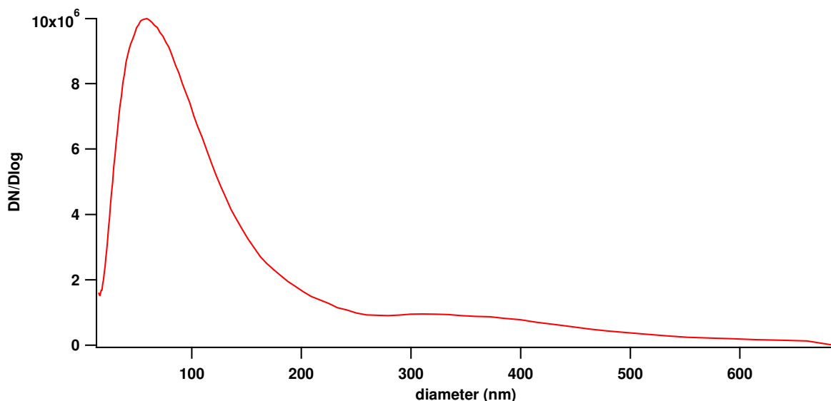
Figure 73. Distribution en taille des tholins mesurée par SMPS.
