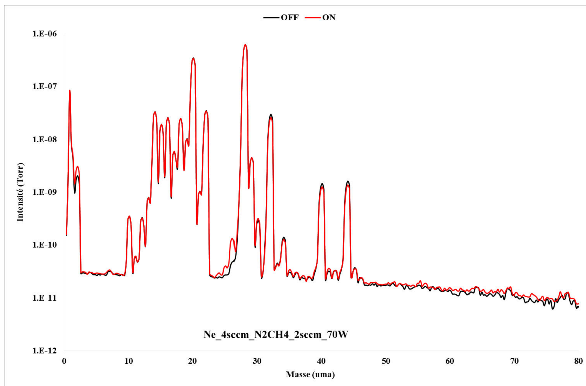
Figure 29. Spectres de masse analogues de notre milieu réactionnel avant (courbe noire) et après (courbe rouge) irradiation à 73.6 nm.
