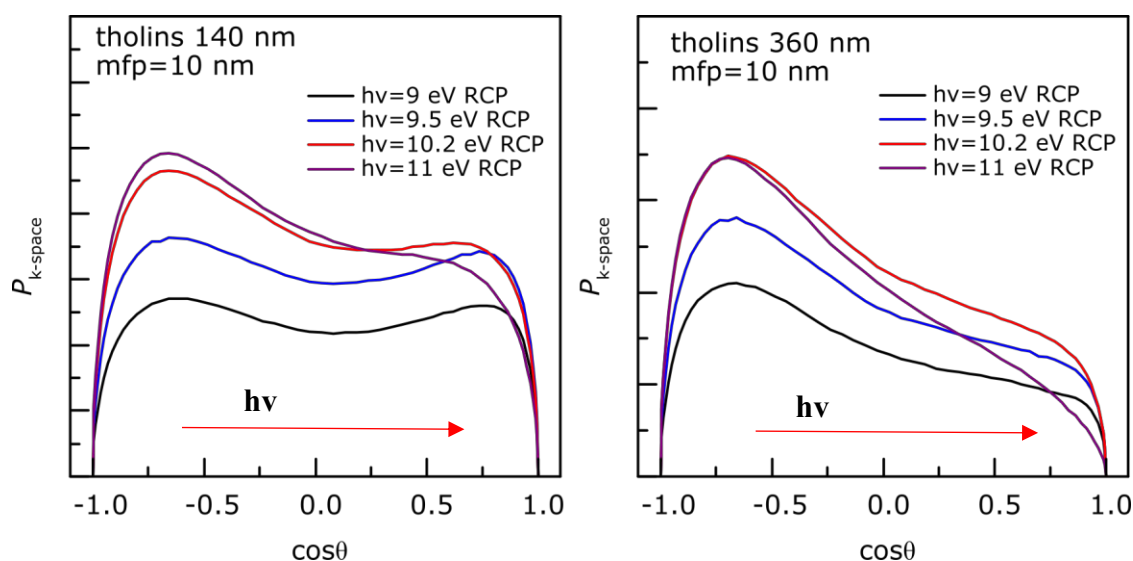
Figure 79. Distribution angulaire en \cos \theta de l'émission des photoélectrons dans l'espace des moments pour nos deux tailles de tholins et aux différentes énergies. Les asymétries sont ici clairement visibles. L'axe de propagation de la lumière est ici gauche \rightarrow droite.
