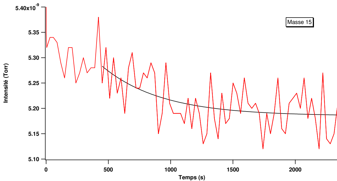
Figure 33. Suivi temporel du signal m/z 15 pour une irradiation à 58.4 nm. La courbe noire indique le fit exponentiel décroissant.
