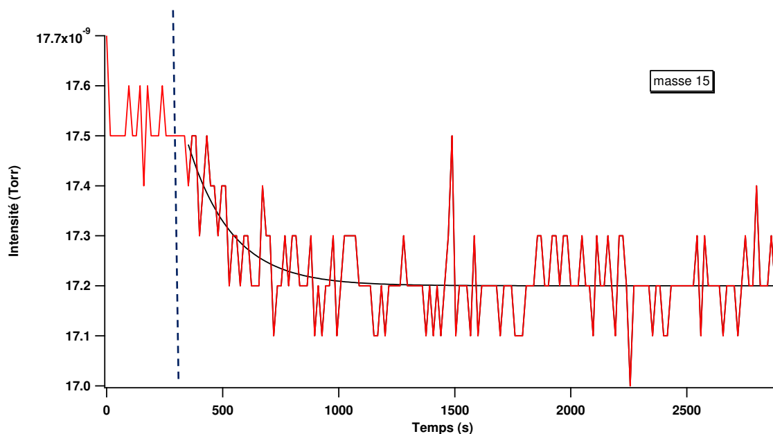
Figure 28. Suivi temporel du signal m/z 15, correspond au fragment du méthane CH_3^+ , pour une irradiation à 73.6 nm. On observe bien une diminution, donc une consommation du réactif durant l'irradiation avec un état stationnaire final. La barre bleue verticale et pointillée indique le début de l'irradiation VUV. La courbe noire représente le fit trouvé avec le logiciel IGOR.
