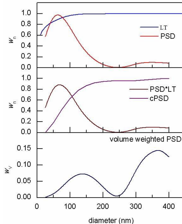
Figure 76. De haut en bas : (1) distribution en taille des tholins étudiés (rouge) et transmission de la lentille aérodynamique (bleu). (2) Distribution en taille pondérée par la transmission de la lentille (rouge foncé) et distribution en taille cumulée (violet). (3). Distribution en volume des tholins
