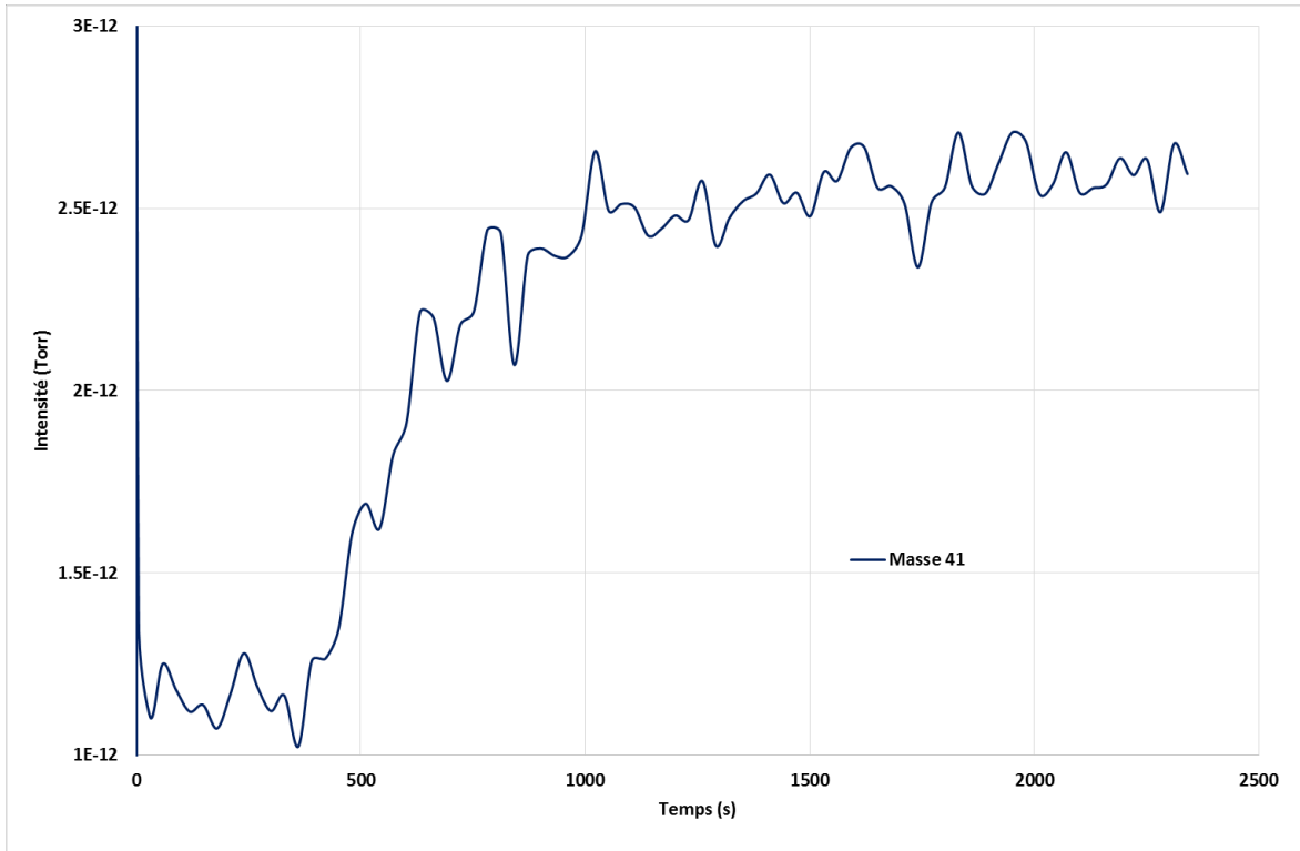
Figure 36. Suivi MID de la masse m/z 41 pour une irradiation à 58.4 nm.
