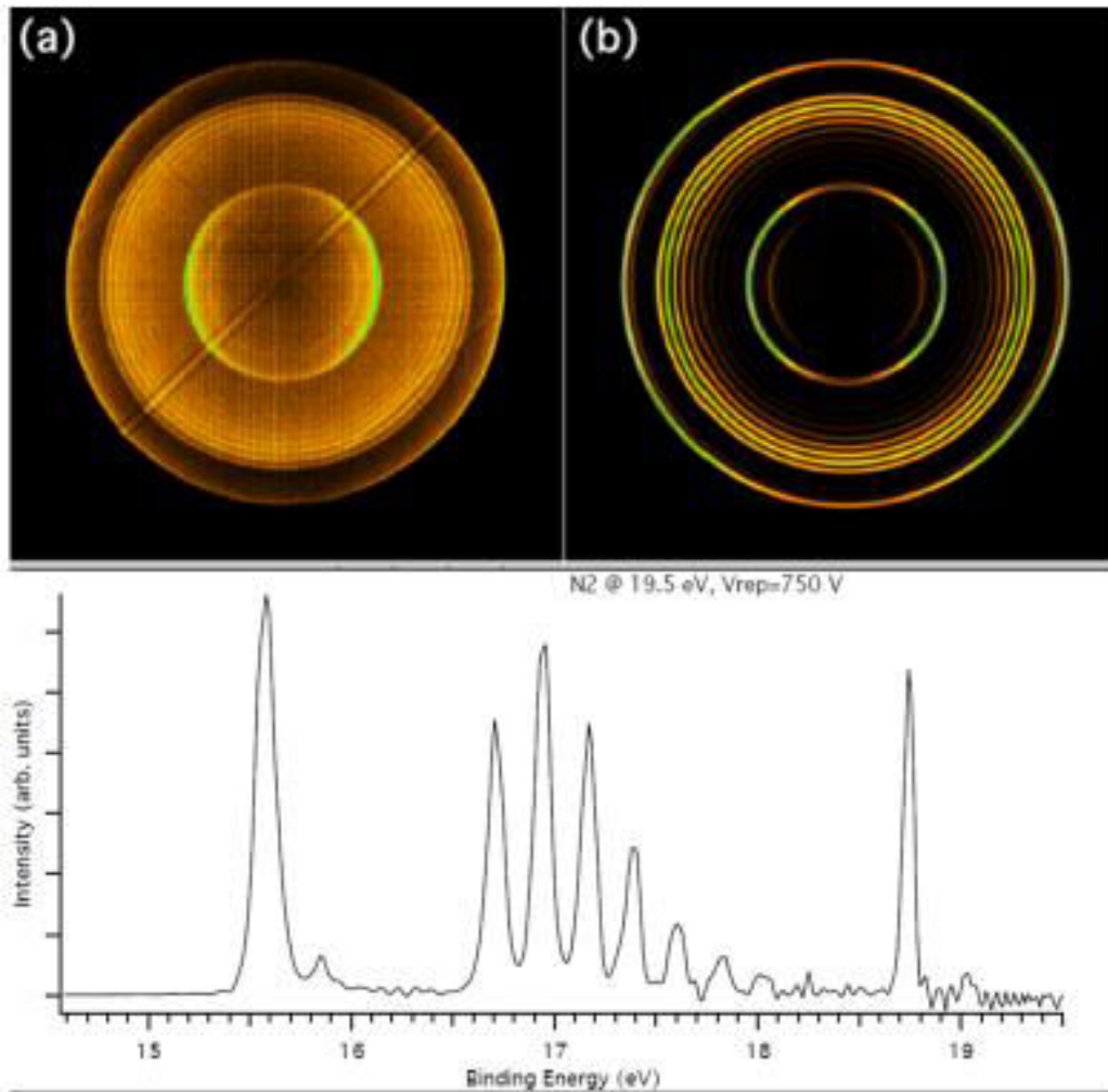
Figure 60. Image brute (haut, gauche) et inversée par transformée d'Abel (pBasex) (haut, droite) de la photoionisation de N_2 à 19.5 eV. Chaque impact des photo-électrons sur le détecteur dépend de leur énergie cinétique. Il s'agit d'une projection en 2D d'une sphère d'émission en 3D. La polarisation est linéaire horizontale dans le plan du détecteur ce qui permet d'inverser les images (symétrie cylindrique autour du vecteur polarisation). En bas : PES de N_2 obtenu par intégration angulaire de l'image inversée.
