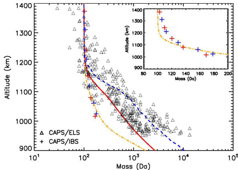
Figure 45. Evolution de la taille des ions négatifs lourds (triangles) en fonction de l'altitude mesurée par l'instrument CAPS/ELS. Les croix dans l'encadré représentent les ions positifs (Lavvas et al. 2013).
