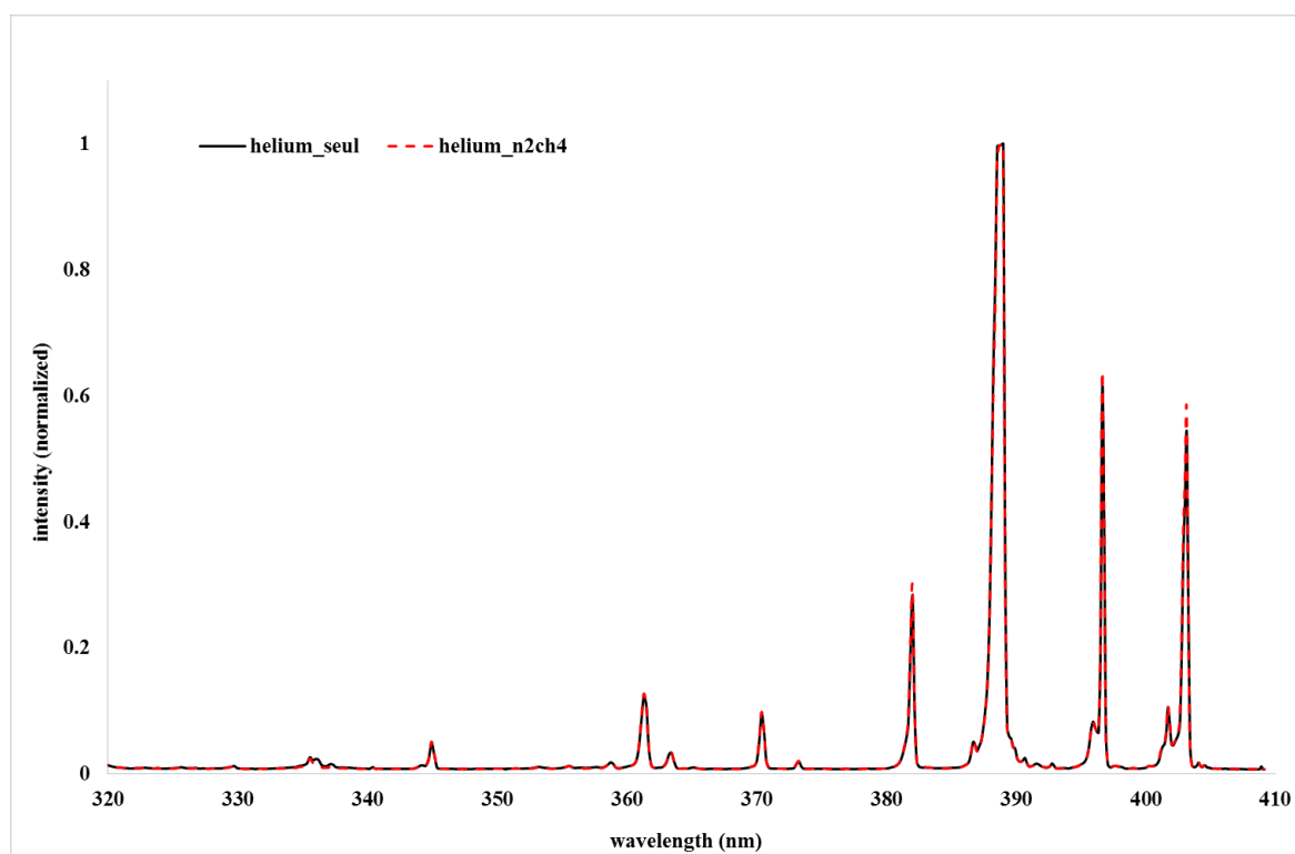
Figure 23. Spectre d'émission UV de l'hélium seul (courbe noire) puis de l'hélium face au mélange N_2 - CH_4 dans les conditions d'utilisation pour de la photochimie sur APSIS (courbe rouge pointillée). La superposition des courbes est parfaite. L'intensité est normalisée.
