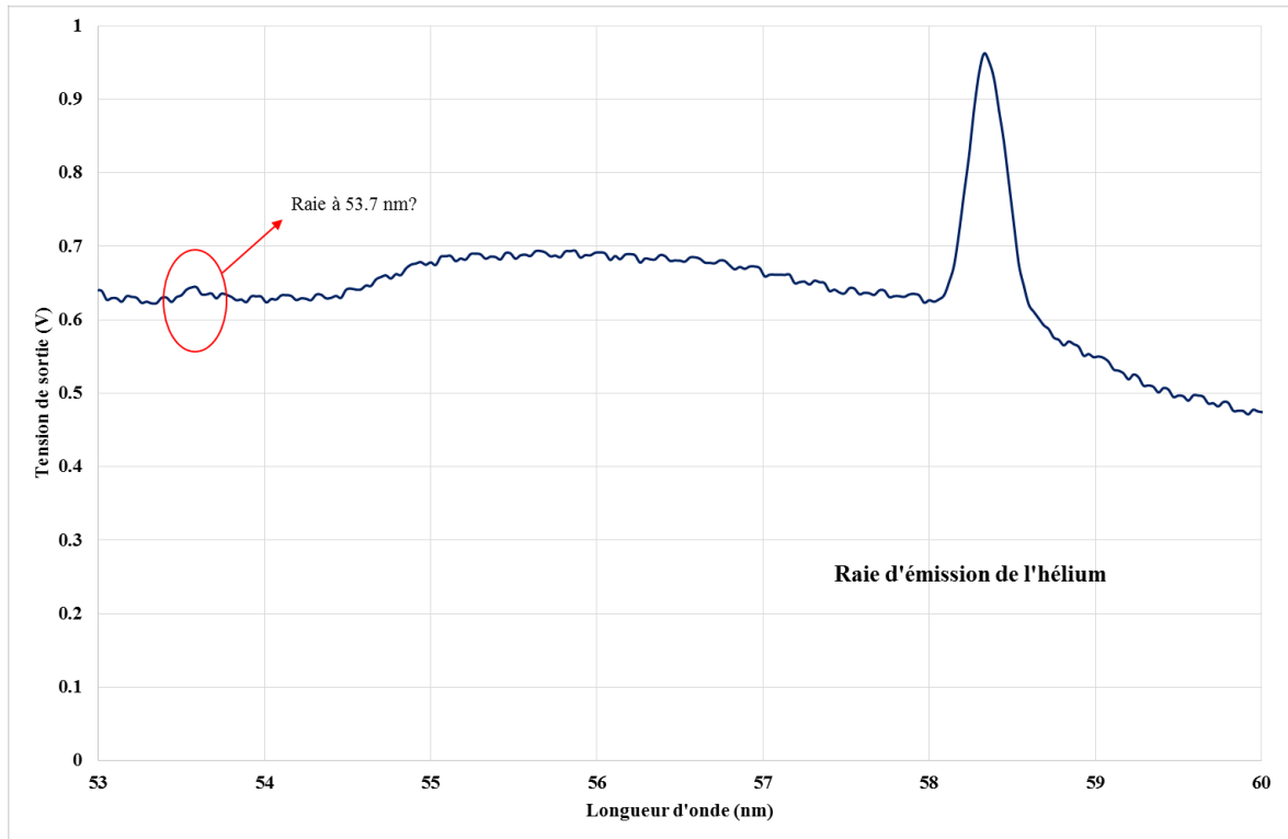
Figure 22. Spectre de la raie d'émission de l'hélium à 58.4 nm. Le signal de l'autre raie de résonance se devine à peine à 53.7 nm. On remarque aussi la déformation de la ligne de base, qui n'apparaît que pour des longueurs d'onde inférieures à 70 nm, et reste à date inexpliquée. Cependant, elle ne perturbera pas les mesures d'intensité des raies dans notre étude.
