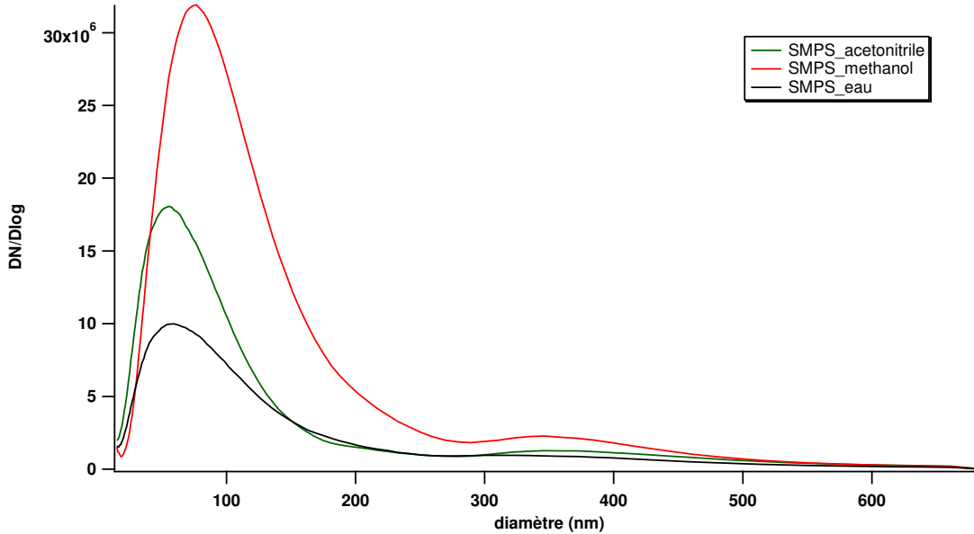
Figure 53. Distributions en taille des tholins à 5% de méthane obtenues par SMPS avec différents solvants pour la mise en solution initiale : l'eau (courbe noire), le méthanol (rouge) et l'acétonitrile (vert).
