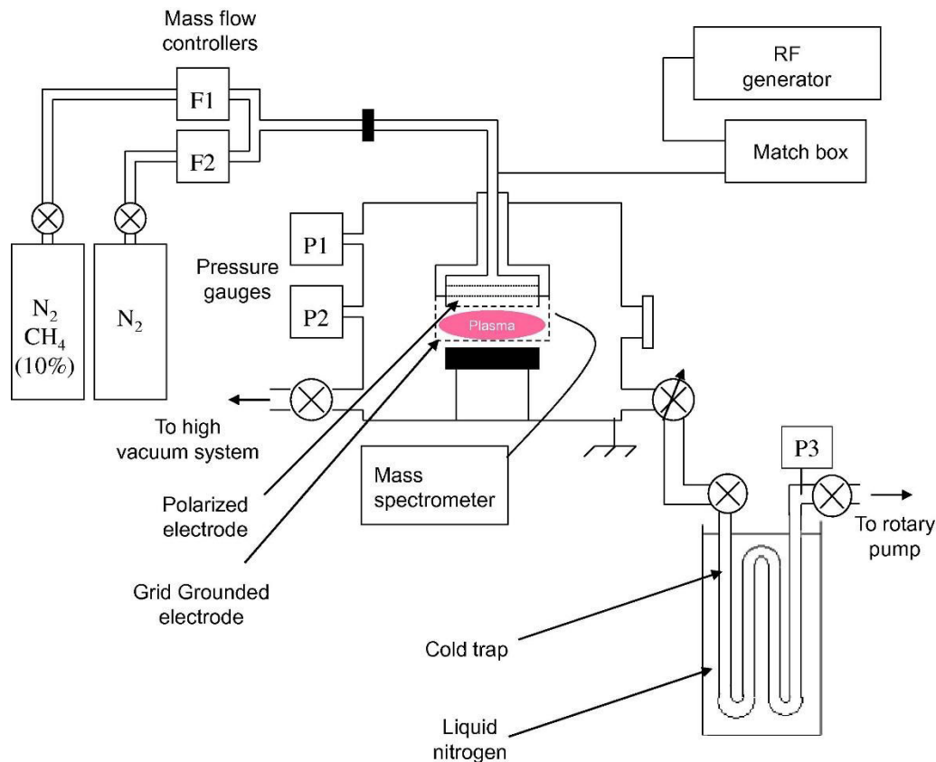
Figure 9. Schéma de l'expérience PAMPRE et de ses différents diagnostics.
