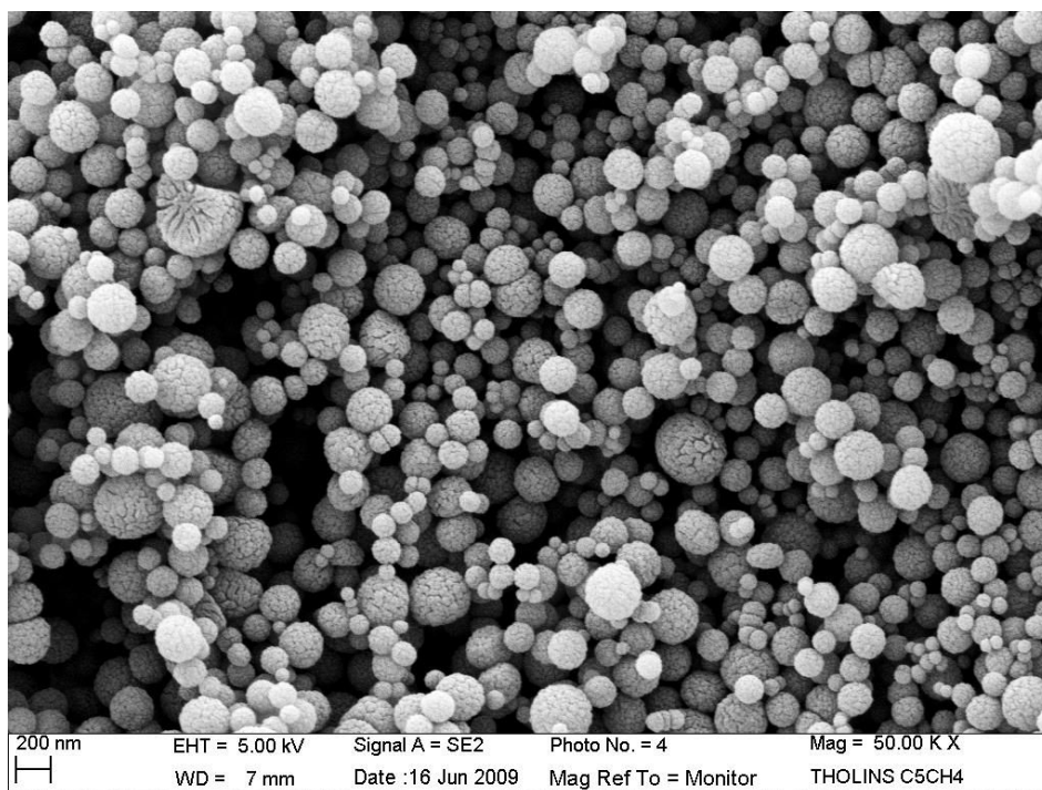
Figure 49. Photographie des tholins de PAMPRE à 5% de méthane prise au microscope électronique à balayage (communication personnelle d'E. Hadamcik).
