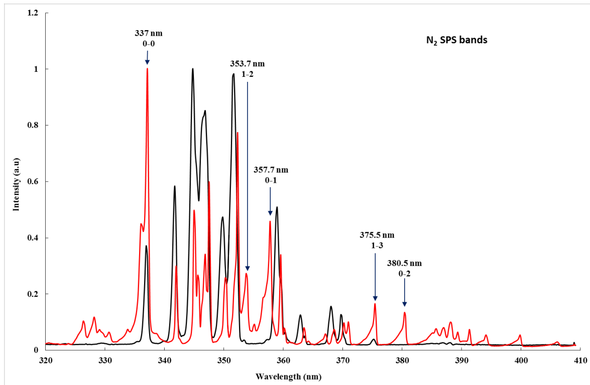
Figure 18. Spectre d'émission du néon dans l'UV (courbe noire), toutes les raies observées sont répertoriées dans la base de données du NIST. En rouge, nous avons le même spectre, mais avec ici le plasma qui pénètre intentionnellement le réacteur APSIS : nous pouvons alors identifier les bandes du SPS de l'azote moléculaire. L'échelle est ici normalisée.
