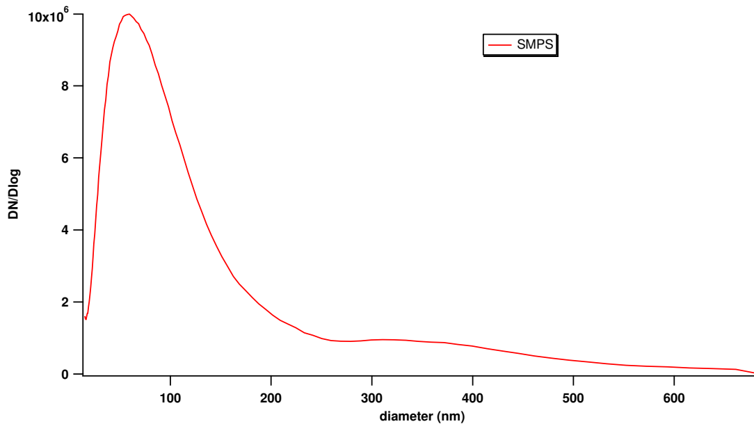
Figure 52. Distribution en taille des tholins obtenue par la méthode SMPS.
