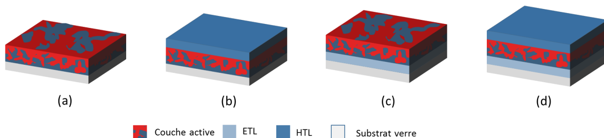
Figure n° IV-9: Architectures étudiées pour le suivi du spectre d'absorption de la couche active HBG1:PC 61 BM
