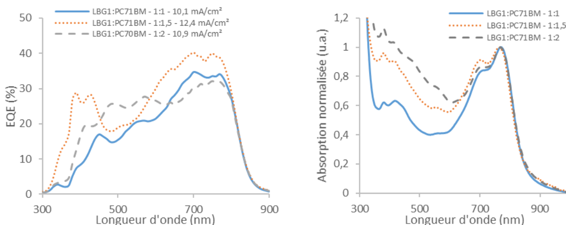
Figure n° III-18 : Mesures EQE (à gauche) et spectre UV-Visible du couple LBG1:PC 71 BM à différents ratio D:A
