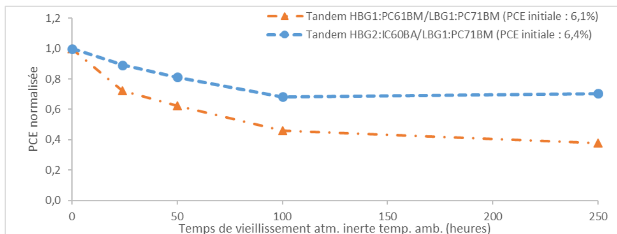
Figure n° IV-29 : Evolution des performances des deux sous-cellules sous illumination continue AM1.5G 1000 W/m 2 , température ambiante et atmosphère inerte
