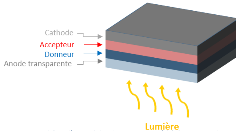
Figure n° I-5: Schéma d'une cellule solaire organique à hétérojonction planeaire
