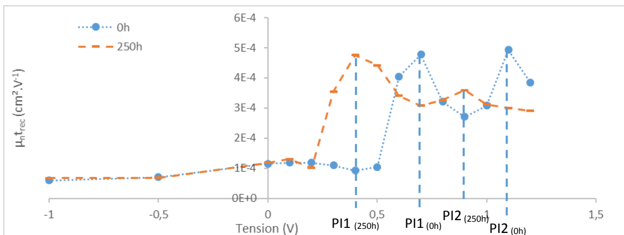
Figure n° IV-40 : Evolution du produit \mu_n t_{rec} d'une cellule tandem HBG1:PC61BM/LBG1:PC71BM en fonction de la tension à 0h et 250h de vieillissement
