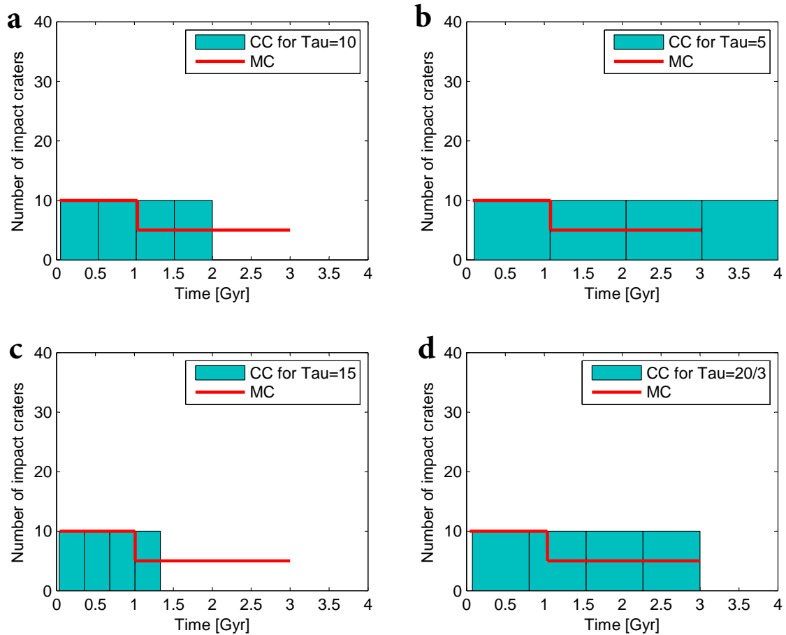
FIGURE 3.14 – Résultats sur le control clock (histogramme bleu) où un flux d'impact variant d'un facteur 2 entre l'intervalle [0 1 Ga] et [1 3 Ga] a été simulé (courbe rouge). La valeur du paramètre \tau représentant la fonction de production est constant dans le temps. a : \tau est égal à 10, b : \tau est égal à 5, c : \tau est égal à 15, d : \tau est égal \frac{20}{3} . Dans ce dernier cas, le control clock est constant entre 0 et 3 Ga. Cependant, aucun des modèles où \tau est modifié mais constant dans le temps ne permet de retrouver le model clock.
