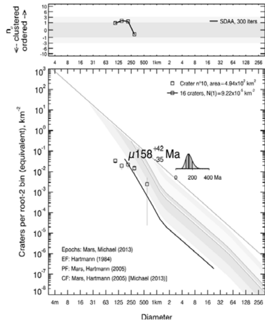
Datation du cratère n°10.
