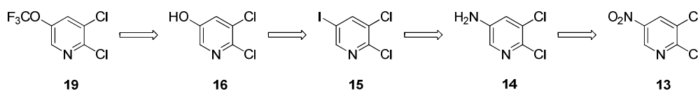
Figure 7: Schéma rétrosynthétique de la préparation de la OCF 3 -« Magic Pyridine »
