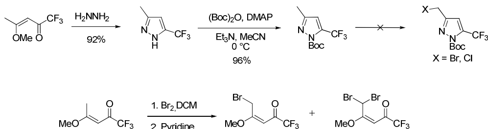
Schéma 12 : Tentatives de bromation de précurseurs et de pyrazoles protégés
