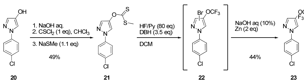
Schéma 3: Préparation d'une 4-OCF 3 pyrazole
