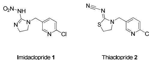
Figure 3: Structures de l'Imidaclopride et de la Thioclopride
