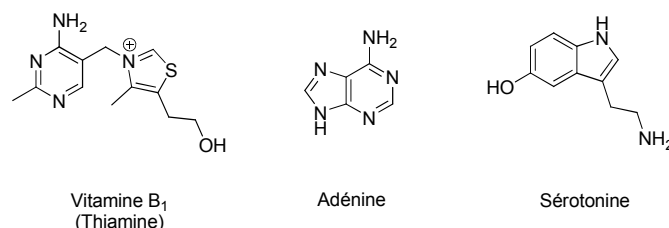
Figure 2: Produits naturels hétérocycliques impliqués dans des processus biologiques
