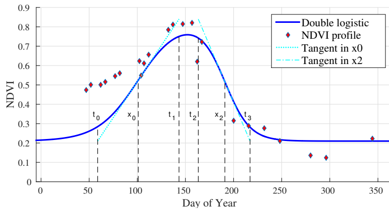
FIGURE 4.2 – Modélisation d'un profil de Normalized Difference Vegetation Index (NDVI) par une double logistique.
