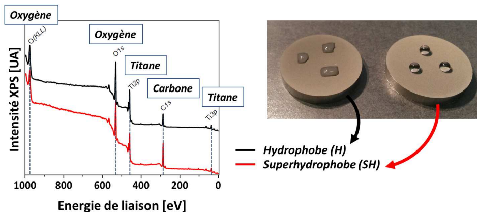
Figure 8.10: Spectres de balayage global obtenu par XPS d'échantillons de titane texturés par laser et stockés dans des environnements différents : le disque de gauche tout juste hydrophobe (H) a été laissé à l'air libre, tandis que celui de droite superhydrophobe (SH) a été placé dans un sachet de polyéthylène.
