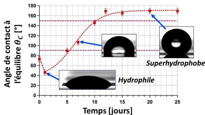
Figure 8.1: Evolution temporelle de la mesure de l'angle de contact à la surface de référence ( \lambda = 1030 \text{ nm} , \tau_{imp} = 300 \text{ fs} , \nu_{rép} = 50 \text{ kHz} , F_0 \approx 1,1 \text{ J/cm}^2 , V_{scan} = 75 \text{ mm/s} , h = 30 \mu\text{m} et 10 passes). Juste après texturation laser, l'angle de contact chute de 75^\circ à 50^\circ , avant de croître selon une courbe sigmoïde jusqu'à atteindre une valeur de plus de 160^\circ .
