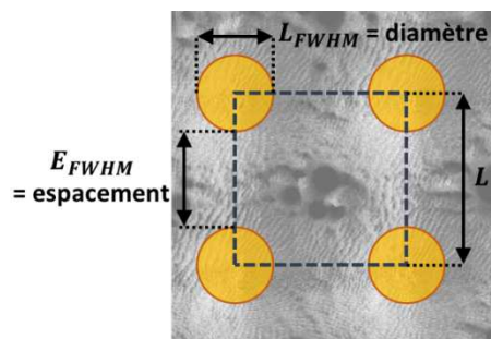
Figure 7.4: Représentation schématique du calcul de fraction de surface solide \phi_s dans le cas de la surface de référence.
