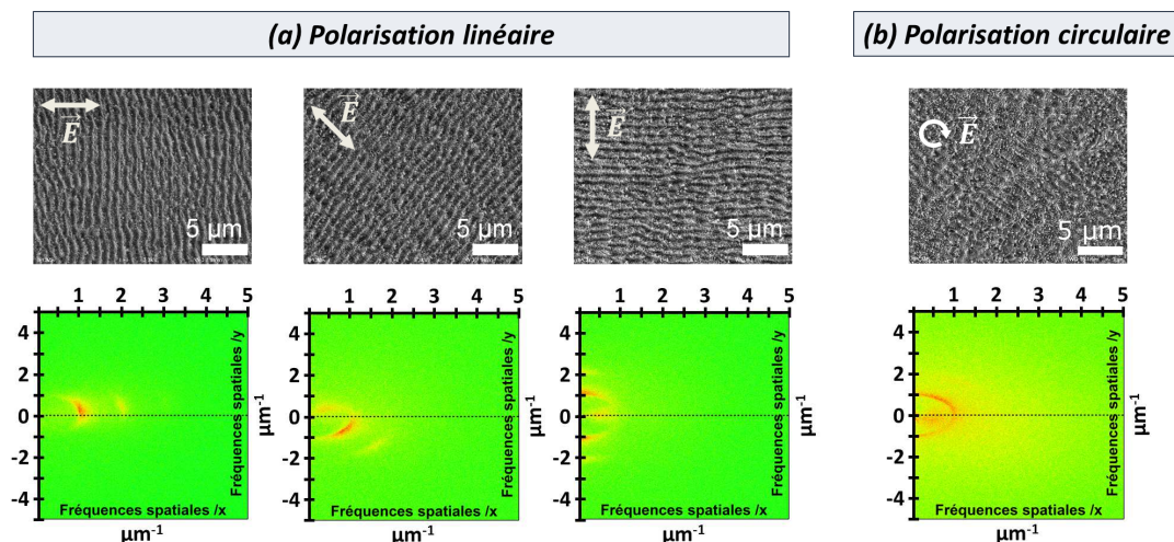
Figure 6.27 : (a) Images MEB de ripples avec différentes orientations de la lame demi-onde à 0^\circ , 30^\circ et 55^\circ , montrant alors un réseau orienté à \sim 90^\circ , \sim 45^\circ et \sim 180^\circ , et les différents spectres de FFT-2D associés. (b) Comparaison avec une image MEB et le spectre de ripples obtenus en polarisation circulaire, montrant une distribution plus circulaire des structures.
