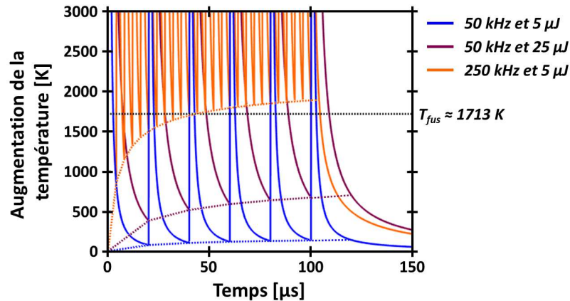
Figure 5.6: Evolution temporelle de l'augmentation de la température de la surface d'acier inoxydable, pour différents taux de répétition (50 et 250 kHz) et des énergies thermiques de 5 et 25 \mu\text{J} . L'enveloppe inférieure (en pointillés) de chaque courbe d'évolution montre les différentes augmentations de la température. A 50 kHz, la température augmente sans dépasser la température de fusion, tandis que l'accumulation thermique est clairement visible pour la fréquence de 250 kHz. Courbes reproduites à partir de [Weber et al. 2014].
