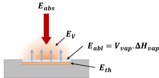
Figure 5.1: Schéma de la répartition de l'énergie absorbée E_{abs} par le matériau en trois parties : énergie E_{abl} pour ablater le matériau, énergie thermique E_V dans la vapeur et énergie thermique résiduelle E_{th} , inspiré de [Bauer et al. 2015].
