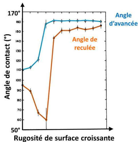
Figure 3.19: Expérience de Johnson et Dettre, montrant l'influence de la rugosité de la cire sur les valeurs des angles de contact et sur l'hystérésis [Dettre & Johnson 1964].
