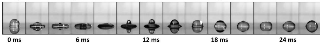
Figure 8.3: Photographies du rebond d'une goutte sur la surface d'acier inoxydable non texturée, pour une hauteur de chute de \sim 2 \text{ cm} , montrant l'ancrage de la goutte sur la surface.
