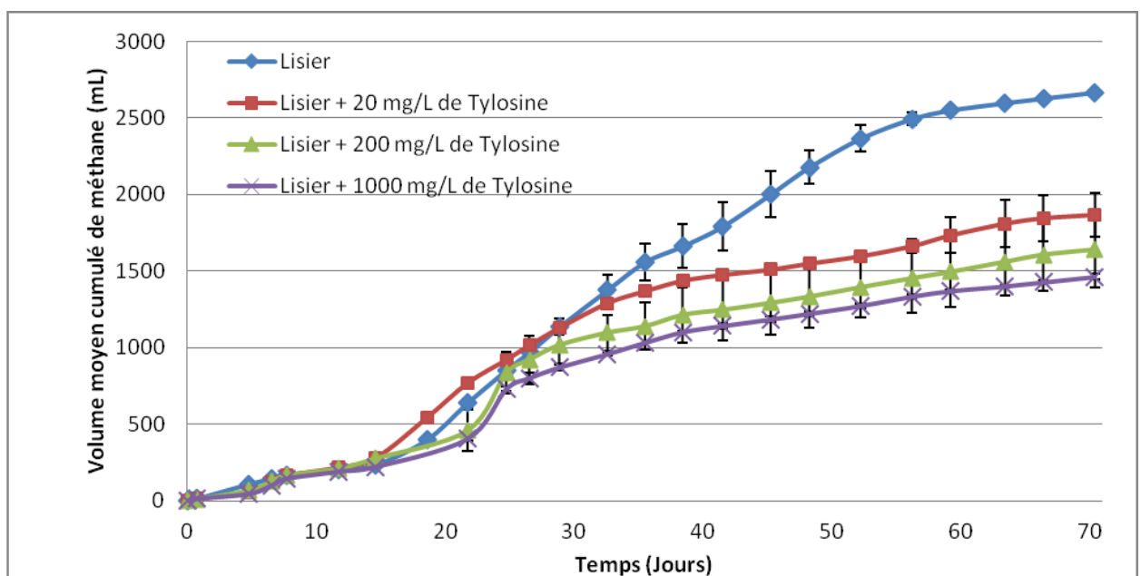
Figure IV.53 : Volume moyen cumulé de méthane pour les tests batch avec la tylosine
