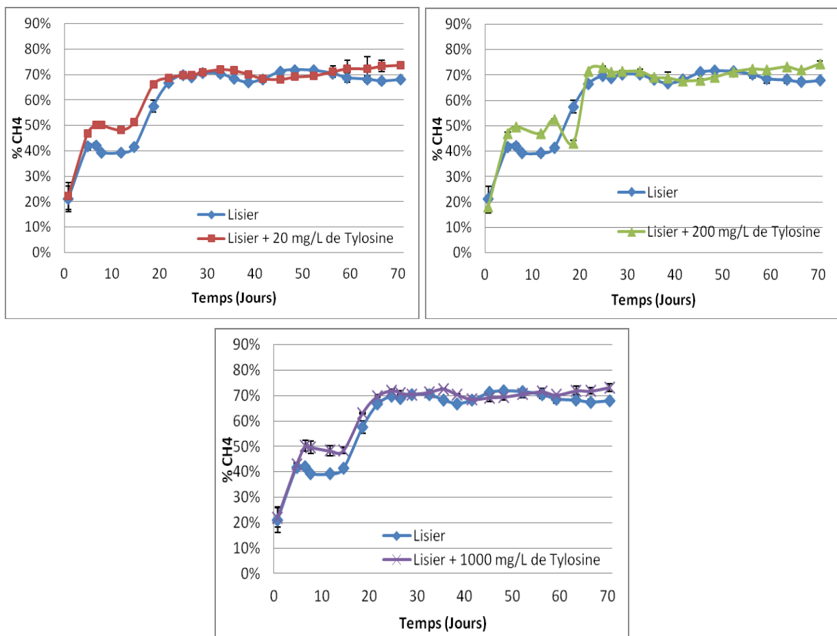
Figure IV.51 : Teneur en méthane des tests batch avec la tylosine
