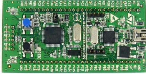
FIGURE 4.4 – Carte de développement STM32F100 utilisée pour nos tests
