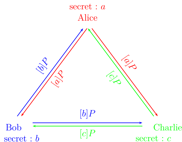
FIGURE 2.2 – Échange triparti en un tour
