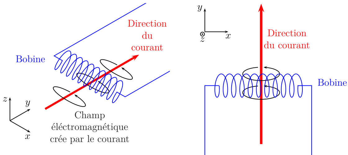
(a) Champ électromagnétique généré par le courant et capté par la bobine
