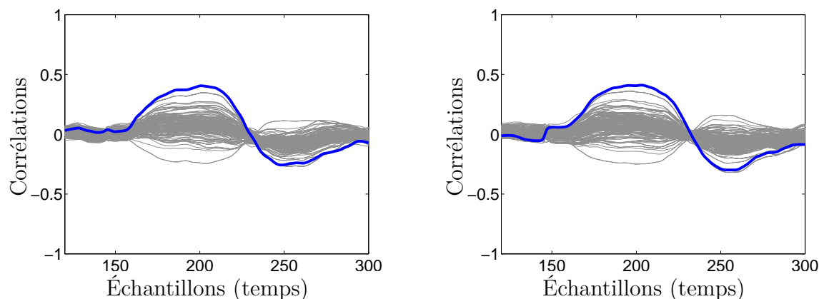
(a) CPA sur a_0 \times b_0 avec a_0 secret
