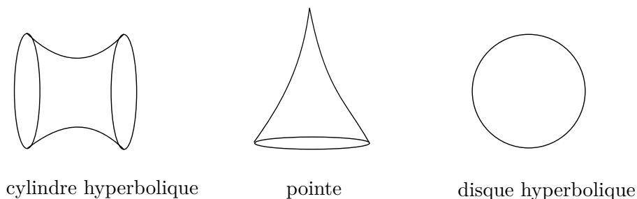
FIGURE 2.2 – exemples de surfaces hyperboliques élémentaires
