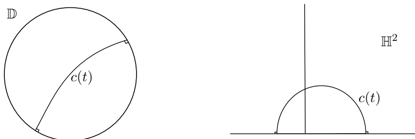
FIGURE 1.1 – géodésiques dans \mathbb{D} et \mathbb{H}
