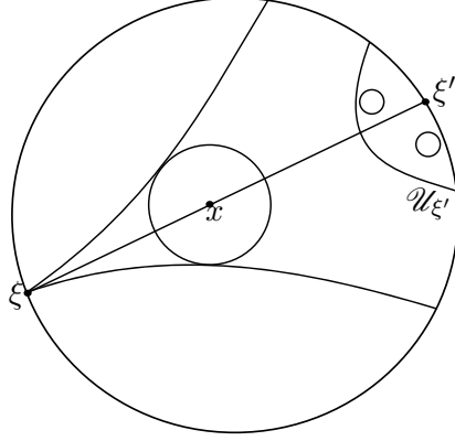
FIGURE 4.1 – Voisinage de \xi' dans \widetilde{M}
