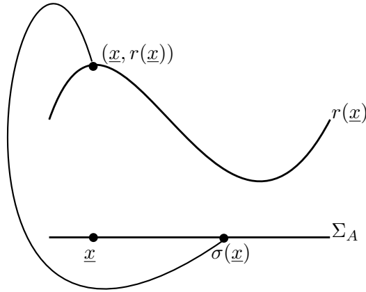
FIGURE 1.2 – Suspension au dessus d'un sous-décalage de type fini
