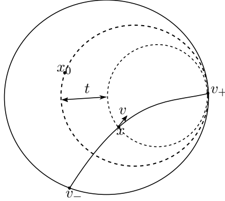
FIGURE 2.3 – coordonnées de Hopf
