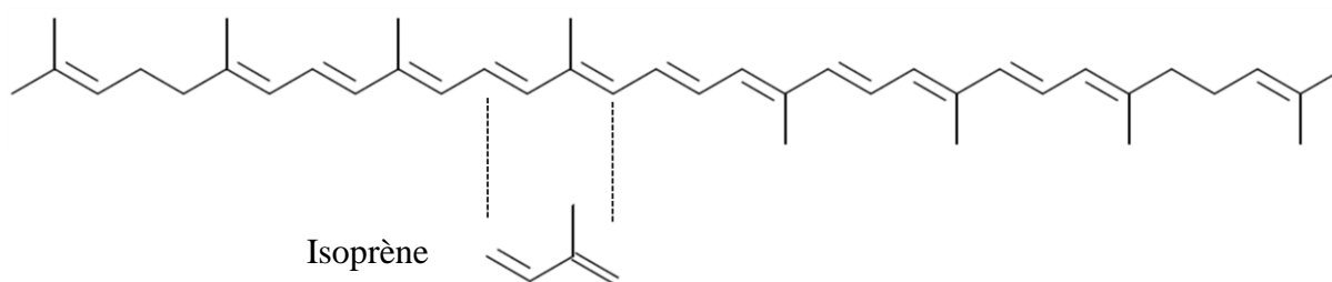
\beta -carotène
