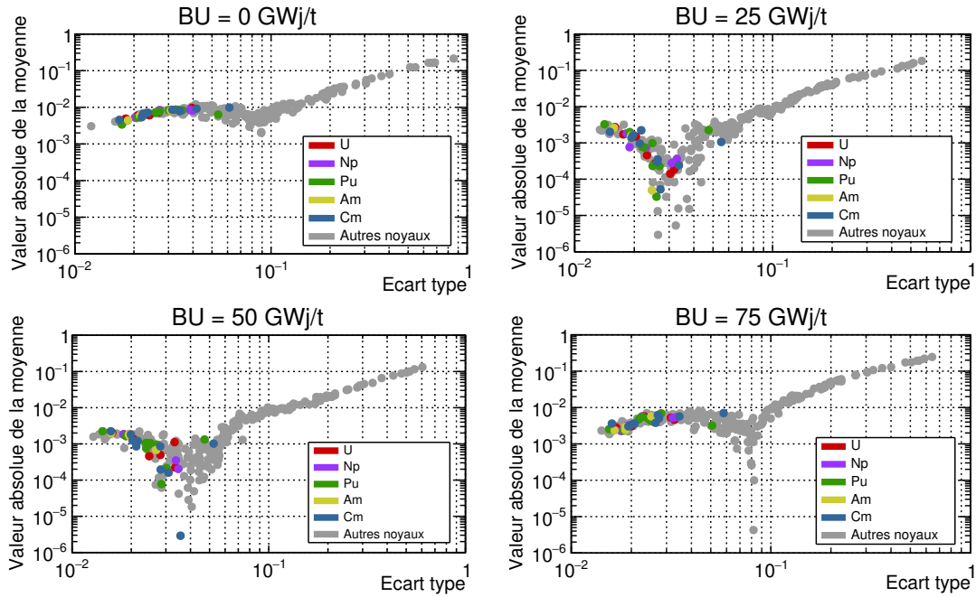
FIGURE 3.25 – Dispersion sur la reconstruction des sections efficaces moyennes (n,2n) par les PMC entraînés sur la BD_{0-16} et testés sur un échantillon de test appartenant à l'espace isotopique du combustible MOXEUS, pour 4 valeurs de burn-up : 0, 25, 50 et 75 GWj/t.
