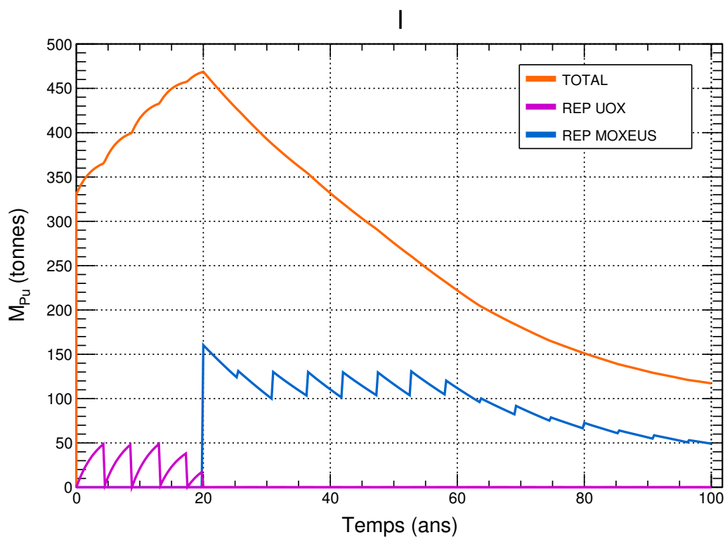
FIGURE 4.14 – Évolution de la masse totale de plutonium en cycle ( M_{Pu}^{TOTAL} ), dans le REP MOXEUS et dans le REP UOX dans les scénarios stabilisateur S_2 et incinérateur I . Dans ces scénarios, les stocks de plutonium sont organisés en gestion LiFo lors de la fabrication de combustible MOXEUS.
