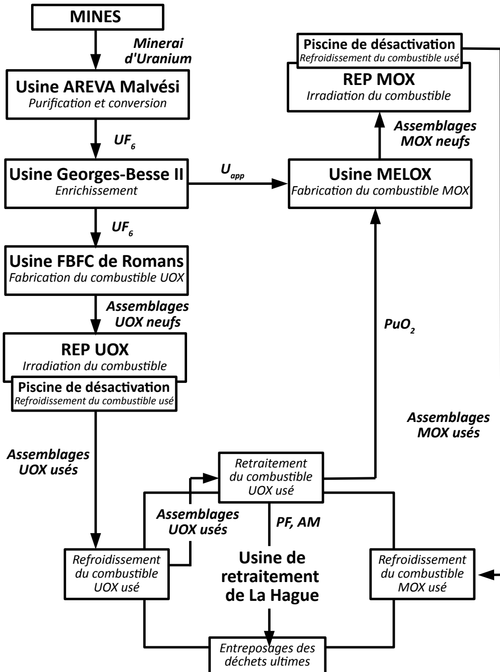
FIGURE 2.2 – Cycle du combustible nucléaire français
