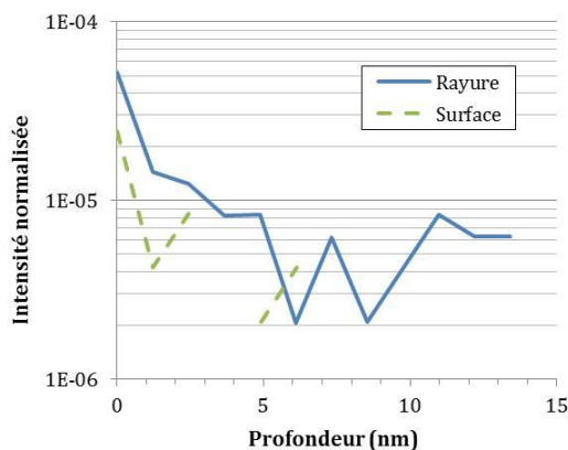
Figure 77 : Profils de pénétration en profondeur du fer dans la rayure et en surface après polissage MRF et traitement chimique léger <2\mu\text{m}</math>.
