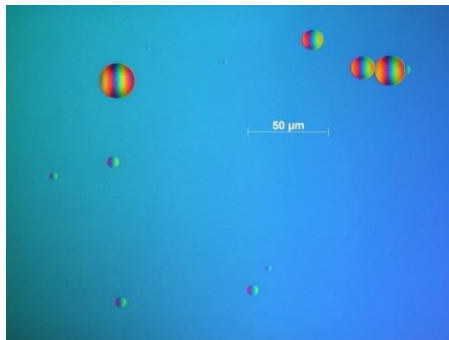
Figure 130 : Observation en microscopie optique des trous créés en surface par les traitements à base d' \text{HF}/\text{HNO}_3 .
