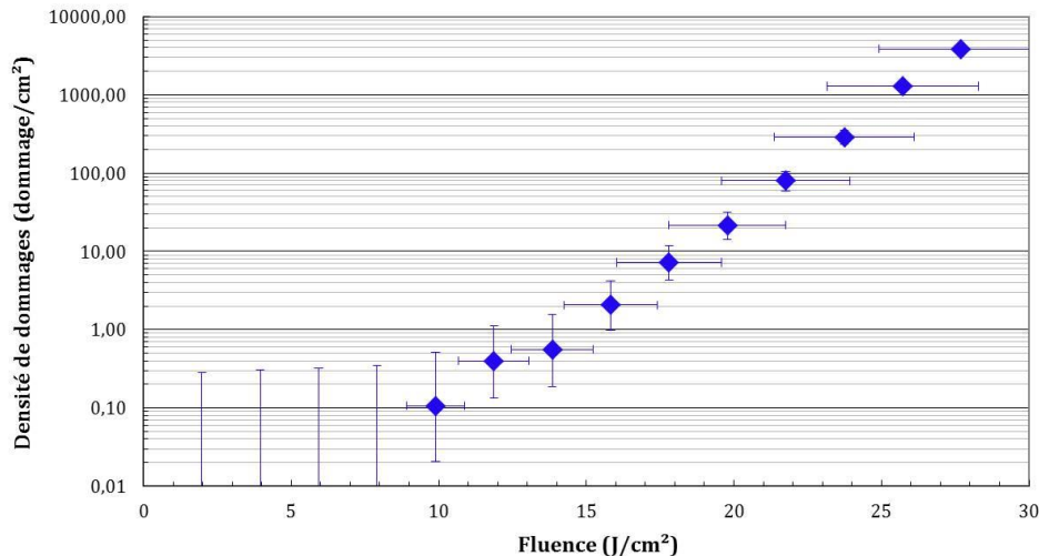
Figure 98 : Exemple de représentation de la tenue au flux laser en densité de dommages.
