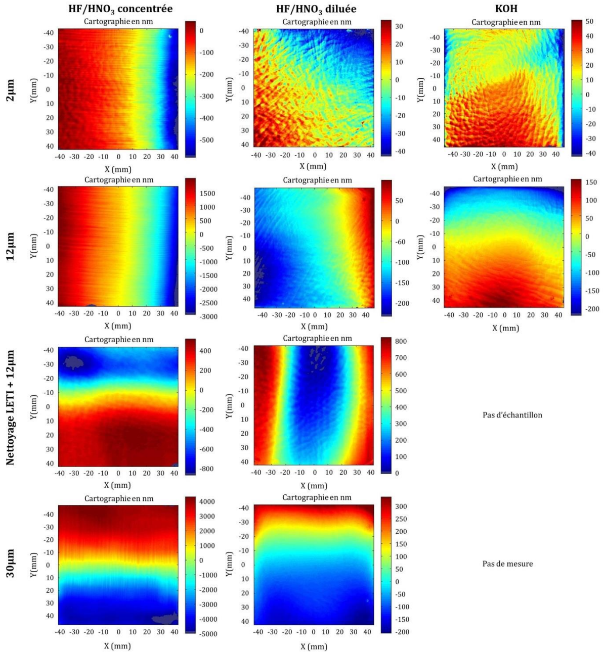
Figure 133 : Cartographies issues des mesures interférométriques d'égale épaisseur qui illustrent l'homogénéité de l'érosion en fonction des paramètres du traitement chimique.
