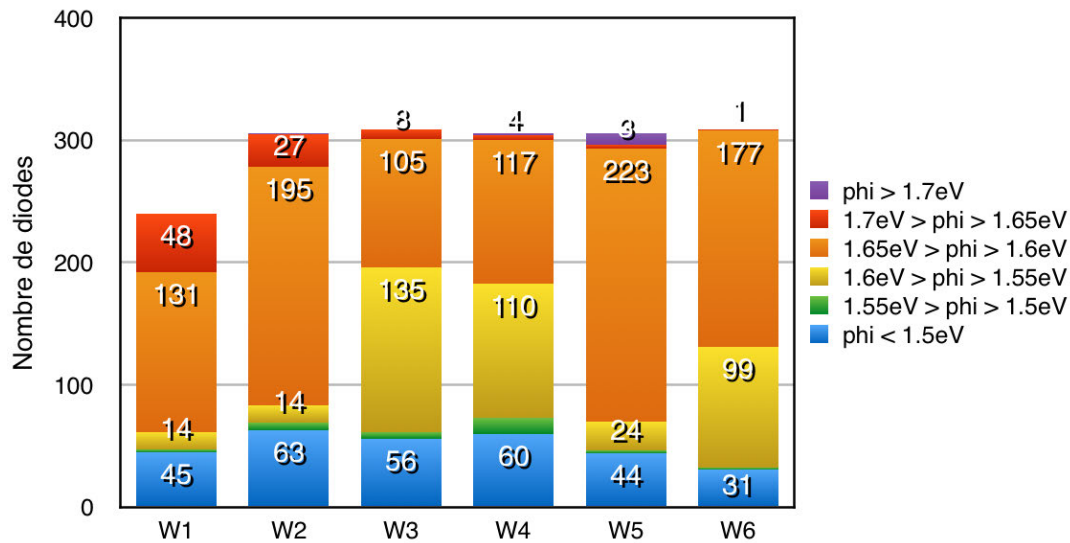
FIGURE 2.18 – Répartition de la hauteur de barrière par plaque du lot 6.
