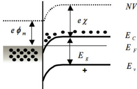
FIGURE 1.25 – Diagramme des bandes d'énergie du contact ohmique parfait sur un semiconducteur de type n [52].
