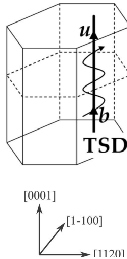
FIGURE 1.33 – Illustration de la dislocation de type “vis” du SiC[90].
