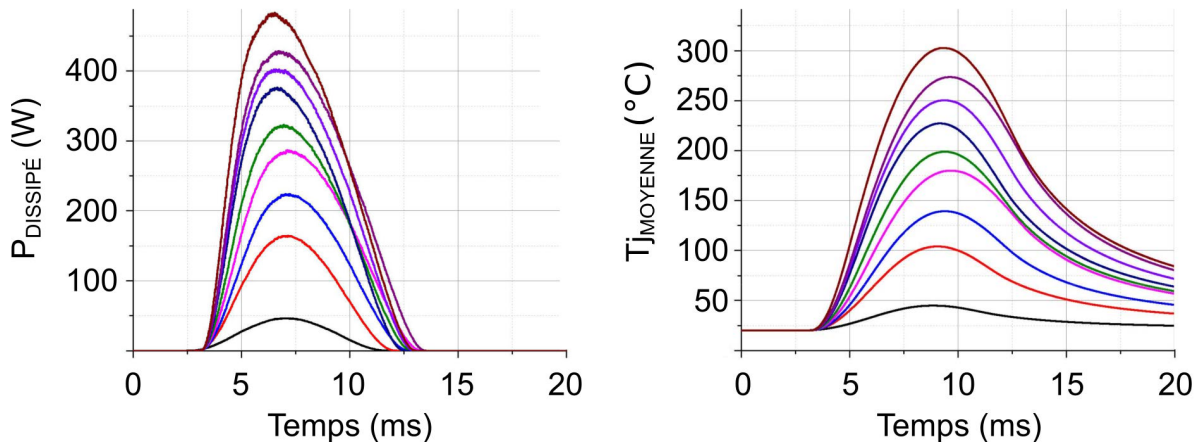
FIGURE 4.14 – Évolution de la puissance dissipée et de la température en fonction du temps pour la diode HL6.
