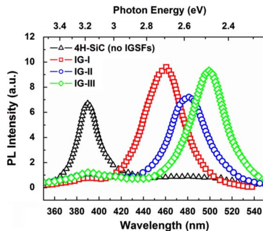
FIGURE 1.38 – Pics de photoluminescence du SiC-4H comparés à ceux des défauts d'empilement dans le substrat [97].
