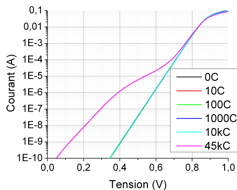
FIGURE 4.23 – Apparition de la double barrière suite aux tests en surcharge sur la diode de référence.
