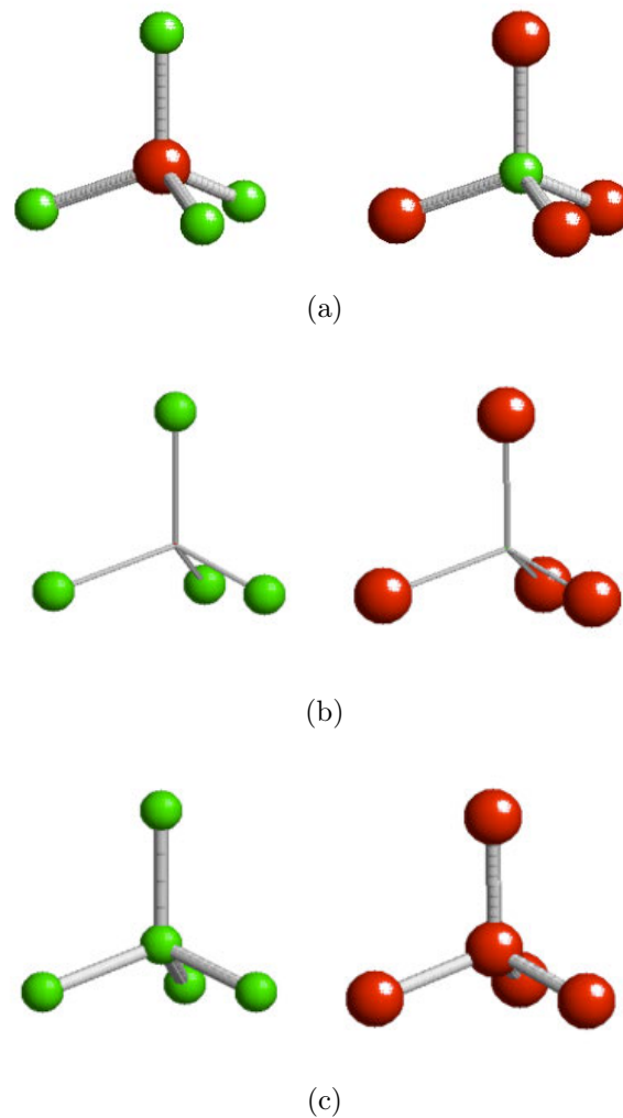
FIGURE 1.45 – Maille élémentaire du cristal SiC (a), lacune (b) et site substitutionnel (c)[104].
