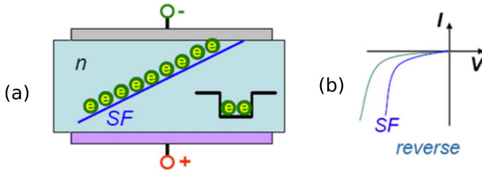
FIGURE 1.40 – Le niveau d'énergie du défaut engendre un puit de potentiel dans lequel les électrons sont piégés (a). La tenue de tension est influencée par le défaut d'empilement (b) [100].
