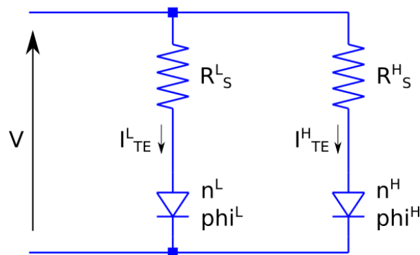
FIGURE 3.2 – Schéma électrique du modèle thermoïonique à double barrière.
