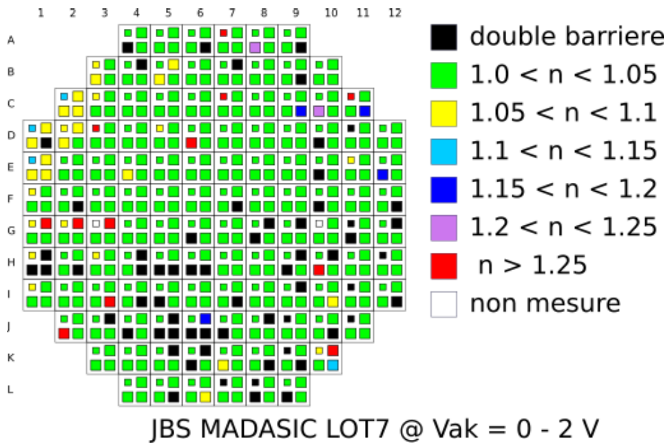
FIGURE 54 – Coefficient d'idéalité de la plaque BC1427-02DC4
