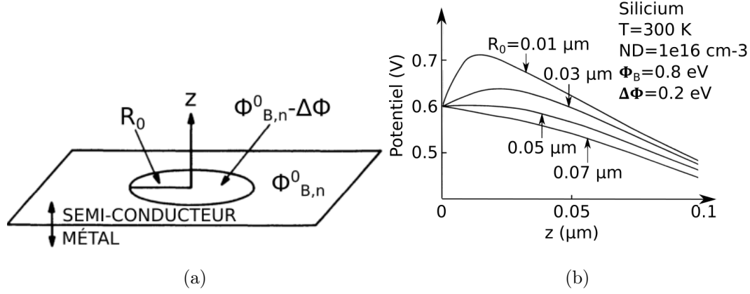
FIGURE 3.20 – La forme et les dimensions du contact Schottky de barrière basse influent sur l'effet de pincement (a). Simulation analytique du potentiel minimum de la bande de conduction d'une zone de barrière basse de rayon R_0 et de hauteur de barrière de 0.6 eV entourée d'un contact Schottky de 0.8 eV (b) [144].
