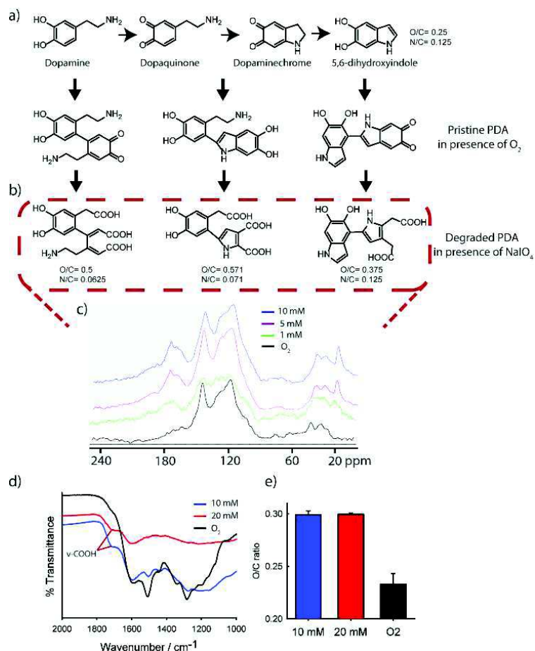
Figure 44 : a) Relations entre les différents monomère de départ, principaux précurseurs de PDA- \text{O}_2 . Composés structurels représentatifs de la dégradation de PDA en présence de périodate de sodium. C) Spectre RMN- \text{C}^{13} du solide de PDA- \text{O}_2 et PDA- \text{NaIO}_4 1, 5, et 10 mM. d) Spectre IR de poudres de PDA-SP et PDA- \text{O}_2 obtenu en solution après 22h en présence de SP et \text{O}_2 . e) Ratio atomique O/C obtenu d'après les analyses XPS des spectres de PDA-SP et PDA- \text{O}_2 .
