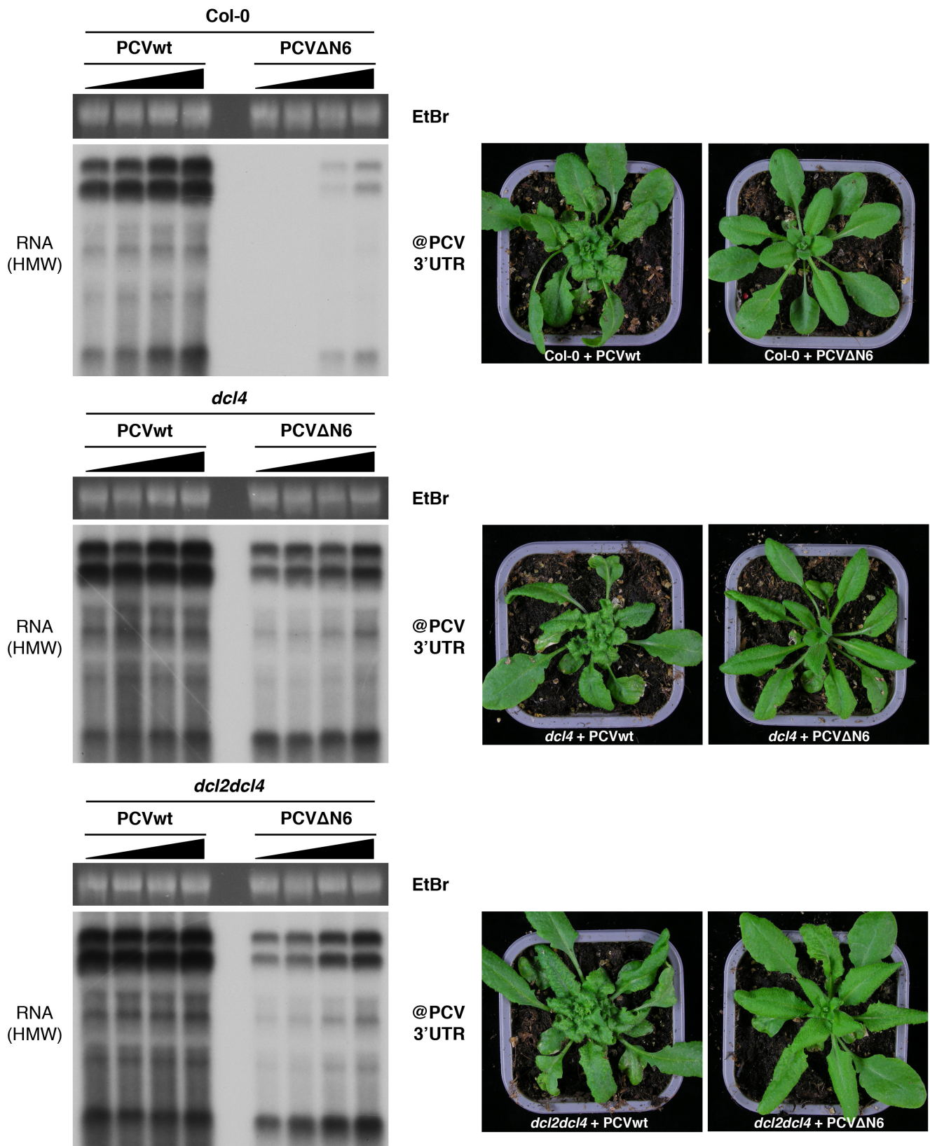
Figure 5: Impact sur le mouvement systémique du PCV de l'import des siARN dans les peroxisomes. (Figure 2.6 de la thèse)
