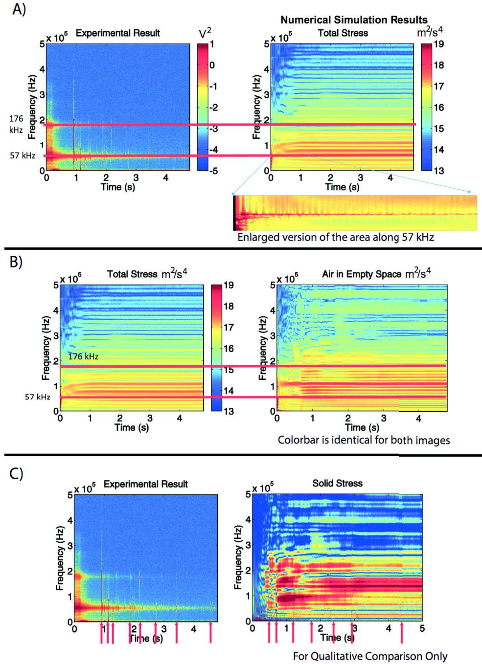
Figure 1.9: La comparaison de résultats des simulations numériques avec les données acquises pendant les expériences de même type. En A, on observe que les pics maximaux (lignes rouges) entre l'expérience et le modèle numérique ont la même fréquence. En B, on voit qu'on obtient les mêmes pics si on utilise uniquement la pression de l'air présente dans les canaux. En C, les flèches verticales rouges indiquent que l'on observe les mêmes structures des événements de type 2 entre l'expérience et la simulation numérique.
