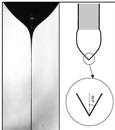
Figure 4: Taylor Cone [28, 29]
