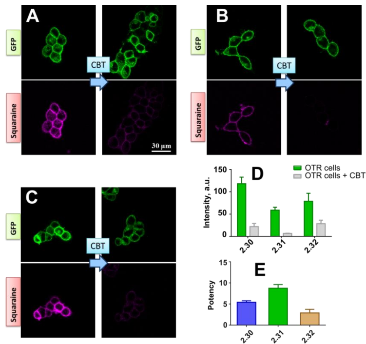
Figure R10. Images des cellules GFP-OTR avec 10 nM de 2.30 (A), 100 nM de 2.31 (B) et 10 nM de 2.32 (C) avant et après l'ajout de la carbécytocine non-modifiée. L'intensité de la fluorescence membranaire avant et après l'ajout de la carbécytocine (D) et la sensibilité des sondes (E).
