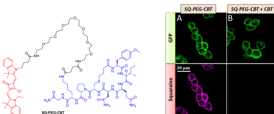
Figure R8. Structure du ligand turn-on basé sur la squaraine et images des cellules exprimant OTR fusionné à la GFP.
