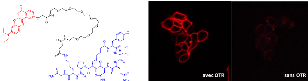
Figure R7. Structure du ligand turn-on basé sur le Nile Rouge et les images des cellules exprimant OTR.
