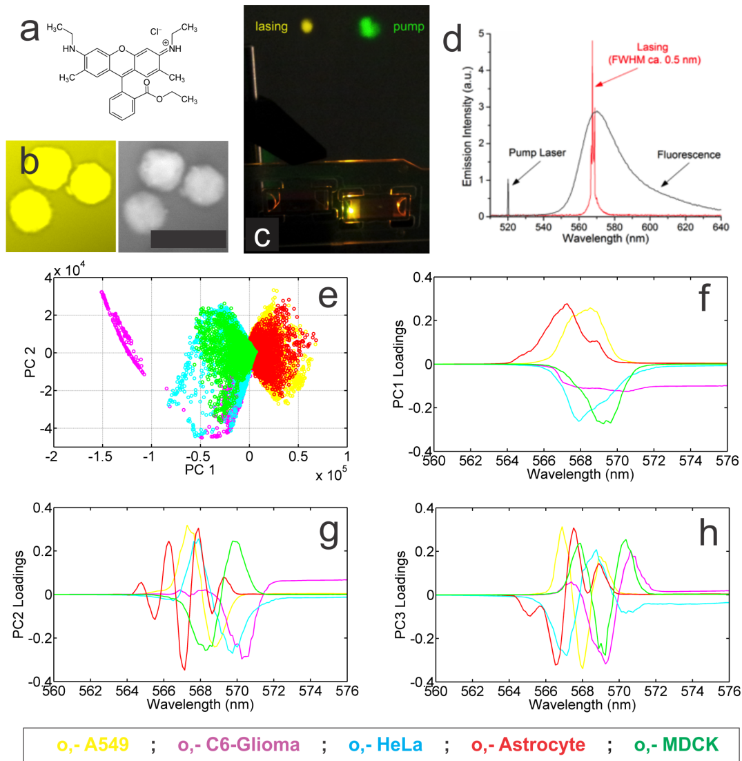
Fig. 2. a. Structure chimique du colorant rhodamine 6G. Micrographie au confocal à fluorescence de HeLa colorée à la R6G et image au champ clair correspondant. c. Vue
