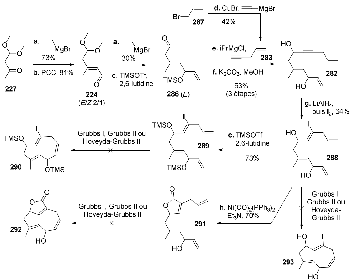
Schéma 58. Première tentative de cyclisation par métathèse. a. Bromure de vinylmagnésium, THF, -78^\circ\text{C} , 2 h, 227-I 73%, 224-I 30% ; b. PCC, \text{CH}_2\text{Cl}_2 , t.a., 48 h, 81% ; c. TMSOTf, 2,6-lutidine, \text{CH}_2\text{Cl}_2 , 0^\circ\text{C} , 1 h, puis \text{H}_2\text{O} , 0^\circ\text{C} , 15 min, 289 73% ; d. Bromure d'éthynylmagnésium, CuBr, THF, t.a., 2 h, 42% ; e. Alcyne 283 , \text{iPrMgCl} , THF, -78^\circ\text{C} , 1 h, 60% (2 étapes) ; f. \text{K}_2\text{CO}_3 , MeOH, t.a., 30 min, 89% ; g. \text{LiAlH}_4 , THF, reflux, 3 h, puis \text{EtOAc} , 0^\circ\text{C} , 15 min, puis \text{I}_2 , 0^\circ\text{C} , 1 h, 64% ; h. \text{Ni}(\text{CO})_2(\text{PPh}_3)_2 , \text{Et}_3\text{N} , toluène, reflux, 15 min, 70%. iPr = isopropyle ; PCC = chlorochromate de pyridinium ; TMS = triméthylsilyle ; Tf = triflyle.
