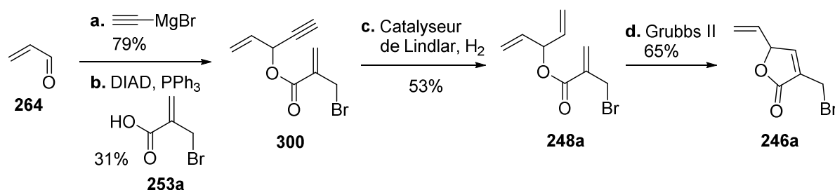
Schéma 61. Première synthèse de la bromolactone 246a . a. Bromure d'éthynylmagnésium, THF, t.a., 2 h, 79% ; b. Acide (2-bromométhyl)acrylique 253a , DIAD, \text{PPh}_3 , \text{Et}_2\text{O} , t.a., 12 h, 31% ; c. Catalyseur de Lindlar, \text{H}_2 , t.a., 12 h, \times 2 , 53% ; d. Grubbs II, \text{CH}_2\text{Cl}_2 , reflux, 3 h, 65%. DIAD = azodicarboxylate de diisopropyle.
