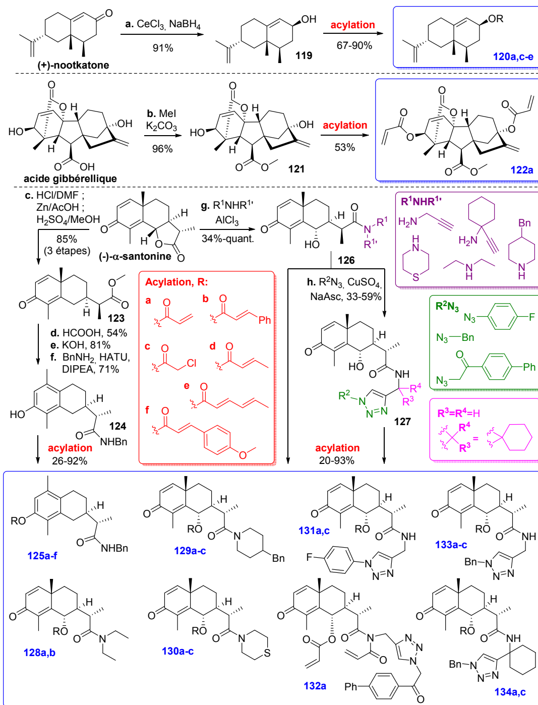
Schéma 23. Dérivatisation de la (+)-nootkatone, de l'acide gibbérellique et de la (-)-α-santonine. a. NaBH 4 , CeCl 3 , MeOH, t.a., 10 min, 91% ; b. K 2 CO 3 , MeI, acétone, t.a., 12 h, 96% ; c. HCl, DMF, 90 °C, 4 h ; Zn, AcOH, MeOH, reflux, 15 min ; H 2 SO 4 , MeOH, reflux, 2 h, 85% (3 étapes) ; d. HCOOH, reflux, 12 h, 54% ; e. KOH, EtOH, t.a., 12 h, 81% ; f. HATU, DIPEA, BnNH 2 , DMF, t.a., 12 h, 71% ; g. R 1 NHR 1' , AlCl 3 , DCE, t.a., 12 h, 34%-quant. ; h. R 2 N 3 , CuSO 4 , NaAsc, TBTA, DMF/H 2 O, t.a., 12 h 33-59%. Asc = ascorbate ; Bn = benzyle ; DCE = 1,2-dichloroéthane ; DIPEA = diisopropyléthylamine ; HATU = hexafluorophosphate de 3-oxyde-1-[bis(diméthylamino)méthylène]-1H-1,2,3-triazolo[4,5-b]pyridinium ; TBTA = tris[(1-benzyl-1H-1,2,3-triazol-4-yl)méthyl]amine.
