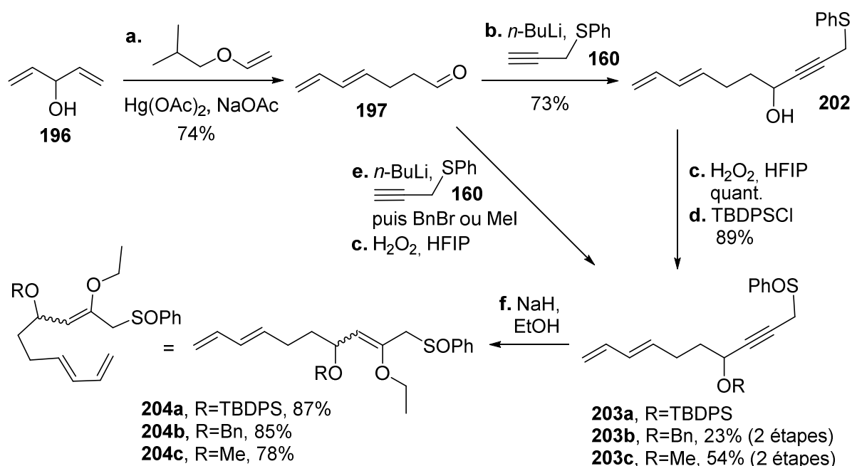
Schéma 39. Synthèse du substrat fonctionnalisé 204 . a. \text{Hg}(\text{OAc})_2 , NaOAc, isobutyl vinyl ether, reflux, 12 h, 74% ; b. Alcyne 160 , n\text{-BuLi} , \text{Et}_2\text{O} , -78^\circ\text{C} , 2 h, 73% ; c. \text{H}_2\text{O}_2 , HFIP, t.a., 30 min, 202-I quant., 203b 76%, 203c quant. ; d. TBDPSCl, imidazole, \text{CH}_2\text{Cl}_2 , t.a., 12 h, 89% ; e. Alcyne 160 , n\text{-BuLi} , \text{Et}_2\text{O} , -78^\circ\text{C} , 2 h, puis BnBr ou MeI, t.a. 12-24 h, 197b-I 30%, 197c-I 54% ; f. NaH, THF/EtOH, t.a., 30 min, 204a 87%, 204b 85%, 204c 78%. n\text{-Bu} = n -butyle ; HFIP = hexafluoroisopropanol ; TBDPS = tert -butyldiphénylsilyle ; Bn = benzyle.
