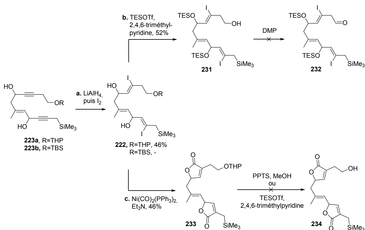
Schéma 46. Tentatives de synthèse du substrat de cyclisation. a. \text{LiAlH}_4 , THF, reflux, 3 h, puis \text{EtOAc} , 0 °C, 15 min, puis \text{I}_2 , 0 °C, 1 h, 46%. b. \text{TESOTf} , 2,4,6-triméthylpyridine, \text{CH}_2\text{Cl}_2 , 0 °C, 1 h, puis \text{H}_2\text{O} , 0 °C, 15 min, 52% ; c. \text{Ni}(\text{CO})_2(\text{PPh}_3)_2 , \text{Et}_3\text{N} , toluène, reflux, 1 h, 46%. DMP = périodine de Dess-Martin ; PPTS = para -toluènesulfonate de pyridinium ; TBS = tert -butyldiméthylsilyle ; TES = triéthylsilyle ; THP = tétrahydropyranyle ; Tf = triflyle.
