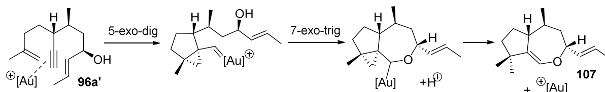
Schéma 19. Schéma réactionnel proposé pour la formation de 107 par action de [\text{AuPPh}_3]\text{OTf} .
