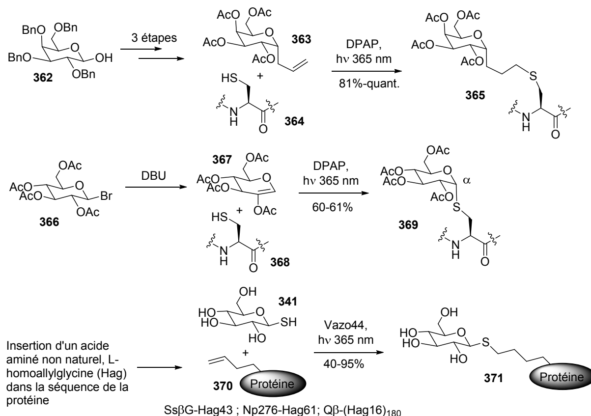
Schéma 76. Exemples de synthèse de S-glycopeptides par couplage thiol-ène. DBU = 1,8-diazabicyclo[5.4.0]undéc-7-ène ; DPAP = 2,2-diméthoxy-2-phénylacétophénone ; Vazo44 = dihydrochlorure de 2,2'-azobis[2-(2-imidazolin-2-yl)propane].
