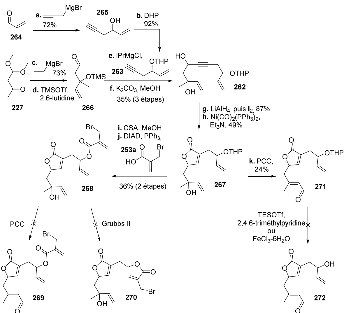
Schéma 55. Tentatives de synthèse du substrat de cyclisation pour l'allylation en 6-7. a. Bromure de propargyle, Mg, HgCl 2 , I 2 , Et 2 O, reflux vers t.a., 2 h, puis acroléine 264 , -78 °C, 1 h, 72% ; b. DHP, PPTS, CH 2 Cl 2 , t.a., 1 h, 92% ; c. Bromure de vinylmagnésium, THF, -78 °C, 2 h, 73% ; d. TMSOTf, 2,6-lutidine, CH 2 Cl 2 , 0 °C, 1 h, puis H 2 O, 0 °C, 15 min, 56% ; e. Alcyne 263 , iPrMgCl, THF, -78°C, 1 h, 72% ; f. K 2 CO 3 , MeOH, t.a., 30 min, 88% ; g. LiAlH 4 , THF, reflux, 3 h, puis EtOAc, 0 °C, 15 min, puis I 2 , 0 °C, 1 h, 87% ; h. Ni(CO) 2 (PPh 3 ) 2 , Et 3 N, toluène, reflux, 15 min, 49% ; i. CSA, MeOH, t.a., 2 h, 83% ; j. Acide (2-bromométhyl)acrylique 253a , DIAD, PPh 3 , Et 2 O, t.a., 12 h, 43% ; k. PCC, CH 2 Cl 2 , t.a., 72 h, 24%. CSA = acide camphorsulfonique ; DHP = 3,4-dihydro-2H-pyrane ; DIAD = azodicarboxylate de diisopropyle ; iPr = isopropyle ; PCC = chlorochromate de pyridinium ; PPTS = para -toluènesulfonate de pyridinium ; TES = triéthylsilyle ; Tf = triflyle ; TMS = triméthylsilyle.
