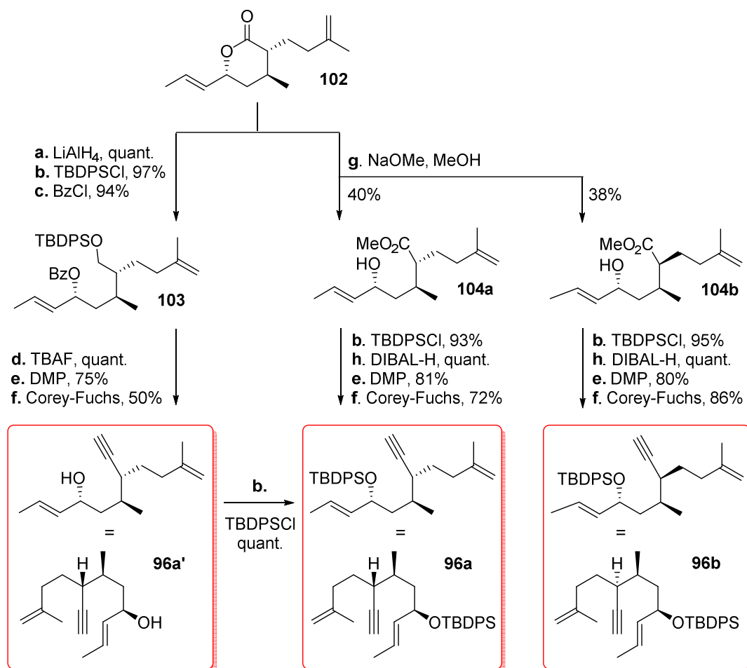
Schéma 15. Synthèse du substrat de cyclisation 96 . a. LiAlH 4 , Et 2 O, 0 °C, 1 h, quant. ; b. TBDPSCI, imidazole, CH 2 Cl 2 , t.a., 12 h, 102-II 97%, 96a quant, 104a-I 93%, 104b-I 95% ; c. BzCl, pyridine, CH 2 Cl 2 , t.a., 3 h, 94% ; d. TBAF, THF, t.a., 12 h, quant. ; e. DMP, CH 2 Cl 2 , t.a., 4-5 h, 103-II 75%, 104a-III 81%, 104b-III 80% ; f. PPh 3 , CBr 4 , CH 2 Cl 2 , 0 °C, 30 min ; n -BuLi, THF, -78 °C, 30 min, 96a' 50%, 96a 72%, 96b 86% (2 étapes) ; g. NaOMe, MeOH, t.a., 12 h, 104a 40%, 104b , 38% ; h. DIBAL-H, toluène, -78 °C, 2 h, 104a-II quant, 104b-II quant. Bz = benzoyl ; DIBAL-H = hydrure de diisobutylaluminium ; DMP = périodine de Dess-Martin ; TBAF = fluorure de tétra- n -butylammonium ; TBDPS = tert -butyldiphénysilyle.
