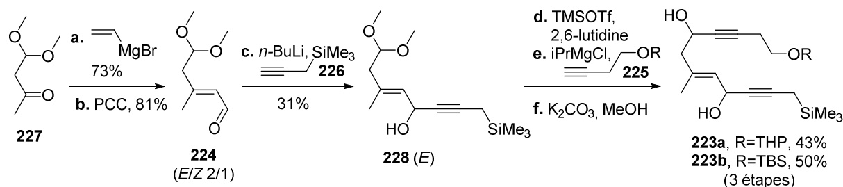
Schéma 45. Synthèse de l'intermédiaire 223 . a. Bromure de vinylmagnésium, THF, -78 °C, 2 h, 73% ; b. PCC, CH 2 Cl 2 , t.a., 48 h, 81% ; c. Alcyne 226 , n -BuLi, THF, -78 °C, 1 h, 31% ; d. TMSOTf, 2,6-lutidine, CH 2 Cl 2 , 0 °C, 1 h, puis H 2 O, 0 °C, 15 min ; e. Alcyne 225 , i PrMgCl, THF, -78 °C, 1 h ; f. K 2 CO 3 , MeOH, t.a., 30 min, 223a 43%, 223b 50% (3 étapes). n -Bu = n -butyle ; i Pr = isopropyle ; PCC = chlorochromate de pyridinium ; Tf = triflyle ; TMS = triméthylsilyl.
