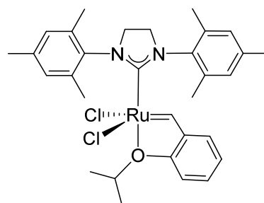
catalyseur de Hoveyda-Grubbs II
