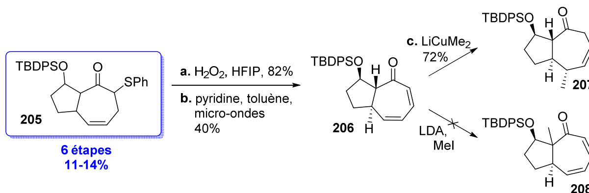
Schéma 40. Fonctionnalisation du noyau hydroazulène 205 . a. \text{H}_2\text{O}_2 , HFIP, t.a., 30 min, 82% ; b. Pyridine, toluène, micro-ondes, 100 °C, 10 min, 40% ; c. MeLi, CuI, \text{Et}_2\text{O} , 1 h, 0 °C, 72%. HFIP = hexafluoroisopropanol ; LDA = diisopropylamide de lithium ; TBDPS = tert -butyldiphénylsilyle.
