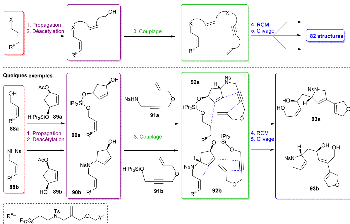
Schéma 9. Synthèse de 82 structures différentes à travers une cascade de métathèses cyclisantes. [53] iPr = isopropyle ; Ns = nosyle ; Ts = tosyle.
