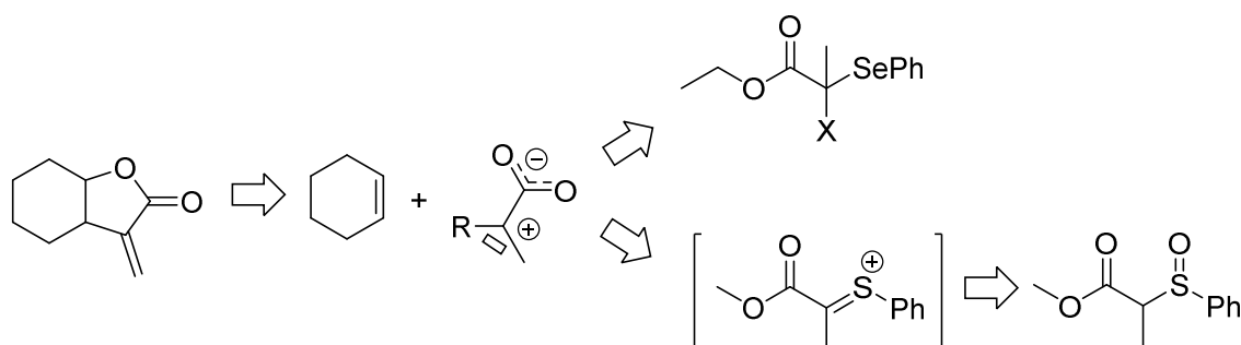
Schéma 27. Addition de dérivés acétylés sur des alcènes pour accéder aux \alpha -méthylène- \gamma -butyrolactones.
