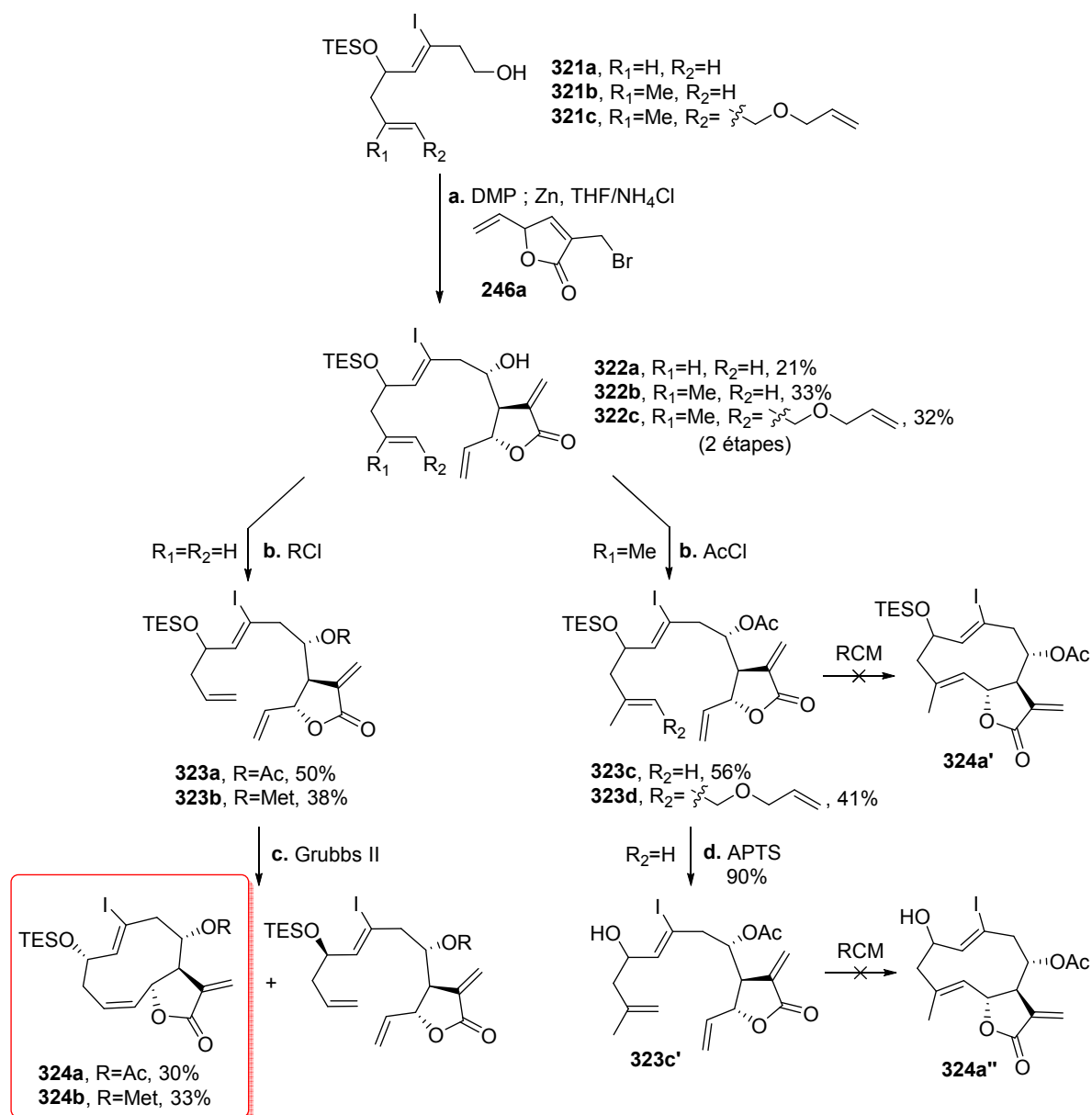
Schéma 69. Vers la métathèse cyclisante. a. DMP, Et_2O , t.a., 1 h ; Zn, THF/ NH_4Cl (2/1), t.a., 20 min, 322a 21%, 322b 33%, 322c 32% (2 étapes) ; b. AcCl, pyridine ou MetCl, Et_3N , CH_2Cl_2 , t.a., 1 h, 323a , 50%, 323b 38%, 323c 56%, 323d 41% ; c. Grubbs II, CH_2Cl_2 , reflux, 12 h, 324a 30%, 324b 33% ; d. APTS- H_2O , THF/ H_2O (5/1), t.a., 2 h, 90%. APTS = acide para -toluènesulfonique ; DMP = périodine de Dess-Martin ; Met = méthacryloyle.
