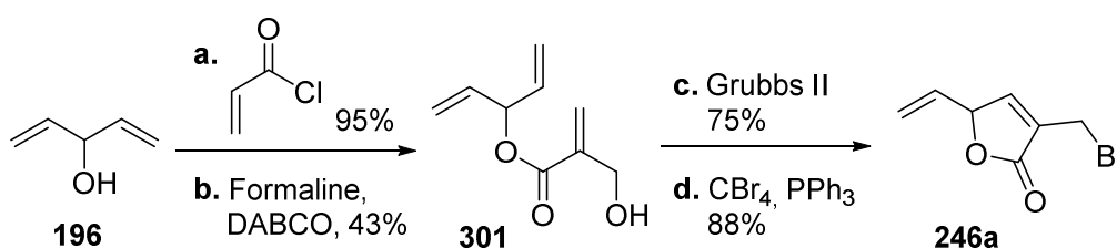
Schéma 62. Deuxième synthèse de la bromolactone 246a . a. Chlorure d'acryloyle, Et 3 N, CH 2 Cl 2 , 0 °C, 1 h, 95% ; b. Formaline, DABCO, H 2 O/1,4-dioxane (1/1), t.a., 48 h, 43% ; c. Grubbs II, CH 2 Cl 2 , reflux, 2 h, 75% ; d. CBr 4 , PPh 3 , CH 2 Cl 2 , 0 °C, 1 h, 88%. DABCO = 1,4-diazabicyclo[2.2.2]octane.
