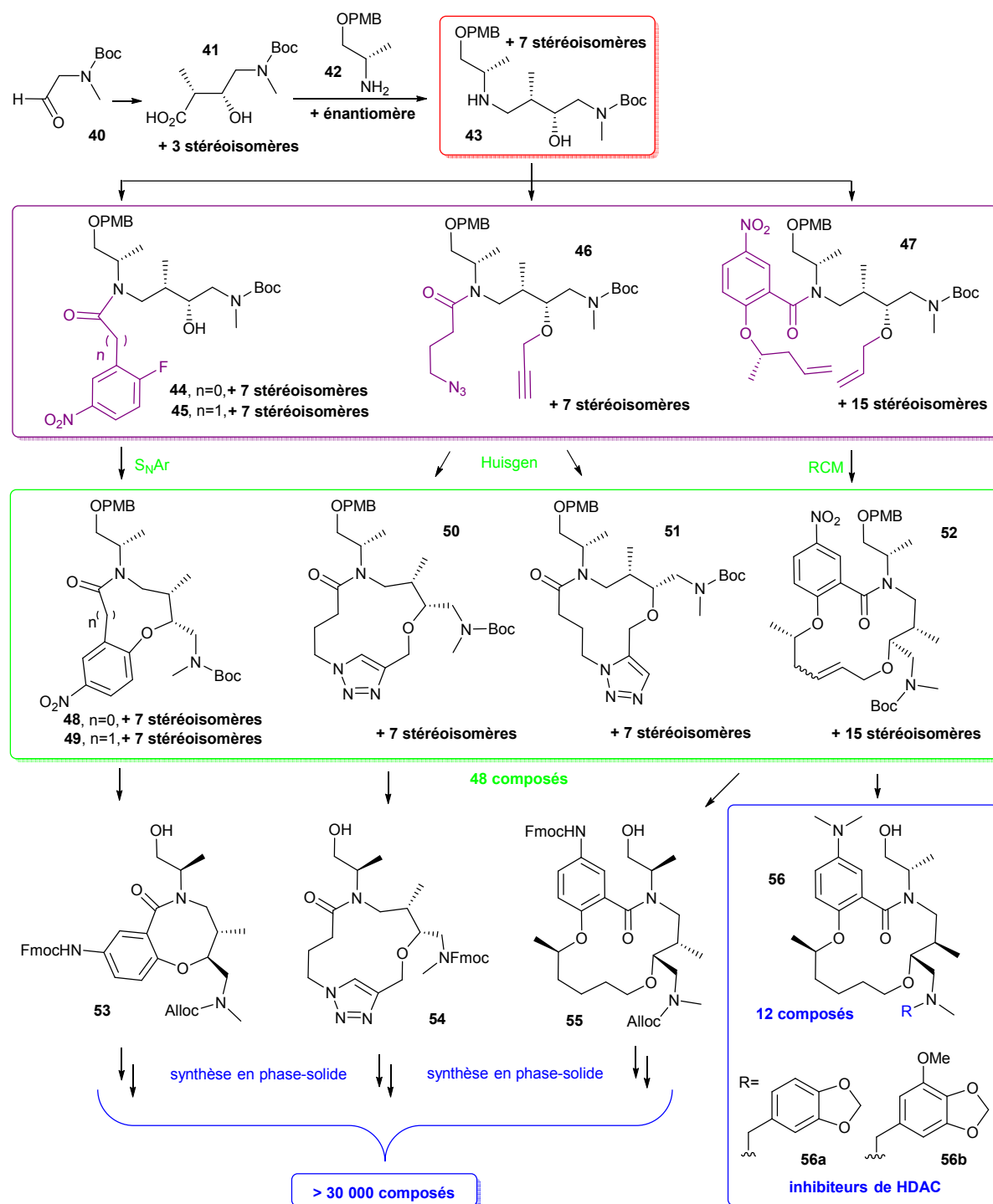
Schéma 6. Synthèse divergente de divers macrocycles utilisant la stratégie build-couple-pair menant à la découverte de nouveaux inhibiteurs de la HDAC. [42] Alloc = allyloxycarbonyl ; Boc = tert -butoxycarbonyl ; Fmoc = 9-fluorénylméthoxycarbonyl ; HDAC = histone déacétylase ; PMB = para -méthoxybenzyle.
