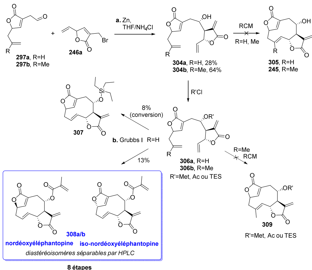
Schéma 64. Synthèse des analogues déméthylés de la déoxyéléphantopine et de l'isodéoxyéléphantopine. a. Zn, THF/NH 4 Cl (2/1), t.a., 20 min, 304a 28%, 304b 64% ; b. Grubbs I, CH 2 Cl 2 , reflux, 12 h, 307 8% conversion, 308 13% (optimisation effectuée par Dr. Roman Lagoutte – Post-doctorant). Met = méthacryloyle ; TES = triéthylsilyle.
