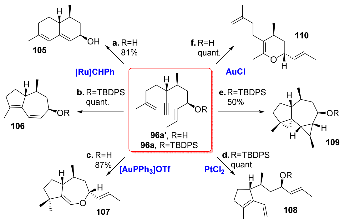
Schéma 16. Synthèse divergente vers diverses structures polycycliques. a. Grubbs II, toluène, reflux, 12 h, 81% ; b. Grubbs II, toluène, reflux, 12 h, quant. ; c. [AuPPh_3]OTf , CH_2Cl_2 , t.a., 20 min, 87% ; d. PtCl_2 , toluène, 50 °C, 2 h, quant. ; e. AuCl , CH_2Cl_2 , t.a., 20 min, 50% ; f. AuCl , CH_2Cl_2 , t.a., 20 min, quant. Tf = triflyle ; TBDPS = tert -butyldiphénylsilyle.
