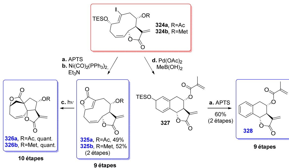
Schéma 70. Synthèse d'analogues à partir du cycle 324 . a. APTS- \text{H}_2\text{O} , \text{THF}/\text{H}_2\text{O} (5/1), t.a., 2 h, 328 60% (2 étapes) ; b. \text{Ni}(\text{CO})_2(\text{PPh}_3)_2 , \text{Et}_3\text{N} , toluène, reflux, 15 min, 325a 49%, 325b 52% (2 étapes) ; c. Lampe U.V. (254 nm, 4W), \text{CD}_3\text{CN} , t.a., 2-7 jours, 326a quant, 326b quant. d. \text{Pd}(\text{OAc})_2 , \text{MeB}(\text{OH})_2 , \text{K}_3\text{PO}_4\text{-H}_2\text{O} , dppb, toluène, 60 °C, 48 h. APTS = acide para -toluènesulfonique ; dppb = 2-dicyclohexylphosphino-2',6'-diméthoxybiphényle ; Met = méthacryloyle ; U.V. = rayonnement ultraviolet.
