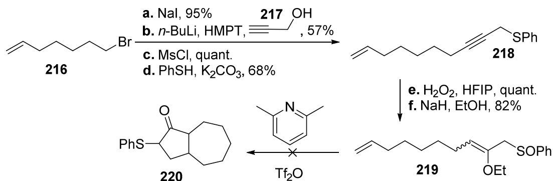
Schéma 43. Tentative de cycloaddition [3+2] pour mener au noyau hydroazulène. a. NaI, Cu, acétone, reflux, 2 h, 95% ; b. Alcyne 217 , n -BuLi, HMPT, t.a., 2 h, 57% ; c. MsCl, Et 3 N, CH 2 Cl 2 , t.a., 2 h, quant. ; d. PhSH, K 2 CO 3 , acétone, t.a., 12 h, 68% ; e. H 2 O 2 , HFIP, t.a., 30 min, quant. ; f. NaH, THF/EtOH, t.a., 30 min, 82%. n -Bu = n -butyle ; HFIP = hexafluoroisopropanol ; HMPT = hexaméthylphosphotriamide ; Ms = mésyle.
