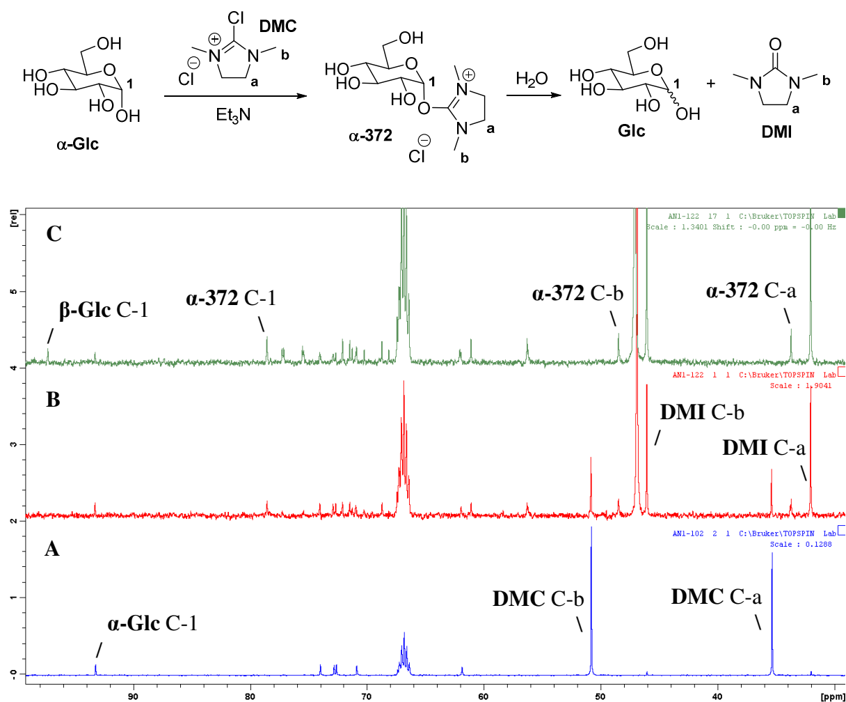
Figure 22. A. Spectre RMN ^{13}\text{C} d'un mélange de \alpha\text{-D-Glucose} (1,0 équiv) et DMC (2,0 équiv) dans \text{D}_2\text{O}/1,4\text{-dioxane-}d_8 (1/1) à -10^\circ\text{C} ; B. Spectre RMN ^{13}\text{C} enregistré 2 minutes après l'ajout de triéthylamine (6,0 équiv) ; C. Spectre RMN ^{13}\text{C} enregistré 30 minutes après B. DMC = chlorure de 2-chloro-1,3-diméthylimidazolinium ; DMI = 1,3-diméthyl-2-imidazolidinone ; Glc = glucose.
