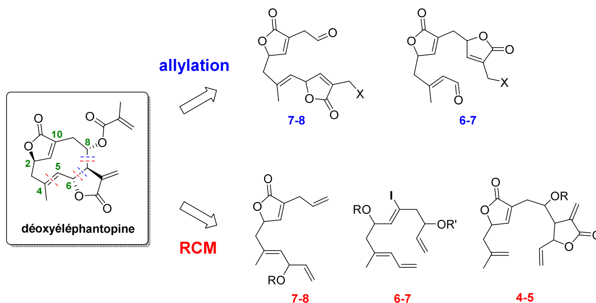
Figure 16. Structure de la déoxyéléphantopine et les deux rétrosynthèses étudiées. Les paires de numéros indiquent les atomes de carbone entre lesquelles s'effectue la déconnexion.
