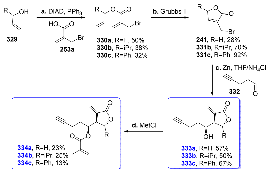
Schéma 71. Synthèse de la première bibliothèque d'analogues. a. Acide (2-bromométhyl)acrylique 253a , DIAD, PPh 3 , Et 2 O, t.a., 12 h, 330a 50%, 330b 38%, 330c 32% ; b. Grubbs II, CH 2 Cl 2 , reflux, 1-2 h, 241 28%, 331b 70%, 331c 92% ; c. Zn, THF/NH 4 Cl (2/1), t.a., 20 min, 333a 57%, 333b 50%, 333c 67% ; d. MetCl, Et 3 N, CH 2 Cl 2 , t.a., 1 h, 334a 23%, 334b 25%, 334c 13%. DIAD = azodicarboxylate de diisopropyle ; iPr = isopropyle ; Met = méthacryloyle.
