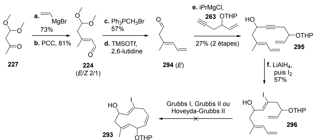
Schéma 59. Deuxième tentative de cyclisation par métathèse. a. Bromure de vinylmagnésium, THF, -78 °C, 2 h, 73% ; b. PCC, CH 2 Cl 2 , t.a., 48 h, 81% ; c. Ph 3 PCH 3 Br, n -BuLi, THF, reflux, 2 h, 57% ; d. TMSOTf, 2,6-lutidine, CH 2 Cl 2 , 0 °C, 1 h, puis H 2 O, 0 °C, 15 min ; e. Alcyne 263 , iPrMgCl, THF, -78°C, 1 h, 27% (2 étapes) ; f. LiAlH 4 , THF, reflux, 3 h, puis EtOAc, 0 °C, 15 min, puis I 2 , 0 °C, 1 h, 57%. iPr = isopropyle ; PCC = chlorochromate de pyridinium ; Tf = triflyle ; TMS = triméthylsilyle.
