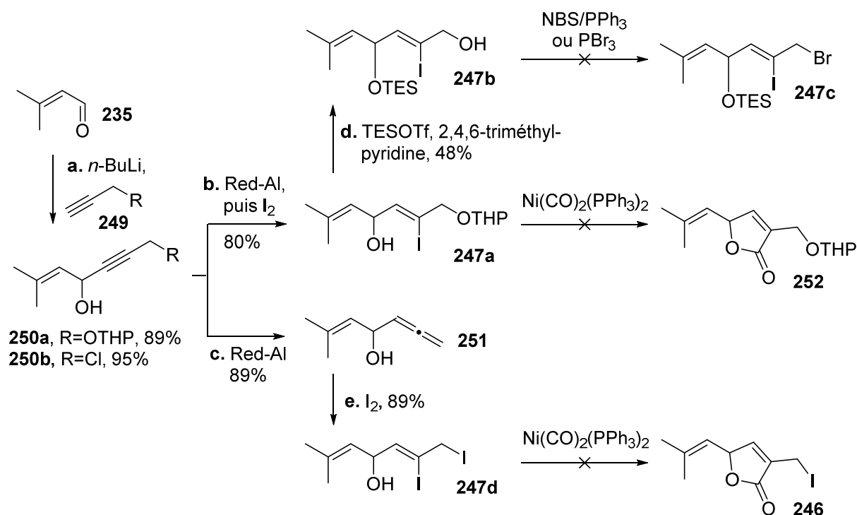
Schéma 50. Tentatives de synthèse de la bromolactone fonctionnalisée 246 . a. Alcyne 249 , n\text{-BuLi} , THF, -78\text{ }^\circ\text{C} , 1 h, 250a 89%, 250b 95% ; b. Red-Al ® , THF, 0\text{ }^\circ\text{C} , 15 min, puis EtOAc, 0\text{ }^\circ\text{C} , 15 min, puis \text{I}_2 , 0\text{ }^\circ\text{C} , 1 h, 80% ; c. Red-Al ® , THF, 0\text{ }^\circ\text{C} , 10 min, 89% ; d. TESOTf, 2,4,6-triméthylpyridine, \text{CH}_2\text{Cl}_2 , 0\text{ }^\circ\text{C} , 1 h, puis \text{H}_2\text{O} , 0\text{ }^\circ\text{C} , 15 min, 48% ; e. \text{I}_2 , THF, t.a., 2 h, 89%. n\text{-Bu} = n -butyle ; NBS = N -bromosuccinimide ; Red-Al ® = bis(2-méthoxyéthoxy)hydruroaluminate de sodium ; TES = triéthylsilyle ; Tf = triflyle ; THP = tétrahydropyrane.
