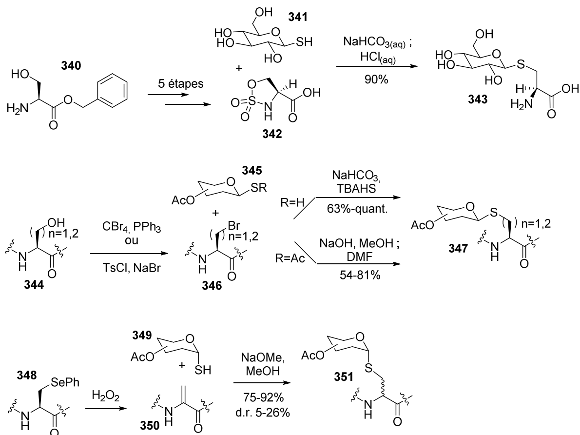
Schéma 74. Quelques exemples de synthèse de S -glycopeptides par addition conjuguée ou substitution de 1-thioglycol. TBAHS = hydrogénosulfate de tétra- n -butylammonium ; Ts = tosyle.
