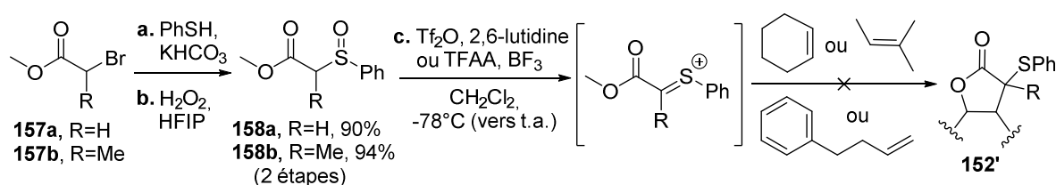
Schéma 29. Tentatives de cyclisation à partir de dérivés soufrés vers les \gamma -butyrolactones. a. PhSH, \text{KHCO}_3 , DMF, t.a., 12 h, 157a-I 90%, 157b-I 97% ; b. \text{H}_2\text{O}_2 , HFIP, t.a., 30 min, 158a quant, 158b 97%. HFIP = hexafluoroisopropanol ; Tf = triflyle ; TFAA = anhydride trifluoroacétique.
