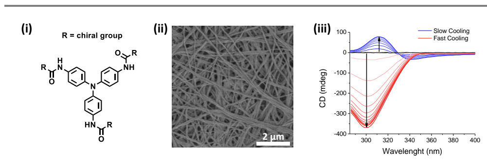
Figure A | (i) Structure de TATAs décorées avec des substituants alkyles ; (ii) Image de microscopie électronique à balayage de l'auto-assemblage de TATA dans le toluène; (iii) Spectres de dichroïsme circulaire obtenus pour une solution de TATA à 0,5 mM dans le toluène pour différents régimes de refroidissement: refroidissement lent (1 K/min, lignes bleues); refroidissement rapide (10 K/min, lignes rouges).
