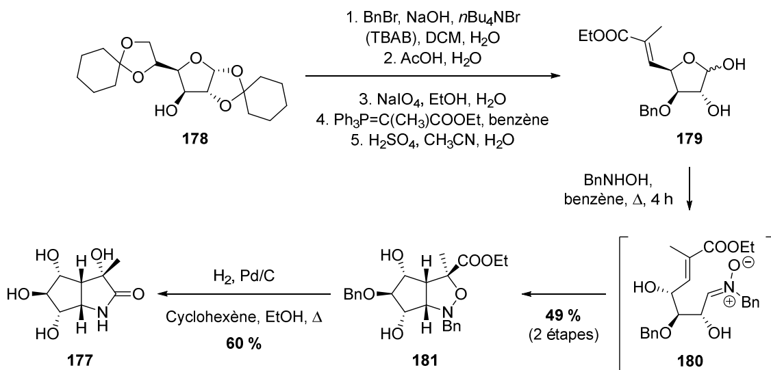
Schéma 27 – Synthèse du 1-aza-2-oxo-3,4,5,6-tétrahydrobicyclo[3.3.0]octane 177
