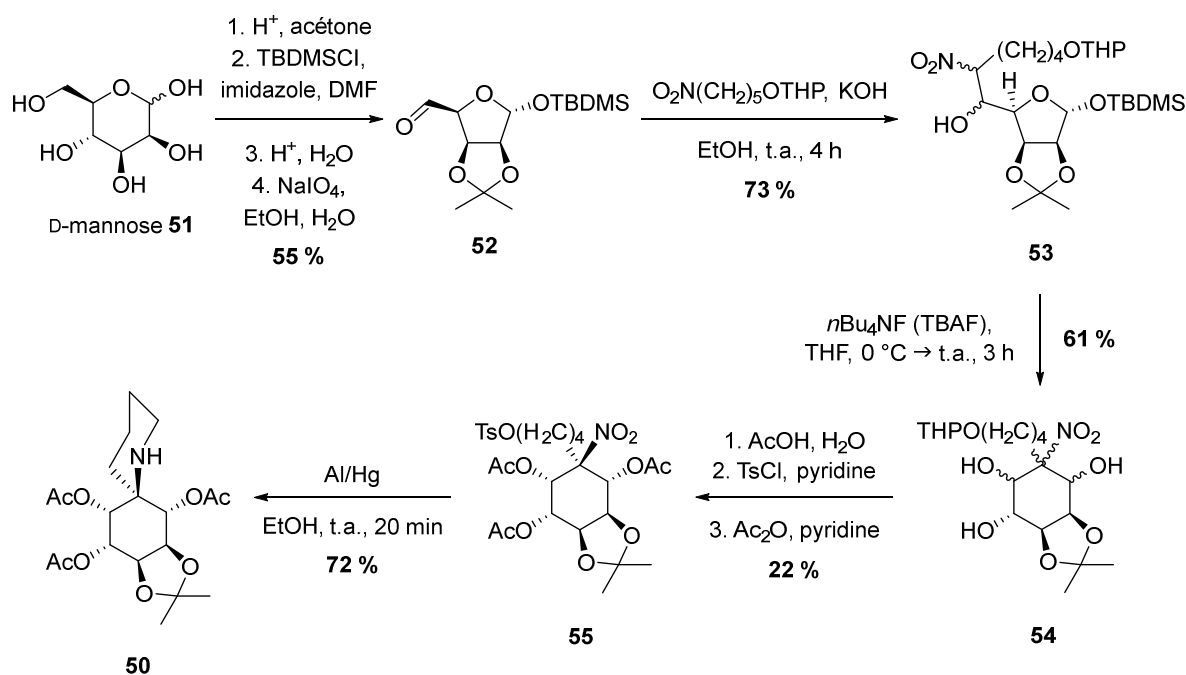
Schéma 7 – Synthèse du 1-azaspiro[5.5]undécane pentahydroxylé 50
