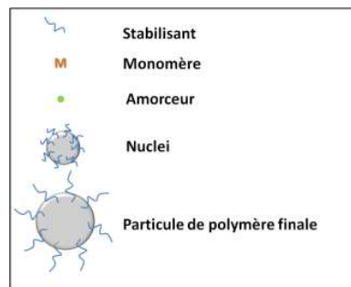
Figure S1. 2: Schéma de la polymérisation en dispersion à l'état initial (1), à la nucléation (2), à la terminaison (3)
