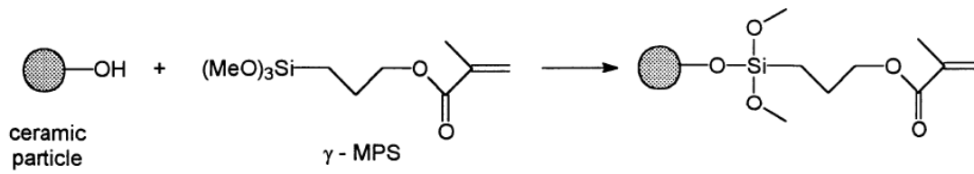
Figure S1.3: Greffage d'un groupement (triméthoxysilyl)propyl méthacrylate en surface d'une particule de céramique[11]
